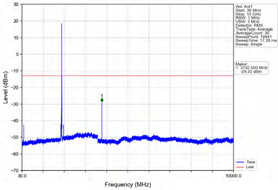
Band25_20MHz_QPSK_HCH_1905MHz_RB_1_0_NTNV
