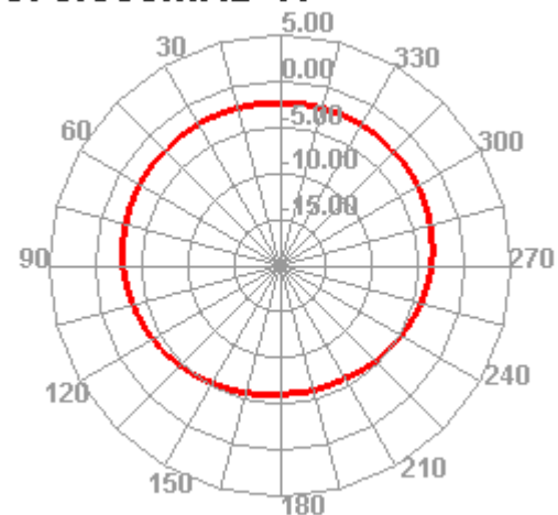
870.000MHz H
