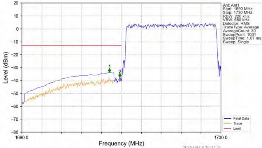
Band66_20MHz_16QAM_LCH_1720MHz_RB_100_0_NTNV
