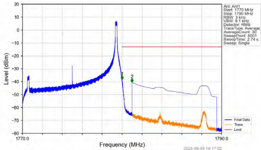
Band66_10MHz_QPSK_HCH_1775MHz_RB_1_49_NTNV
