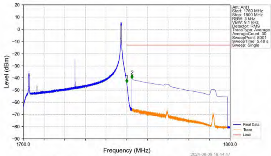
Band66_20MHz_16QAM_HCH_1770MHz_RB_1_99_NTNV
