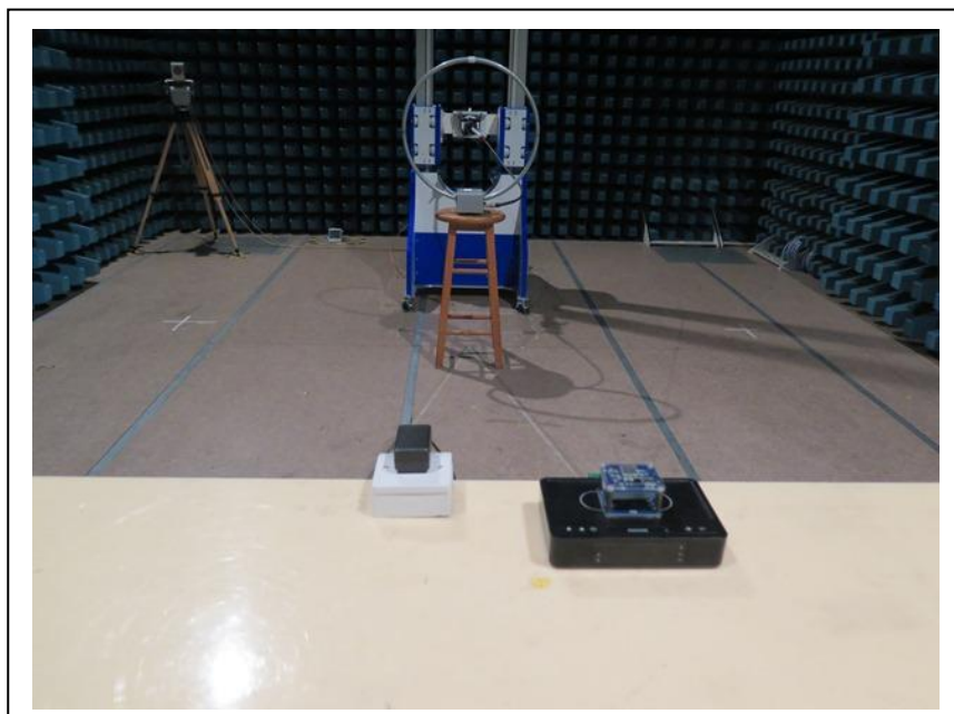
9kHz – 30MHz
