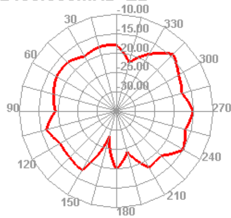
2450.000MHz E2
