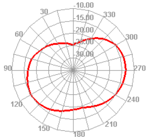
2500.000MHz H
