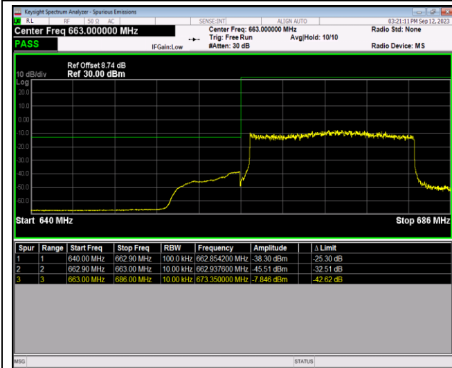
Band71-20MHz-16QAM-133372-1RB#99
