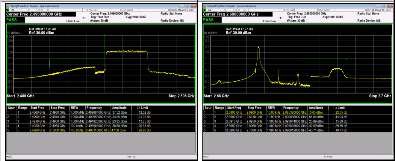
Band41-5MHz-16QAM-41565-1RB#24
