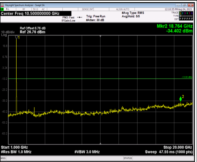
Band25-20MHz-16QAM-26365-1RB#0-Range2:1000~20000MHz
