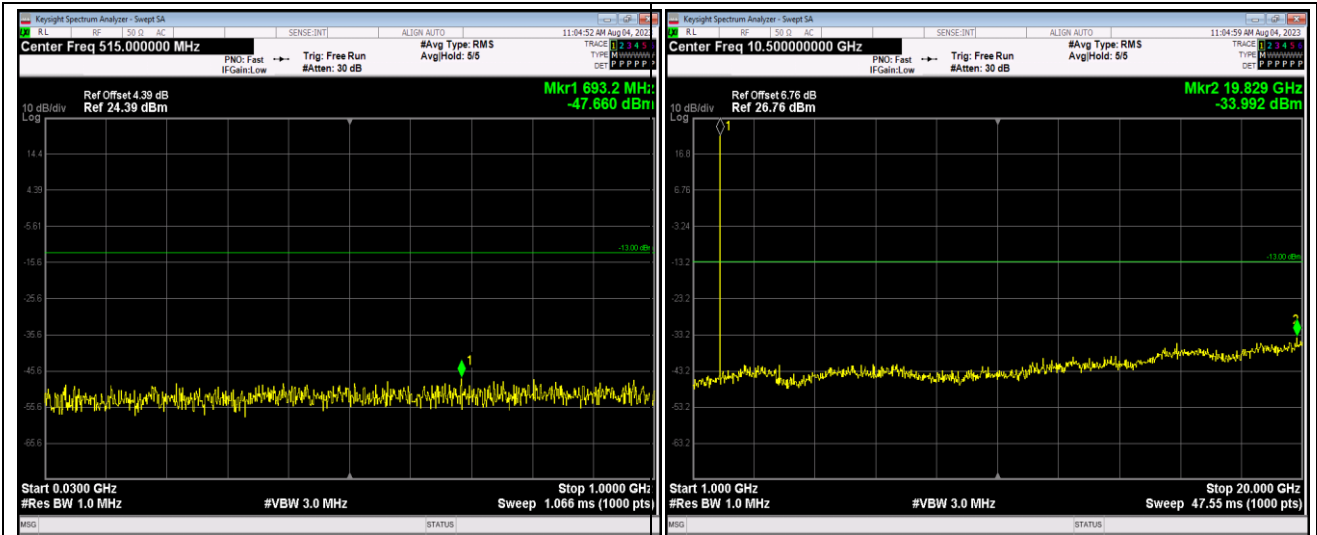
Band25-1.4MHz-64QAM-26365-1RB#0-Range1:30 ~1000MHz
