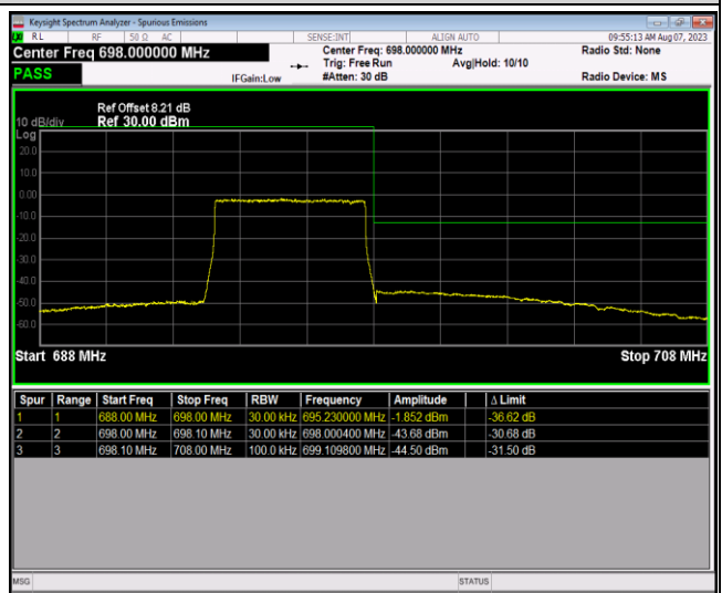
Band71-20MHz-QPSK-133222-1RB#99
