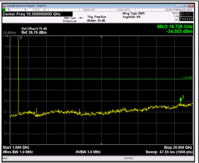
Band4-1.4MHz-QPSK-19957-1RB#0-Range2:1000~20000MHz
