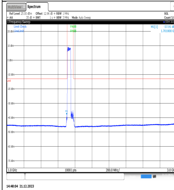
NTVN_N66_PC3_15_40_L_TID1_NS_01_1000_3_000_#1
