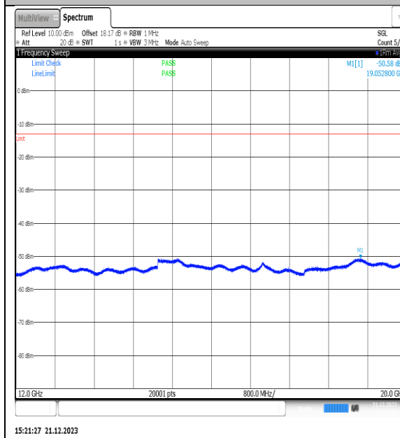
NTVN_N66_PC3_15_40_L_TID12_NS_01_12000_20000_#1
