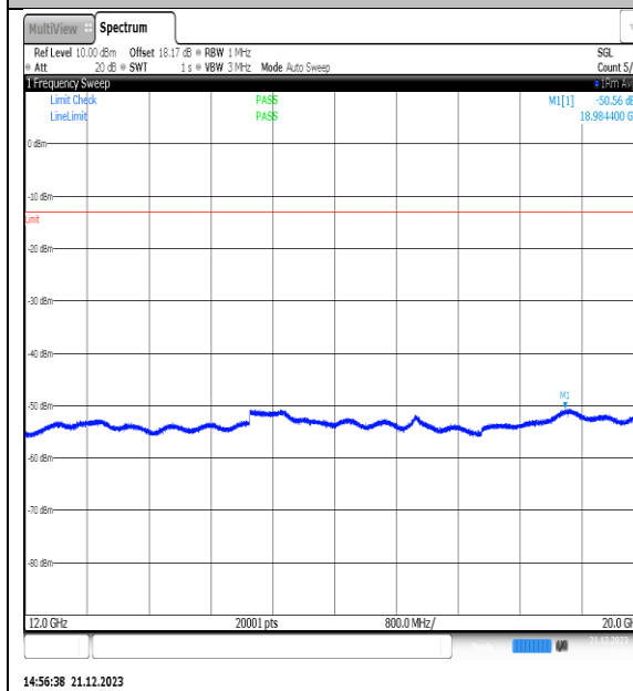
NTVN_N66_PC3_15_40_L_TID4_NS_01_12000_20000_#1
