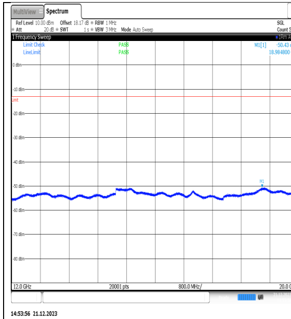
NTVN_N66_PC3_15_40_L_TID3_NS_01_12000_20000_#1
