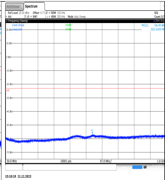
NTVN_N66_PC3_15_40_L_TID9_NS_01_30_100_0_#1
