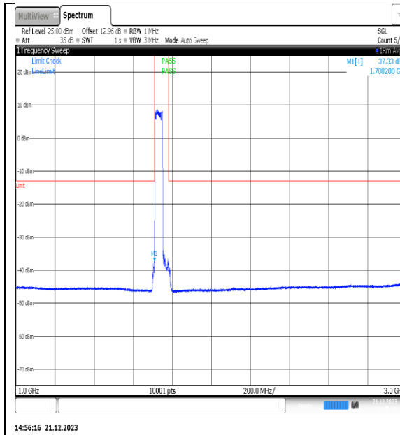
NTVN_N66_PC3_15_40_L_TID4_NS_01_1000_3000_#1
