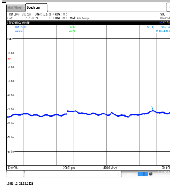
NTVN_N66_PC3_15_40_L_TID6_NS_01_12000_20000_#1
