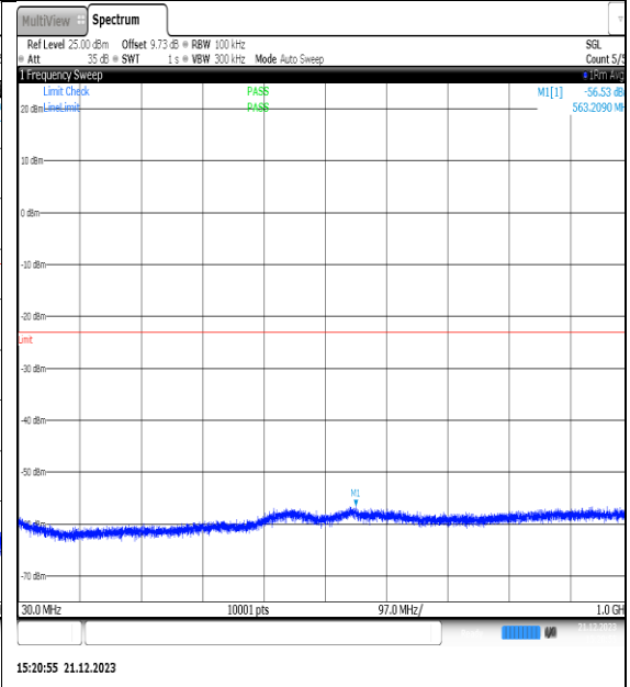
NTNV_N66_PC3_15_40_L_TID12_NS_01_30_100_#1
