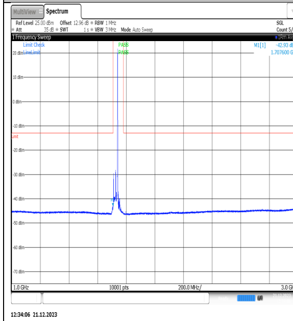
NTVN_N66_PC3_15_30_L_TID12_NS_01_1000_3000_#1
