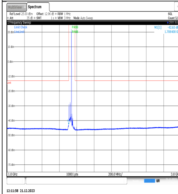
NTVN_N66_PC3_15_30_L_TID6_NS_01_1000_3_000_#1
