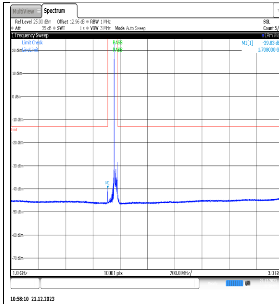
NTVN_N66_PC3_15_25_H_TID2_NS_01_1000_3000_#1
