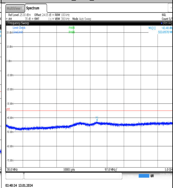
NTVN_N41_PC2_30_100_M_TID3_NS_01_30_1_000_#1
