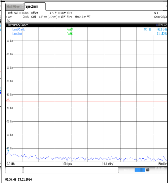
NTVN_N41_PC2_30_100_L_TID5_NS_01_0.009_0.15_#1
