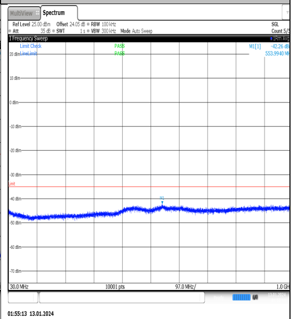
NTNV_N41_PC2_30_100_L_TID4_NS_01_30_100_00_#1
