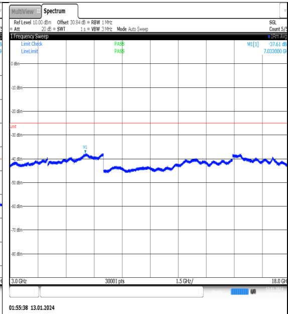
NTVN_N41_PC2_30_100_L_TID4_NS_01_3000_18000_#1
