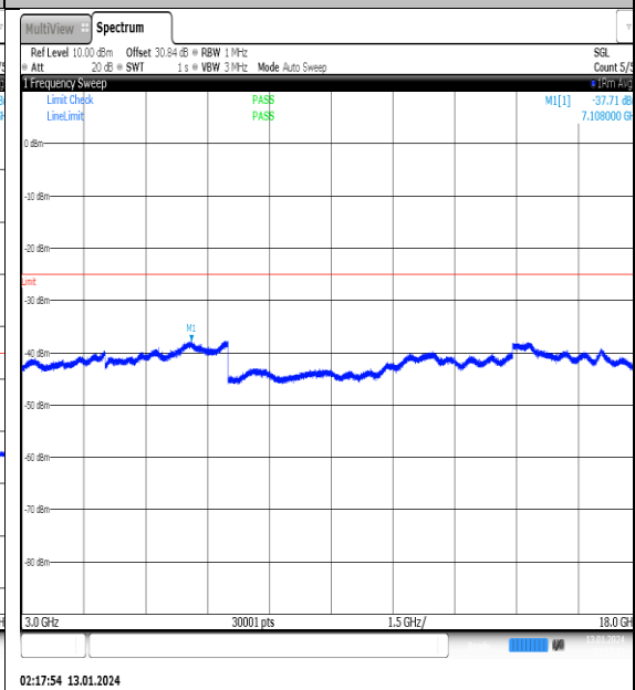
NTVN_N41_PC2_30_100_L_TID11_NS_01_3000_18000_#1
