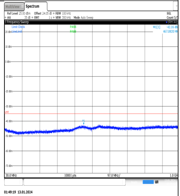
NTNV_N41_PC2_30_100_L_TID2_NS_01_30_100_#1
