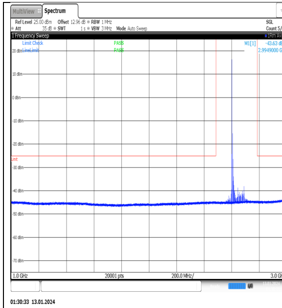
NTVN_N41_PC2_30_90_H_TID11_NS_01_1000_3000_#1
