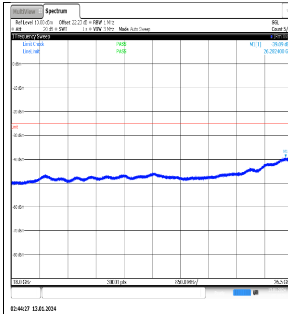
NTVN_N41_PC2_30_100_M_TID4_NS_01_1800_0_26500_#1
