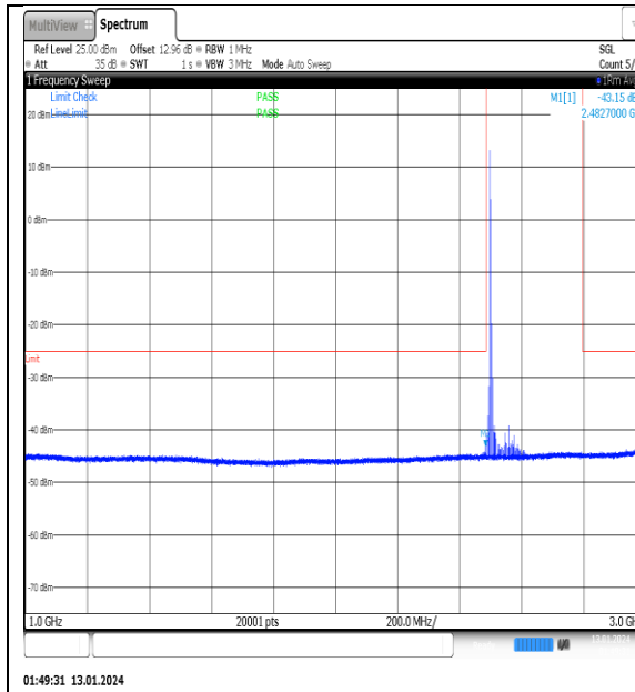
NTNV_N41_PC2_30_100_L_TID2_NS_01_1000_3000_#1
