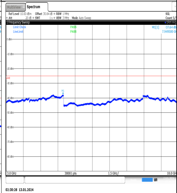
NTVN_N41_PC2_30_100_L_TID15_NS_01_3000_18000_#1
