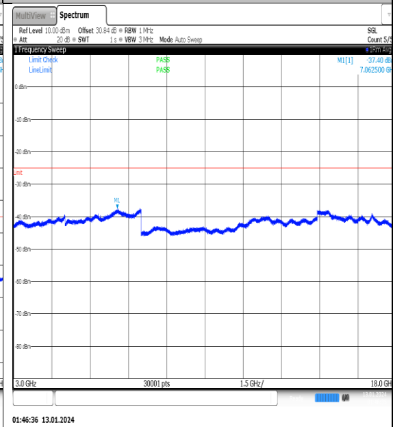
NTVN_N41_PC2_30_100_L_TID1_NS_01_3000_18000_#1
