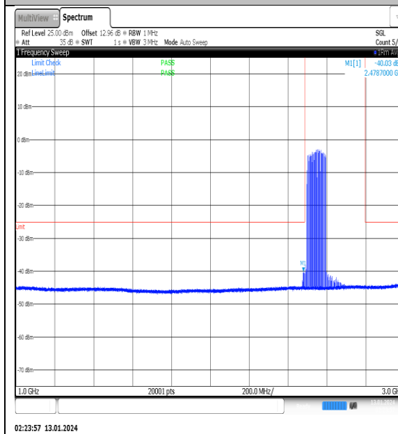
NTVN_N41_PC2_30_100_L_TID13_NS_01_1000_3000_#1
