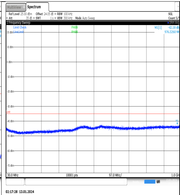
NTVN_N41_PC2_30_100_L_TID11_NS_01_30_1_000_#1
