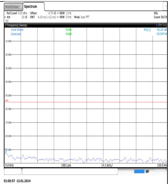
NTVN_N41_PC2_30_100_L_TID6_NS_01_0.009_0.15_#1
