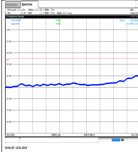
NTNV_N41_PC2_30_100_L_TID6_NS_01_18000_26500_#1
