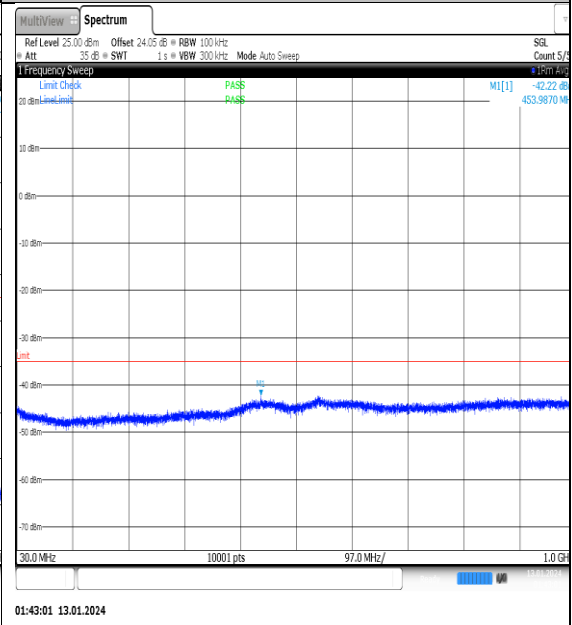
NTVN_N41_PC2_30_90_H_TID15_NS_01_30_1000_#1
