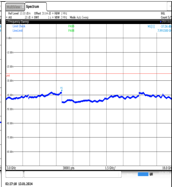
NTNV_N41_PC2_30_100_L_TID14_NS_01_3000_18000_#1
