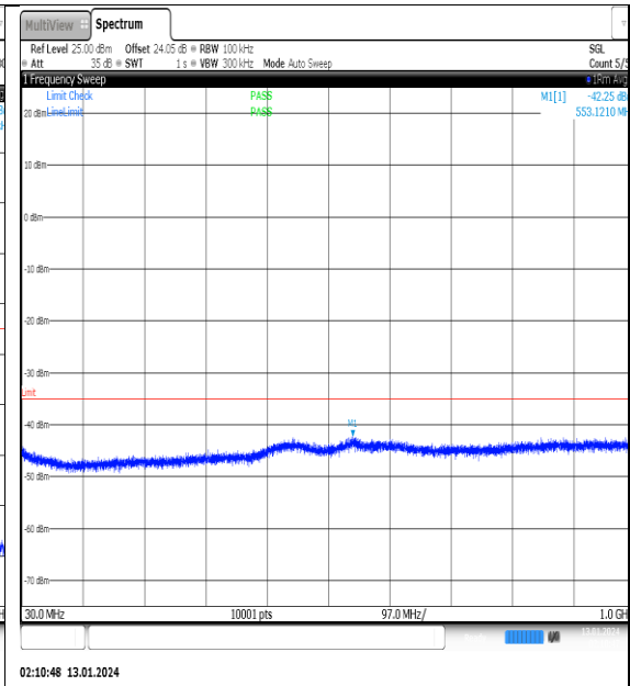
NTVN_N41_PC2_30_100_L_TID9_NS_01_30_1000_#1
