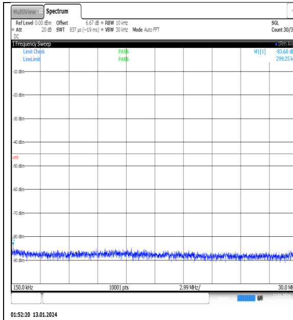
NTVN_N41_PC2_30_100_L_TID3_NS_01_0.15_30_#1
