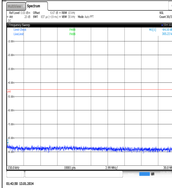
NTVN_N41_PC2_30_90_H_TID15_NS_01_0.15_30_#1
