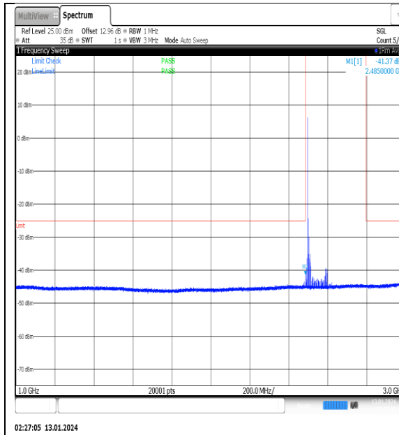
NTNV_N41_PC2_30_100_L_TID14_NS_01_1000_3000_#1
