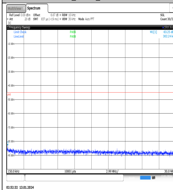
NTVN_N41_PC2_30_100_M_TID7_NS_01_0.15_30_#1
