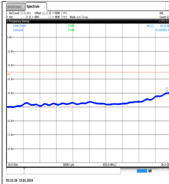
NTVN_N41_PC2_30_100_L_TID9_NS_01_18000_26500_#1
