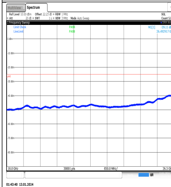
NTVN_N41_PC2_30_90_H_TID15_NS_01_18000_26500_#1
