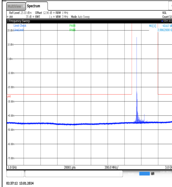
NTNV_N41_PC2_30_100_M_TID2_NS_01_1000_3000_#1
