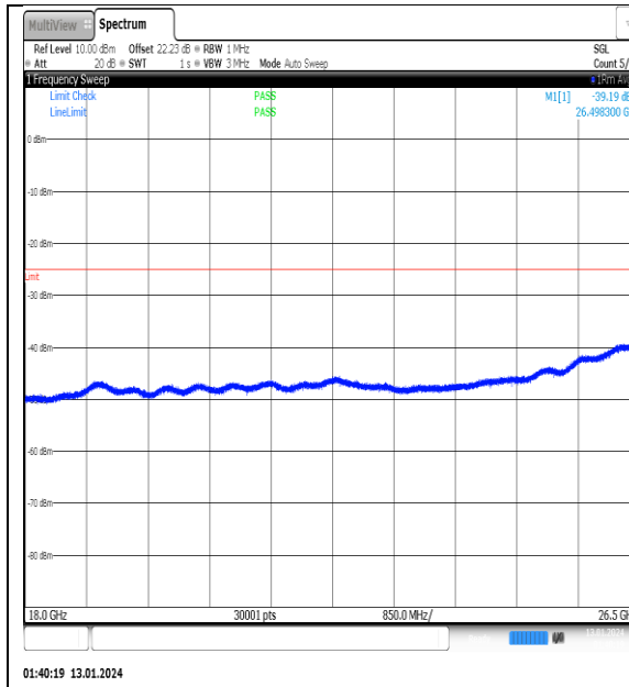
NTVN_N41_PC2_30_90_H_TID14_NS_01_18000_26500_#1
