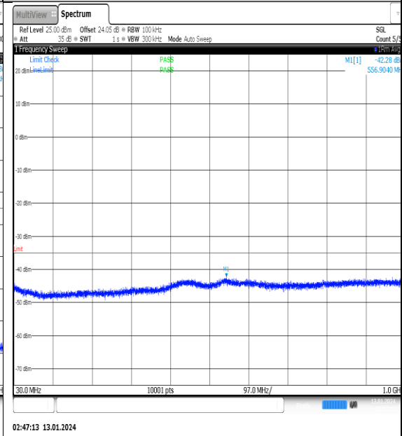
NTVN_N41_PC2_30_100_M_TID5_NS_01_30_1_000_#1
