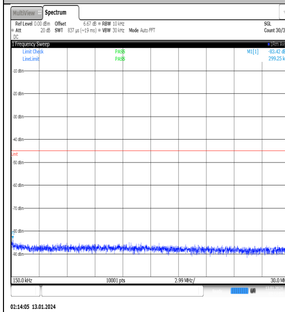
NTVN_N41_PC2_30_100_L_TID10_NS_01_0.15_30_#1
