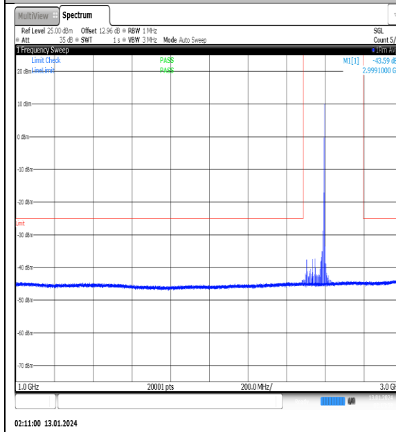
NTVN_N41_PC2_30_100_L_TID9_NS_01_1000_3000_#1
