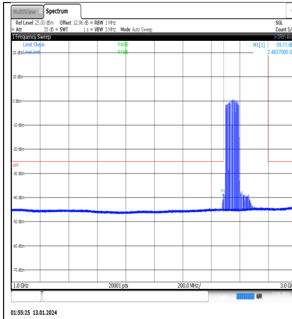
NTVN_N41_PC2_30_100_L_TID4_NS_01_1000_3000_#1
