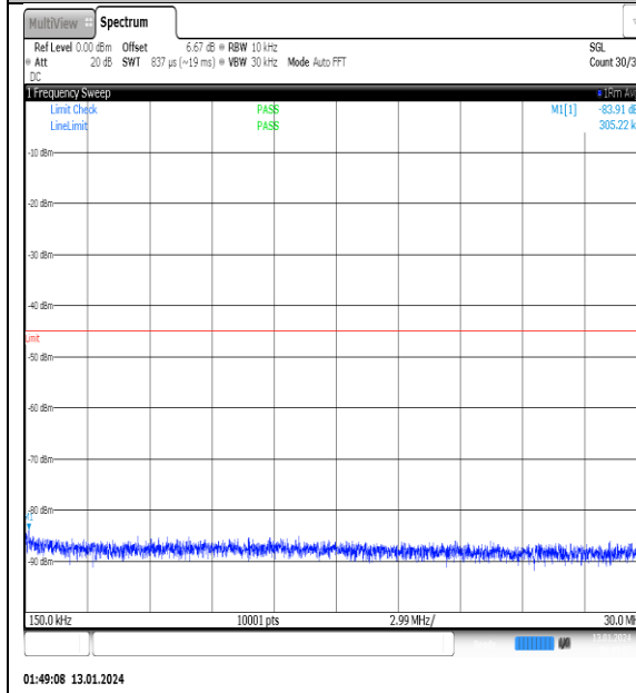
NTNV_N41_PC2_30_100_L_TID2_NS_01_0.15_30_#1
