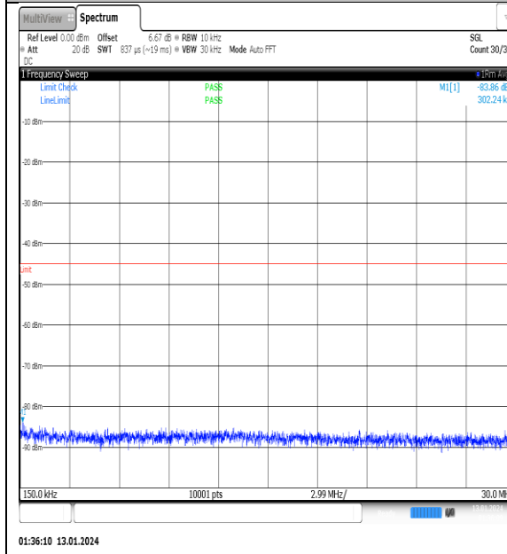
NTVN_N41_PC2_30_90_H_TID13_NS_01_0.15_30_#1
