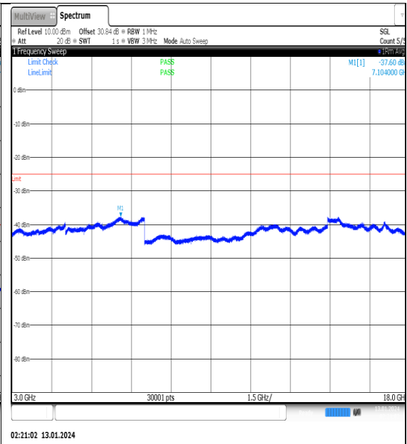
NTVN_N41_PC2_30_100_L_TID12_NS_01_3000_18000_#1
