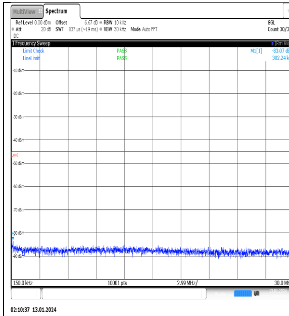
NTVN_N41_PC2_30_100_L_TID9_NS_01_0.15_30_#1
