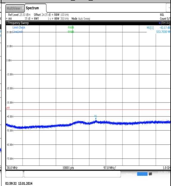
NTVN_N41_PC2_30_100_M_TID9_NS_01_30_1_000_#1
