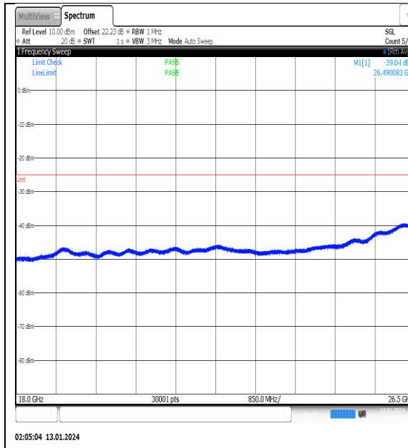
NTNV_N41_PC2_30_100_L_TID7_NS_01_18000_26500_#1
