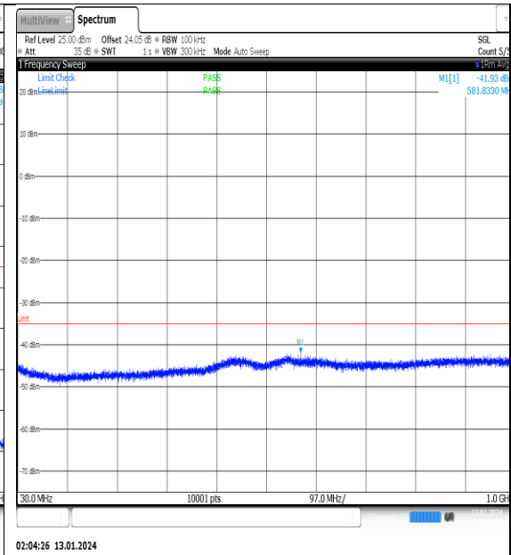
NTVN_N41_PC2_30_100_L_TID7_NS_01_30_1000_#1
