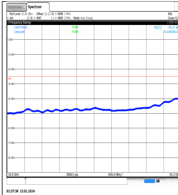
NTVN_N41_PC2_30_100_M_TID2_NS_01_1800 0_26500_#1
