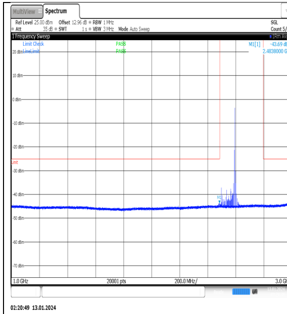
NTVN_N41_PC2_30_100_L_TID12_NS_01_1000_3000_#1
