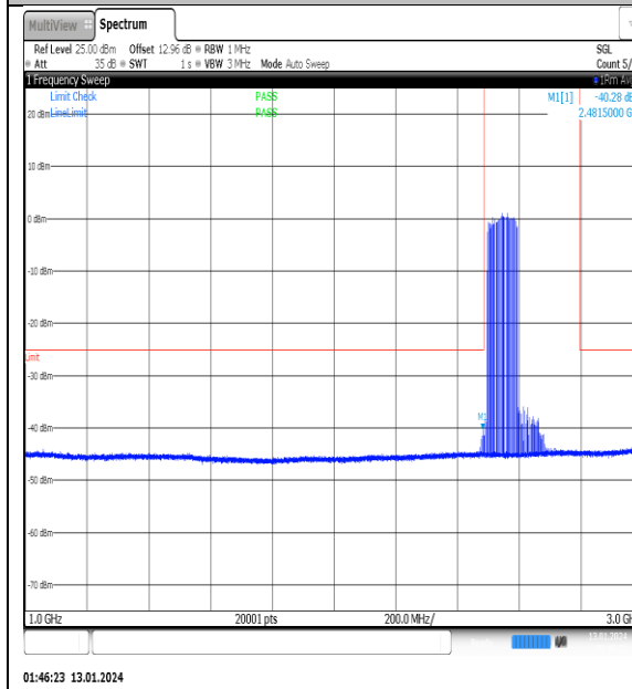
NTVN_N41_PC2_30_100_L_TID1_NS_01_1000_3000_#1
