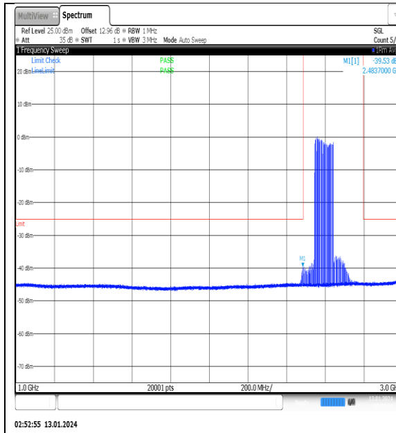
NTNV_N41_PC2_30_100_M_TID7_NS_01_1000_3000_#1
