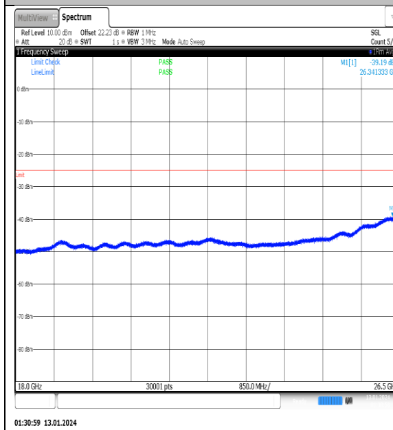
NTVN_N41_PC2_30_90_H_TID11_NS_01_18000_26500_#1
