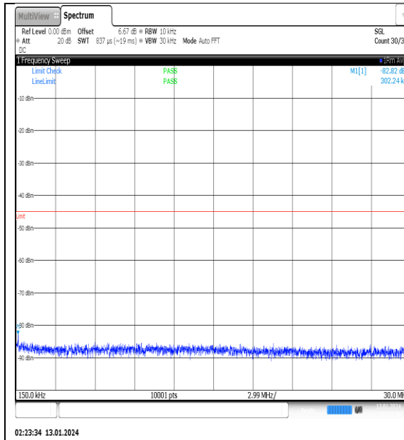
NTVN_N41_PC2_30_100_L_TID13_NS_01_0.15_30_#1
