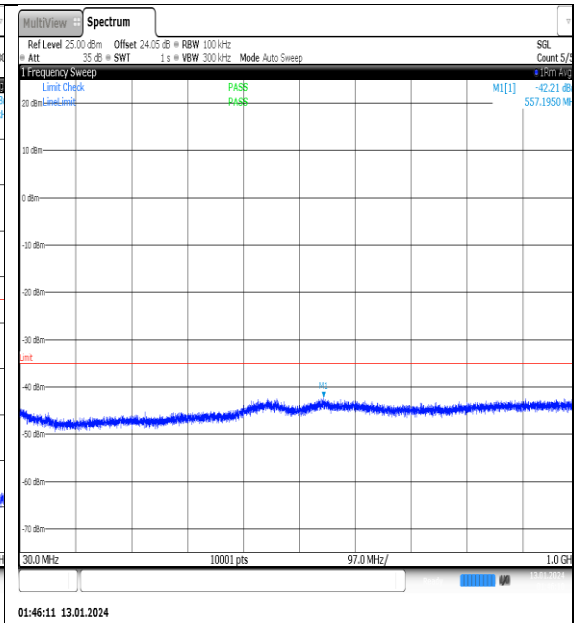
NTVN_N41_PC2_30_100_L_TID1_NS_01_30_1000_#1
