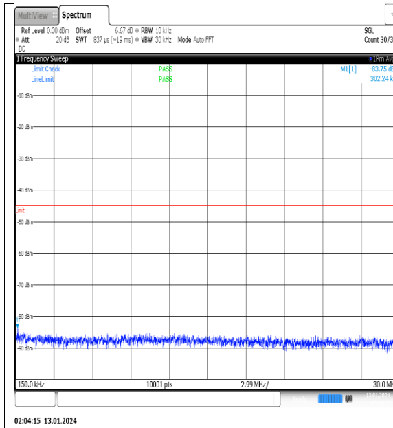
NTVN_N41_PC2_30_100_L_TID7_NS_01_0.15_30_#1
