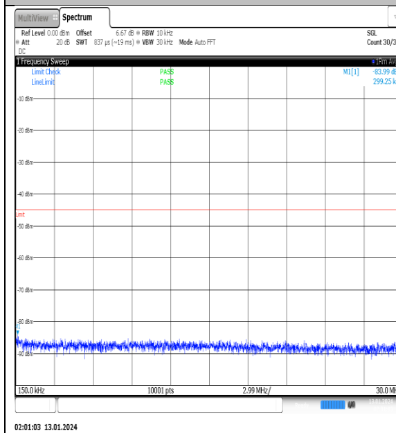
NTVN_N41_PC2_30_100_L_TID6_NS_01_0.15_30_#1
