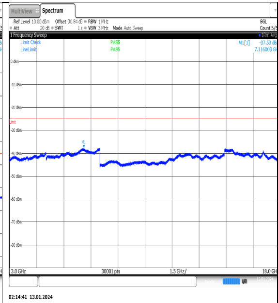
NTNV_N41_PC2_30_100_L_TID10_NS_01_3000_18000_#1
