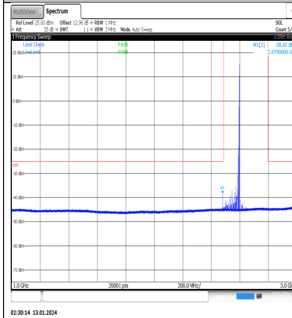
NTVN_N41_PC2_30_100_L_TID15_NS_01_1000_3000_#1
