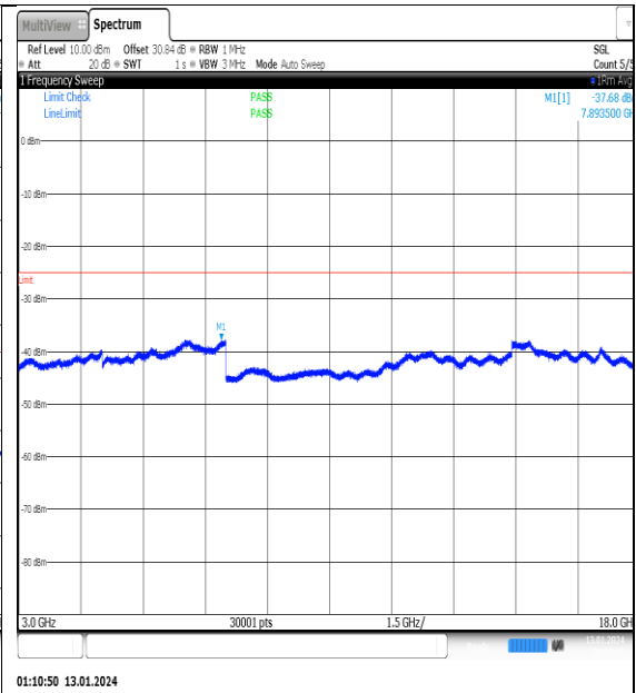
NTVN_N41_PC2_30_90_H_TID5_NS_01_3000_18000_#1
