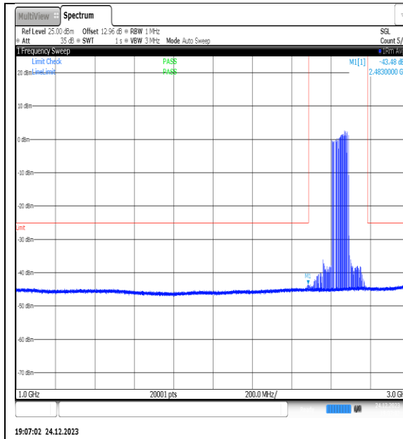
NTVN_N41_PC2_30_90_H_TID1_NS_01_1000_3000_#1
