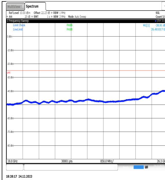
NTVN_N41_PC2_30_90_M_TID3_NS_01_18000_26500_#1
