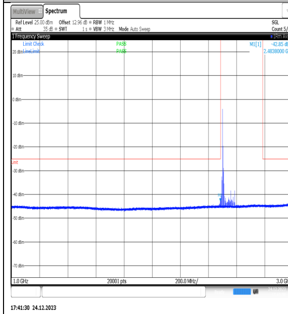
NTVN_N41_PC2_30_90_L_TID14_NS_01_1000_3000_#1
