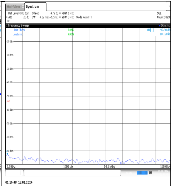
NTVN_N41_PC2_30_90_H_TID7_NS_01_0.009_0.15_#1
