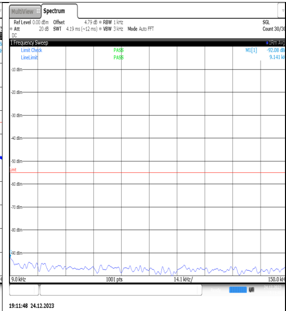
NTVN_N41_PC2_30_90_H_TID3_NS_01_0.009_0.15_#1
