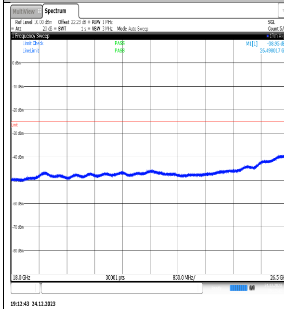
NTVN_N41_PC2_30_90_H_TID3_NS_01_18000_26500_#1
