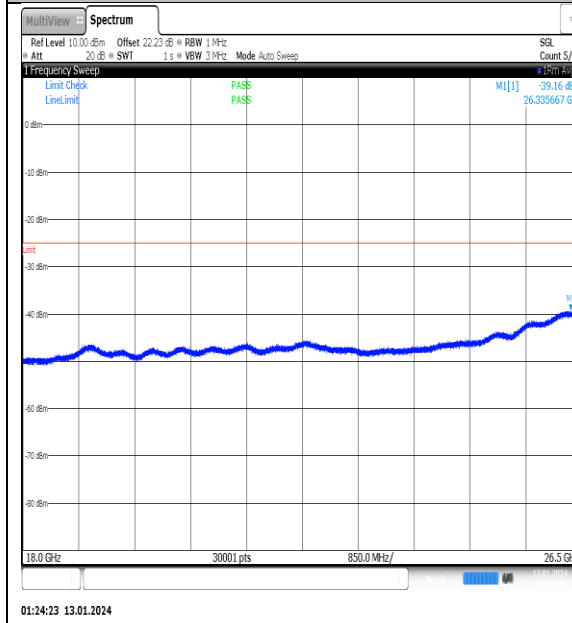
NTVN_N41_PC2_30_90_H_TID9_NS_01_18000_26500_#1
