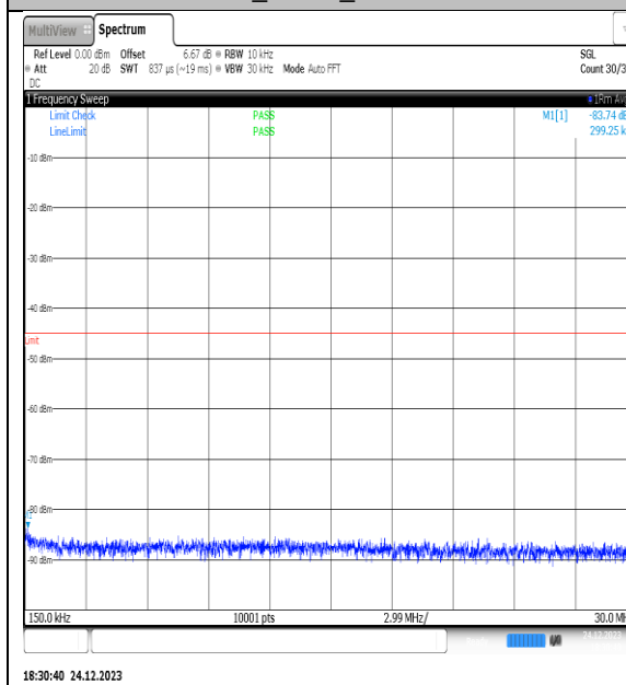
NTVN_N41_PC2_30_90_M_TID4_NS_01_0.15_30_#1
