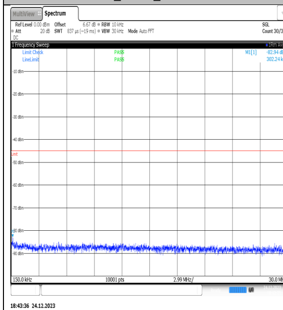
NTVN_N41_PC2_30_90_M_TID8_NS_01_0.15_30_#1
