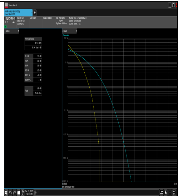
NTNV_N66_PC3_15_5_L_TID1_#1
