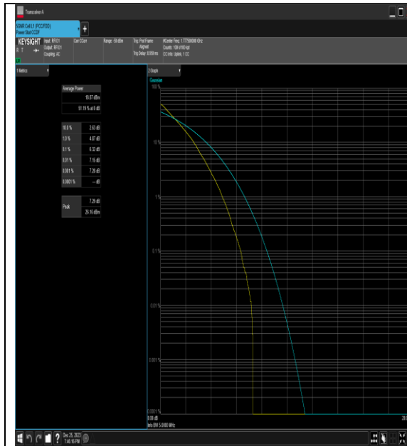
NTNV_N66_PC3_15_5_H_TID2_#1
