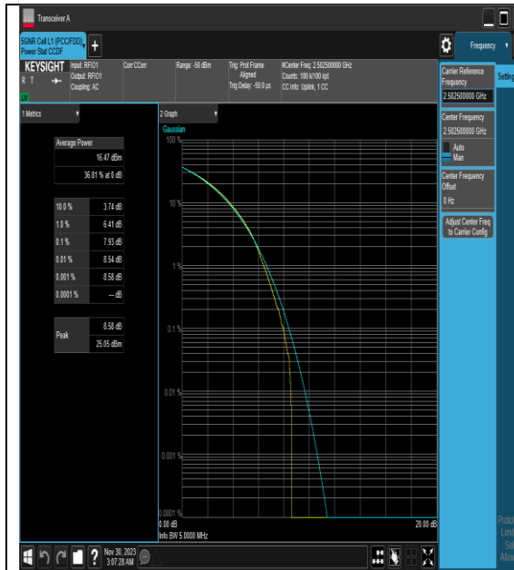
NTNV_N7_PC3_15_5_L_TID8_#1
