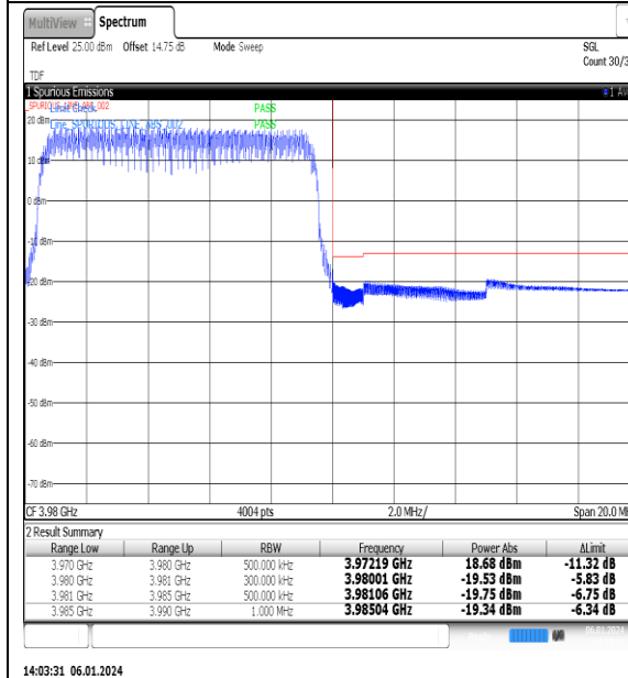
NTNV_N77-3700-3980_PC2_30_10_H_TID7_#1
