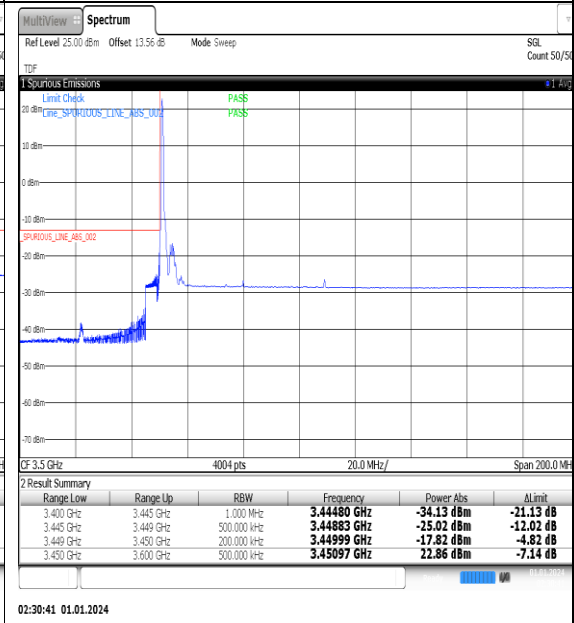
NTNV_N77-3450-3550_PC2_30_60_L_TID2_#1
