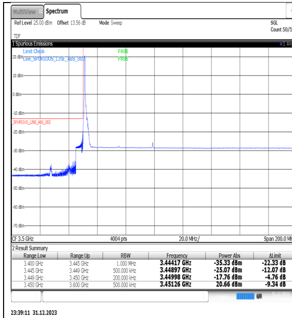
NTNV_N77-3450-3550_PC2_30_50_L_TID5_#1
