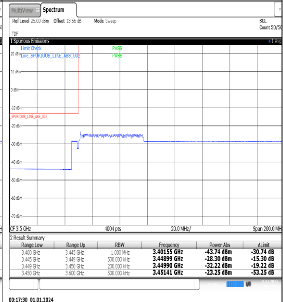
NTNV_N77-3450-3550_PC2_30_50_L_TID10_#1
