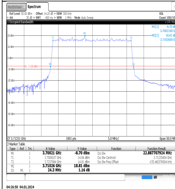
NTNV_N77-3700- 3980_PC2_30_25_L_TID1_Ant1#1
