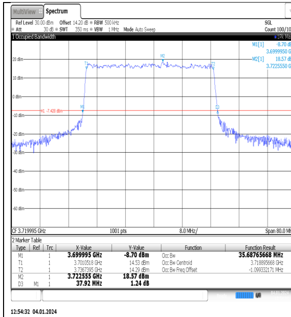
NTNV_N77-3700- 3980_PC2_30_40_L_TID2_Ant1#1
