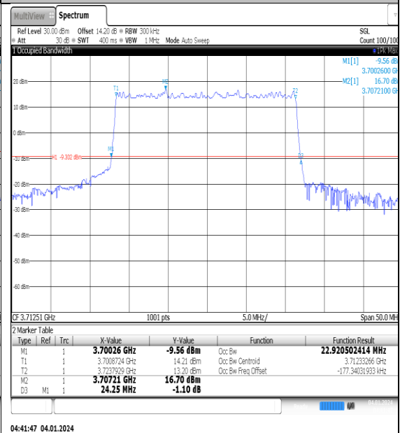
NTNV_N77-3700- 3980_PC2_30_25_L_TID3_Ant1#1
