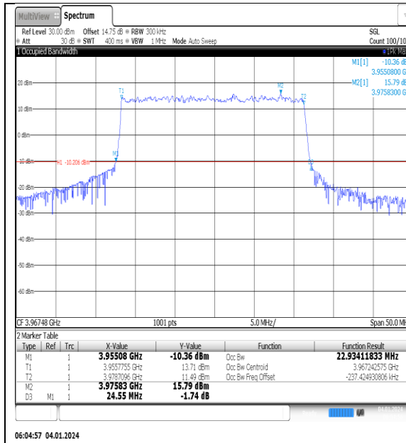
NTNV_N77-3700- 3980_PC2_30_25_H_TID4_Ant1#1
