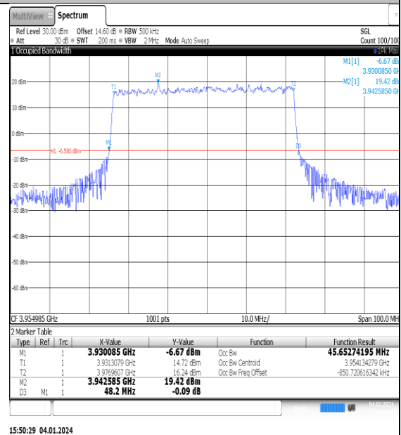
NTNV_N77-3700- 3980_PC2_30_50_H_TID1_Ant1#1
