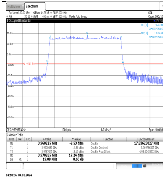
NTNV_N77-3700- 3980_PC2_30_20_H_TID3_Ant1#1
