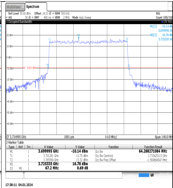
NTNV_N77-3700- 3980_PC2_30_70_L_TID2_Ant1#1
