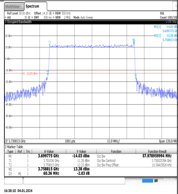
NTNV_N77-3700- 3980_PC2_30_60_L_TID4_Ant1#1
