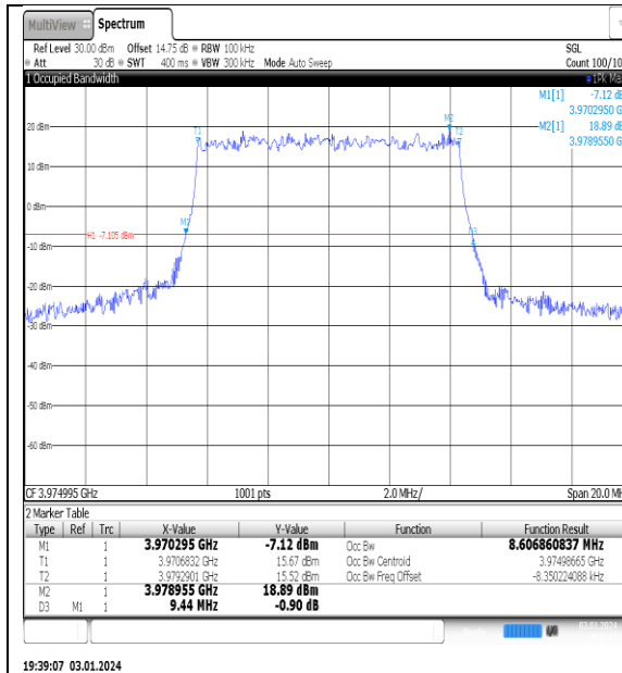
NTNV_N77-3700- 3980_PC2_30_10_H_TID2_Ant1#1
