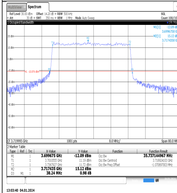
NTNV_N77-3700- 3980_PC2_30_40_L_TID4_Ant1#1
