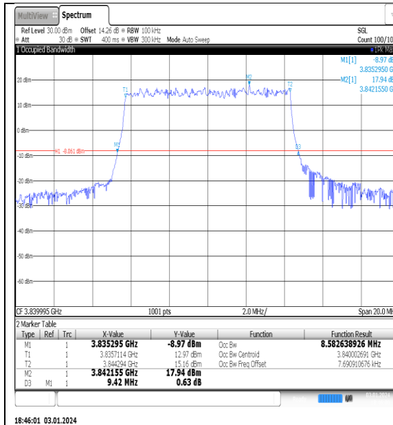
NTNV_N77-3700- 3980_PC2_30_10_M_TID1_Ant1#1
