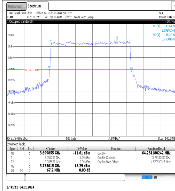
NTNV_N77-3700- 3980_PC2_30_70_L_TID3_Ant1#1
