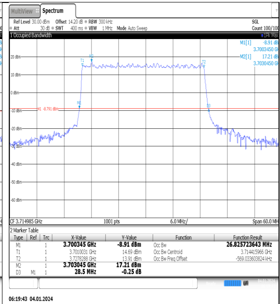
NTNV_N77-3700- 3980_PC2_30_30_L_TID2_Ant1#1
