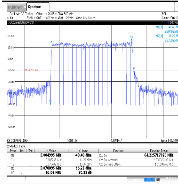
NTNV_N77-3700- 3980_PC2_30_70_M_TID3_Ant1#1
