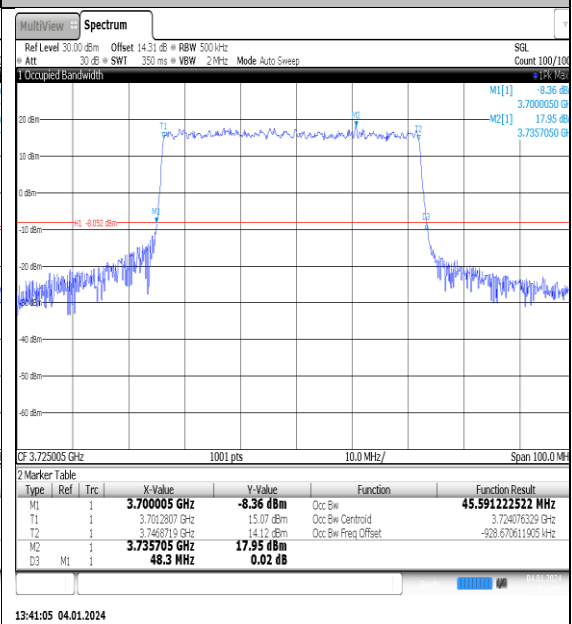
NTNV_N77-3700- 3980_PC2_30_50_L_TID1_Ant1#1
