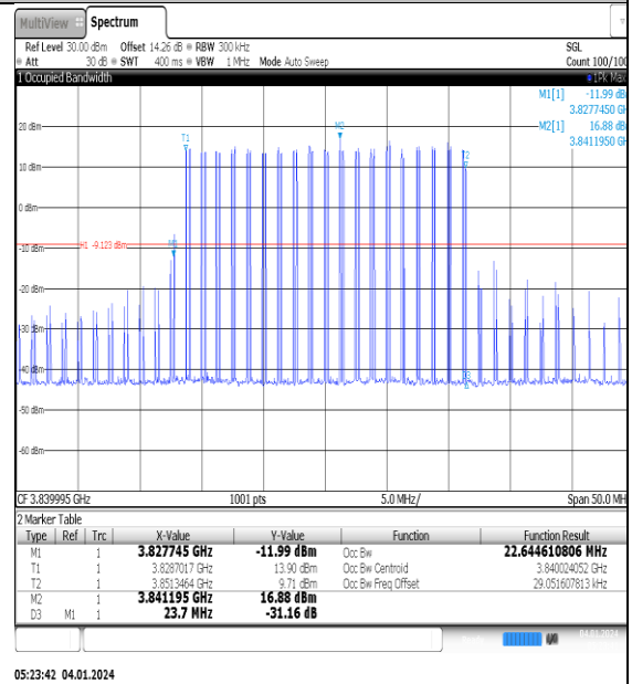
NTNV_N77-3700- 3980_PC2_30_25_M_TID3_Ant1#1
