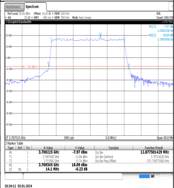
NTNV_N77-3700- 3980_PC2_30_15_L_TID2_Ant1#1
