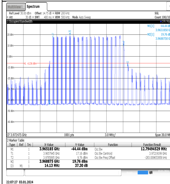
NTNV_N77-3700- 3980_PC2_30_15_H_TID1_Ant1#1
