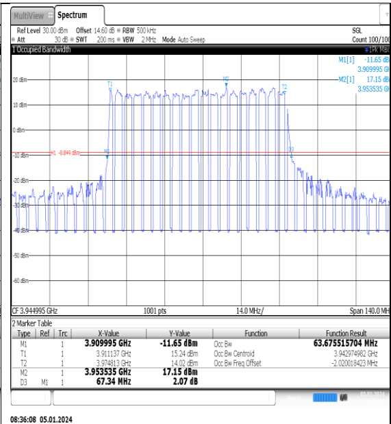
NTNV_N77-3700- 3980_PC2_30_70_H_TID2_Ant1#1
