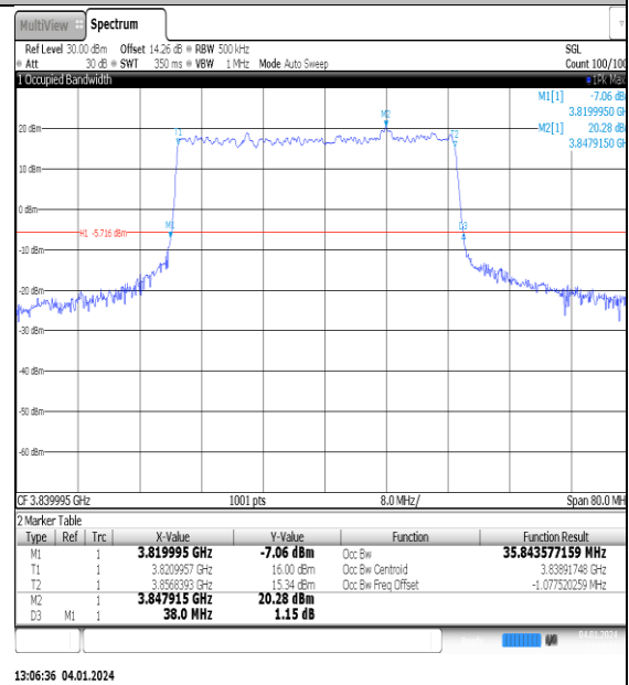
NTNV_N77-3700- 3980_PC2_30_40_M_TID1_Ant1#1
