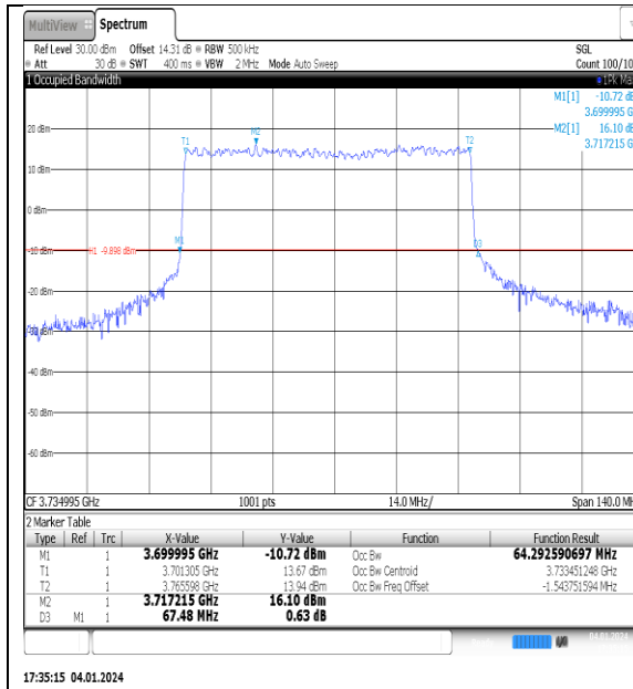
NTNV_N77-3700- 3980_PC2_30_70_L_TID1_Ant1#1
