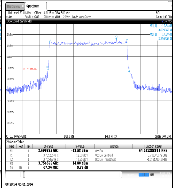
NTNV_N77-3700- 3980_PC2_30_70_L_TID4_Ant1#1
