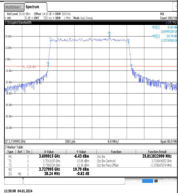
NTNV_N77-3700- 3980_PC2_30_40_L_TID1_Ant1#1
