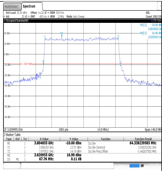
NTNV_N77-3700- 3980_PC2_30_70_M_TID2_Ant1#1
