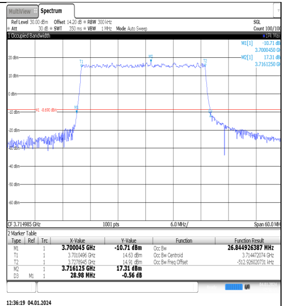
NTNV_N77-3700- 3980_PC2_30_30_L_TID1_Ant1#1
