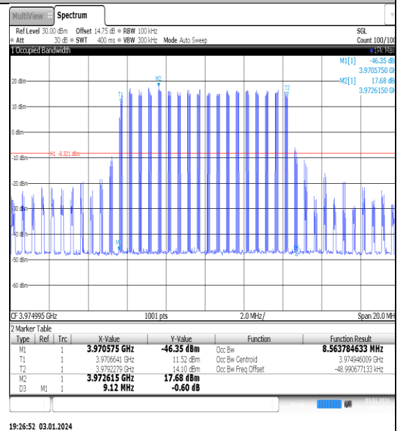
NTNV_N77-3700- 3980_PC2_30_10_H_TID1_Ant1#1
