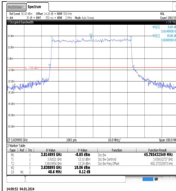
NTNV_N77-3700- 3980_PC2_30_50_M_TID2_Ant1#1
