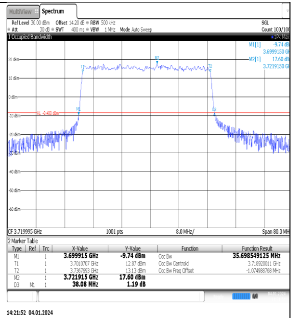
NTNV_N77-3700- 3980_PC2_30_40_L_TID3_Ant1#1
