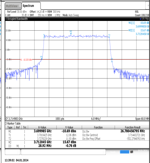
NTNV_N77-3700- 3980_PC2_30_30_L_TID4_Ant1#1
