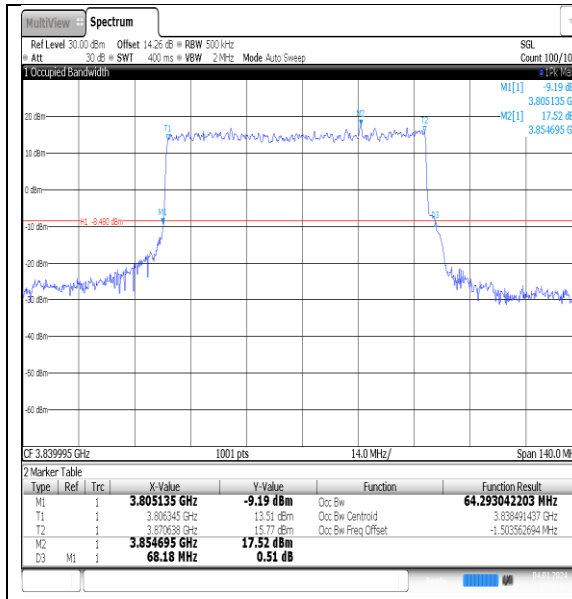
NTNV_N77-3700- 3980_PC2_30_70_M_TID1_Ant1#1
