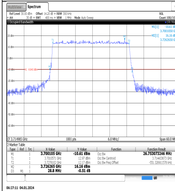
NTNV_N77-3700- 3980_PC2_30_30_L_TID3_Ant1#1
