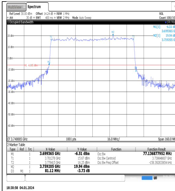
NTNV_N77-3700-3980_PC2_30_80_L_TID1_Ant1#1
