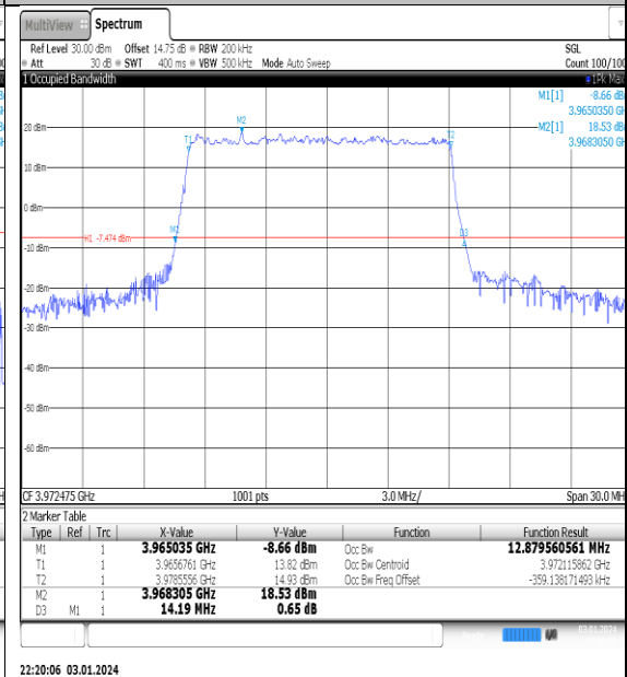
NTNV_N77-3700- 3980_PC2_30_15_H_TID3_Ant1#1
