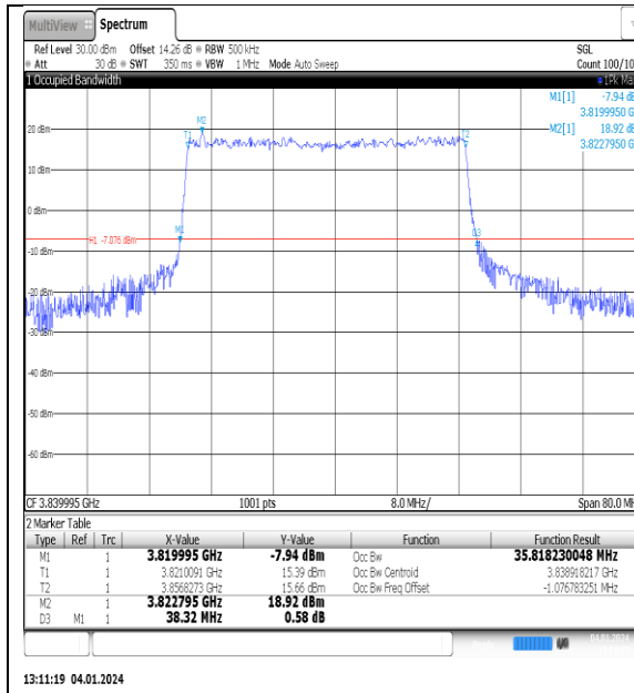
NTNV_N77-3700- 3980_PC2_30_40_M_TID2_Ant1#1
