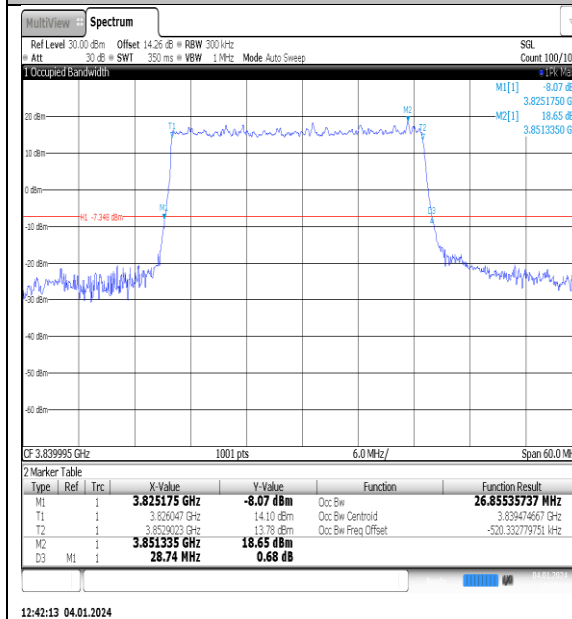
NTNV_N77-3700- 3980_PC2_30_30_M_TID1_Ant1#1
