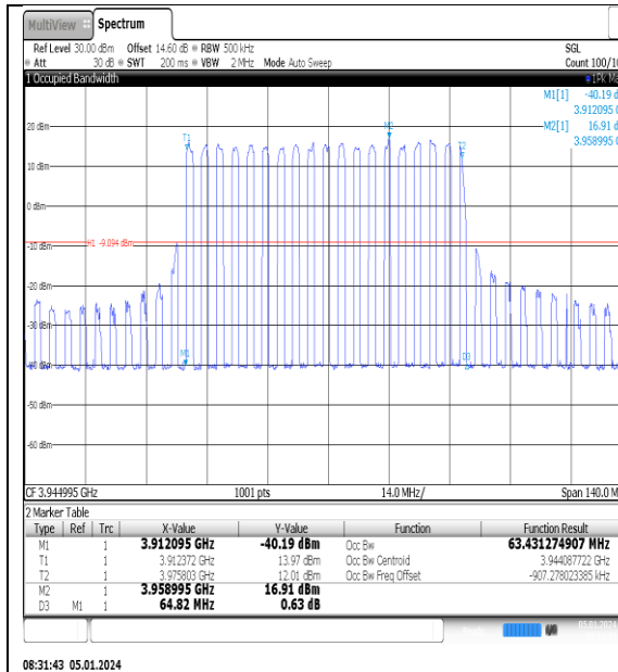
NTNV_N77-3700- 3980_PC2_30_70_H_TID1_Ant1#1
