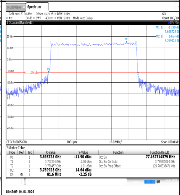
NTNV_N77-3700-3980_PC2_30_80_L_TID4_Ant1#1
