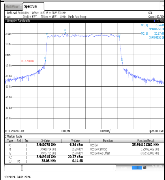
NTNV_N77-3700- 3980_PC2_30_40_H_TID1_Ant1#1
