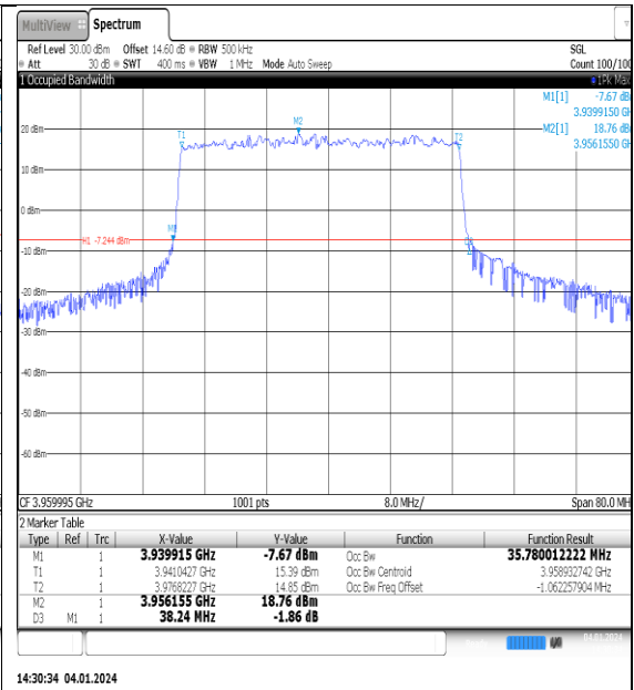
NTNV_N77-3700- 3980_PC2_30_40_H_TID3_Ant1#1
