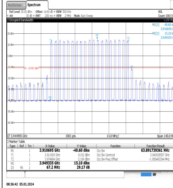
NTNV_N77-3700- 3980_PC2_30_70_H_TID3_Ant1#1
