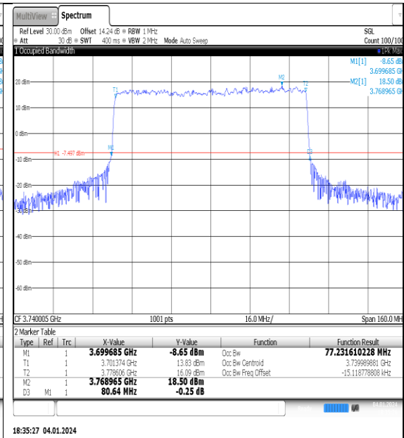
NTNV_N77-3700-3980_PC2_30_80_L_TID2_Ant1#1
