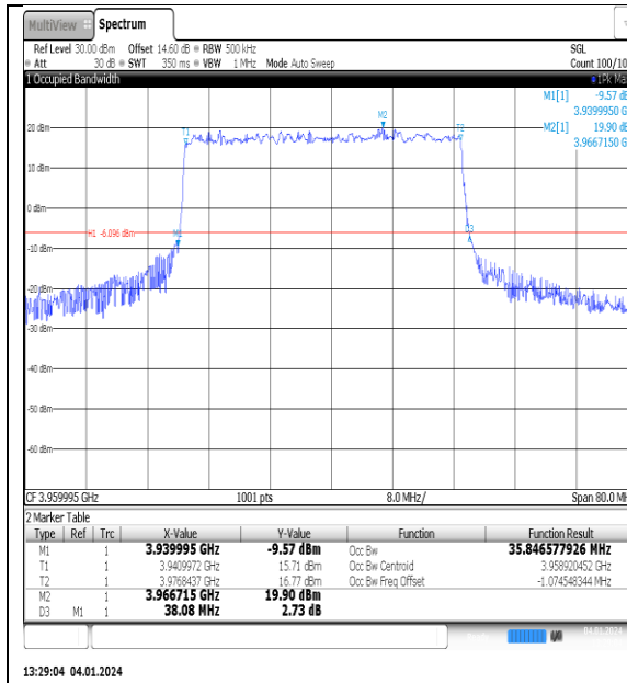
NTNV_N77-3700- 3980_PC2_30_40_H_TID2_Ant1#1
