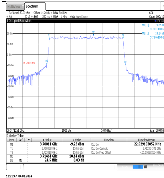
NTNV_N77-3700- 3980_PC2_30_25_L_TID2_Ant1#1
