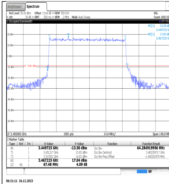
NTNV_N77-3450- 3550_PC2_30_70_L_TID1_Ant1#1
