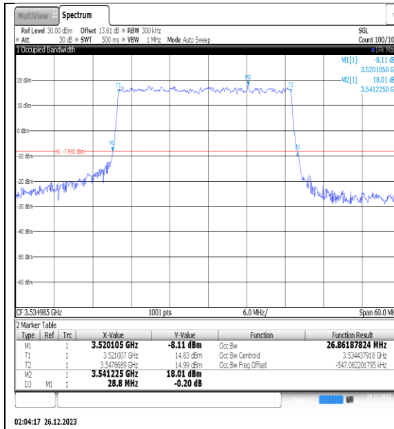
NTNV_N77-3450-3550_PC2_30_30_H_TID1_Ant1#1
