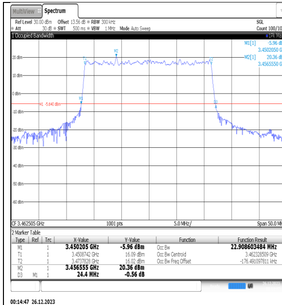
NTNV_N77-3450- 3550_PC2_30_25_L_TID1_Ant1#1
