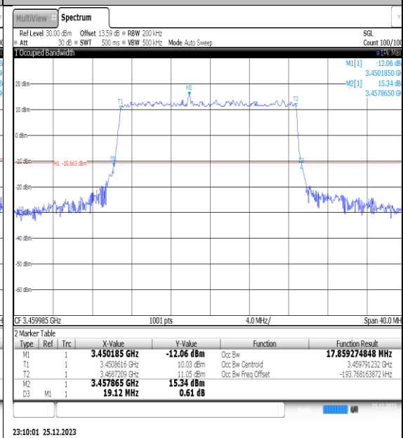
NTNV_N77-3450- 3550_PC2_30_20_L_TID4_Ant1#1
