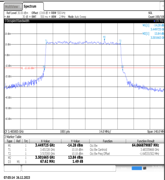
NTNV_N77-3450- 3550_PC2_30_70_L_TID4_Ant1#1
