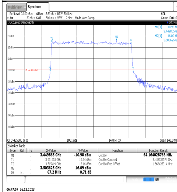
NTNV_N77-3450- 3550_PC2_30_70_L_TID3_Ant1#1
