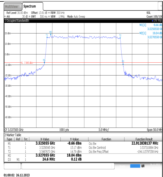
NTNV_N77-3450- 3550_PC2_30_25_H_TID2_Ant1#1
