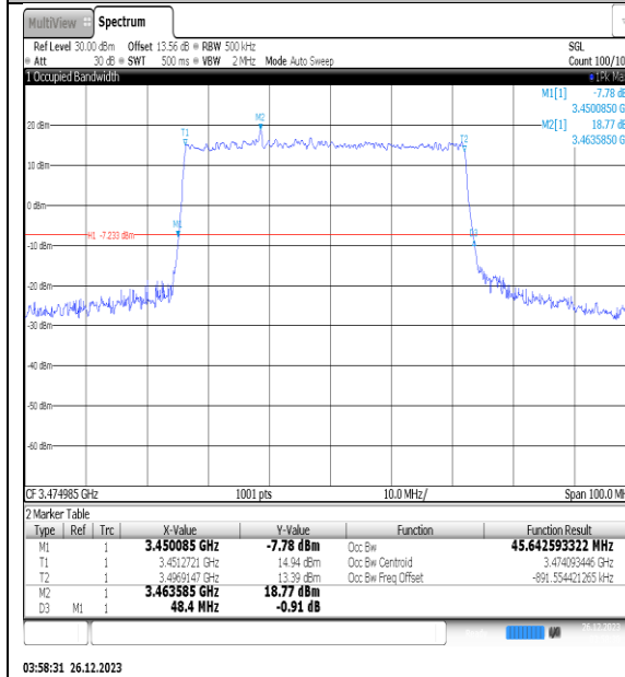
NTNV_N77-3450- 3550_PC2_30_50_L_TID3_Ant1#1
