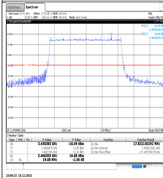
NTNV_N77-3450- 3550_PC2_30_20_L_TID3_Ant1#1
