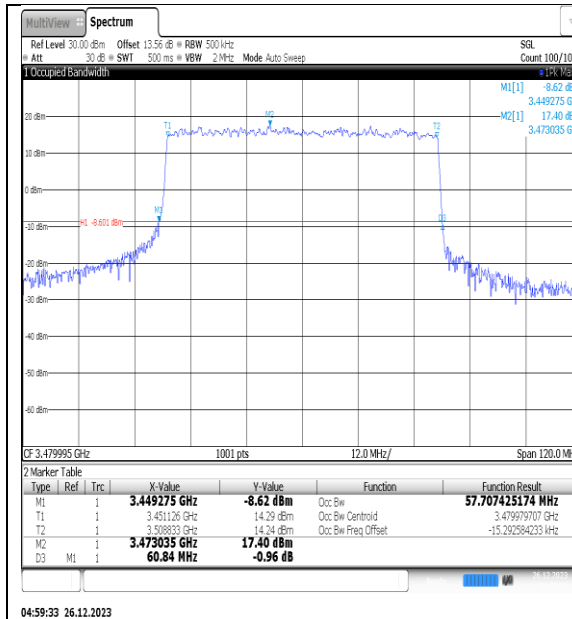
NTNV_N77-3450- 3550_PC2_30_60_L_TID1_Ant1#1
