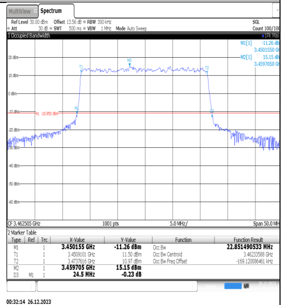
NTNV_N77-3450- 3550_PC2_30_25_L_TID4_Ant1#1
