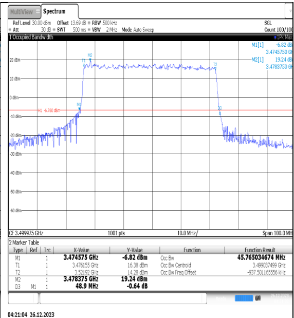
NTNV_N77-3450- 3550_PC2_30_50_M_TID2_Ant1#1
