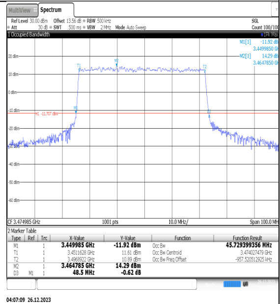
NTNV_N77-3450- 3550_PC2_30_50_L_TID4_Ant1#1
