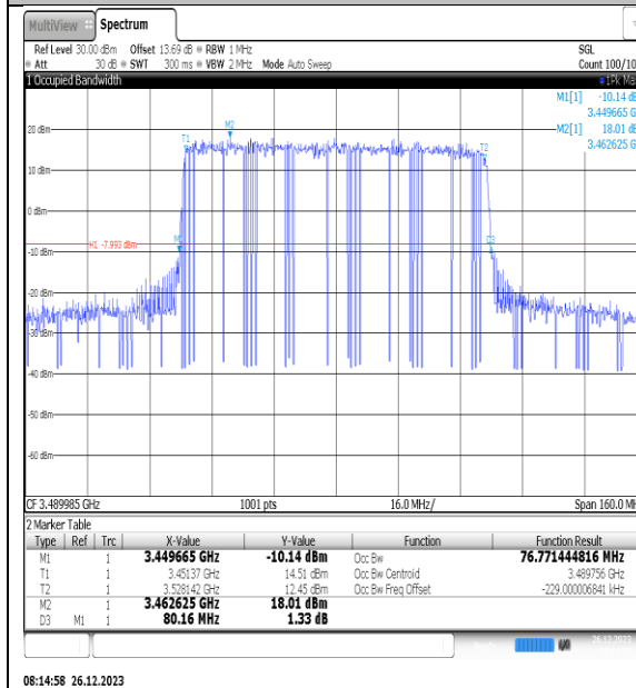
NTNV_N77-3450- 3550_PC2_30_80_L_TID3_Ant1#1
