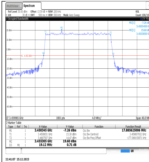
NTNV_N77-3450- 3550_PC2_30_20_L_TID1_Ant1#1
