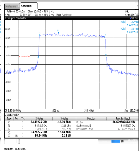
NTNV_N77-3450- 3550_PC2_30_90_L_TID4_Ant1#1
