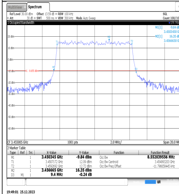
NTNV_N77-3450- 3550_PC2_30_10_L_TID3_Ant1#1
