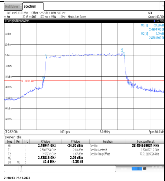
NTNV_N7_PC3_15_40_L_TID6_Ant1#1
