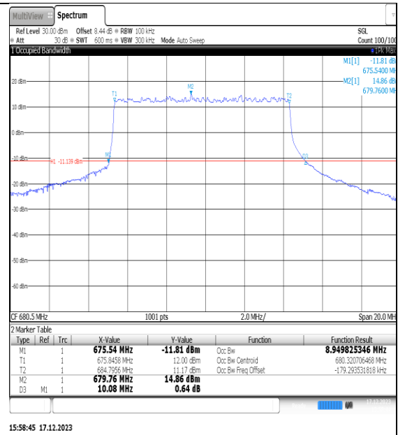
NTNV_N71_PC3_15_10_M_TID2_Ant1#1
