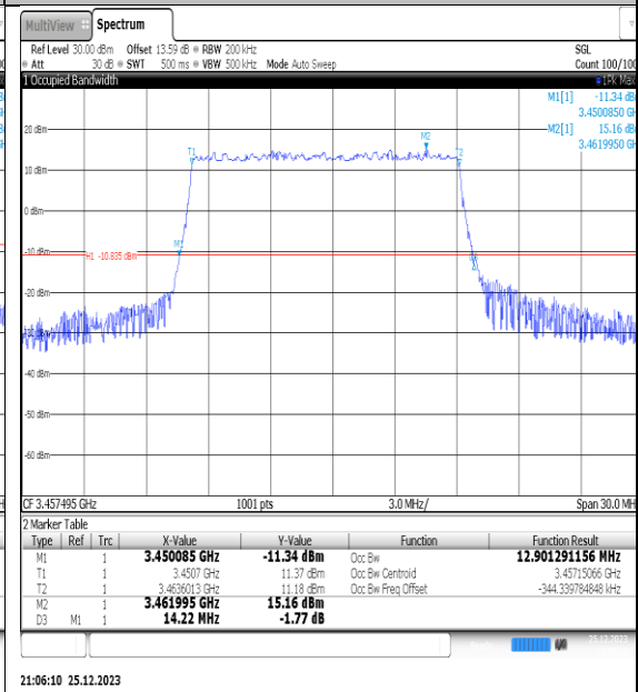
NTNV_N77-3450- 3550_PC2_30_15_L_TID4_Ant1#1
