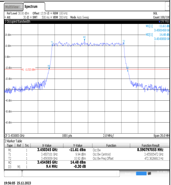
NTNV_N77-3450- 3550_PC2_30_10_L_TID4_Ant1#1
