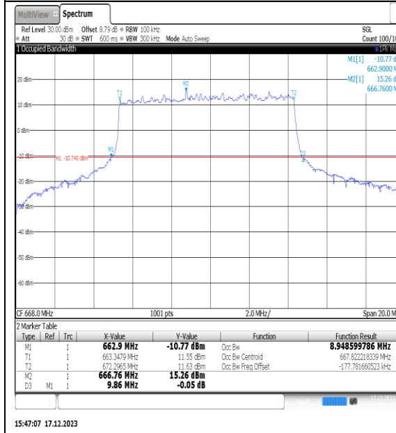
NTNV_N71_PC3_15_10_L_TID3_Ant1#1
