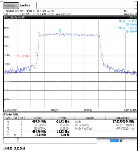
NTNV_N71_PC3_15_20_H_TID2_Ant1#1
