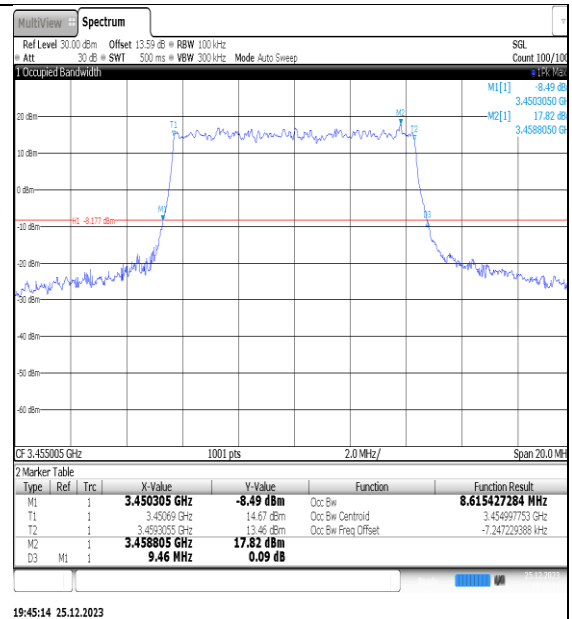
NTNV_N77-3450- 3550_PC2_30_10_L_TID2_Ant1#1
