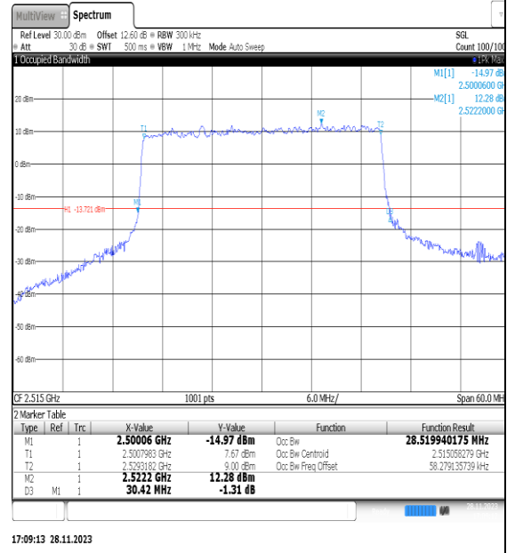
NTNV_N7_PC3_15_30_L_TID1_Ant1#1
