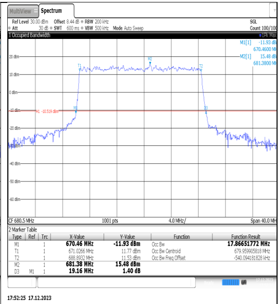
NTNV_N71_PC3_15_20_M_TID2_Ant1#1
