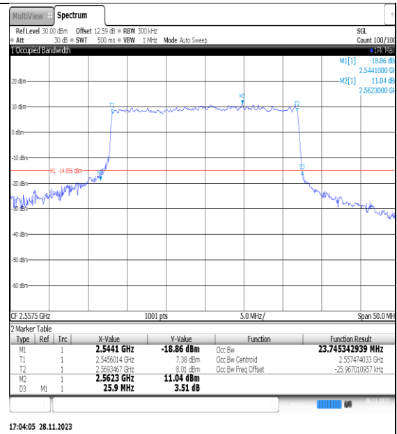
NTNV_N7_PC3_15_25_H_TID7_Ant1#1
