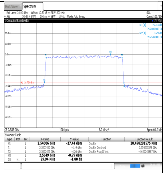
NTNV_N7_PC3_15_30_H_TID6_Ant#1
