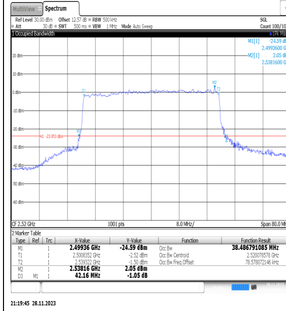
NTNV_N7_PC3_15_40_L_TID7_Ant1#1
