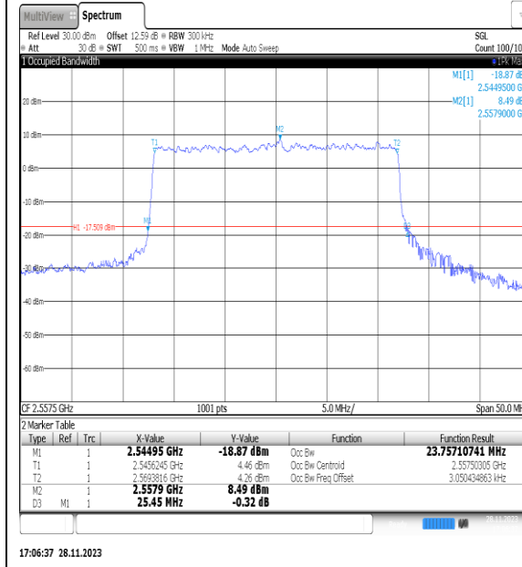
NTNV_N7_PC3_15_25_H_TID8_Ant1#1
