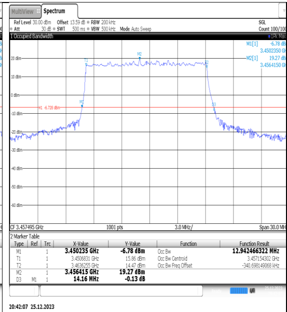
NTNV_N77-3450- 3550_PC2_30_15_L_TID2_Ant1#1
