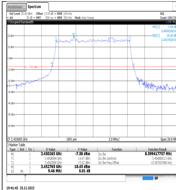
NTNV_N77-3450- 3550_PC2_30_10_L_TID1_Ant1#1
