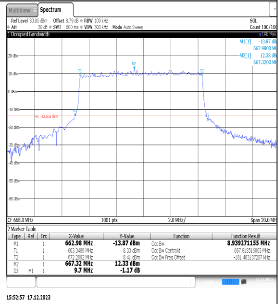
NTNV_N71_PC3_15_10_L_TID4_Ant1#1
