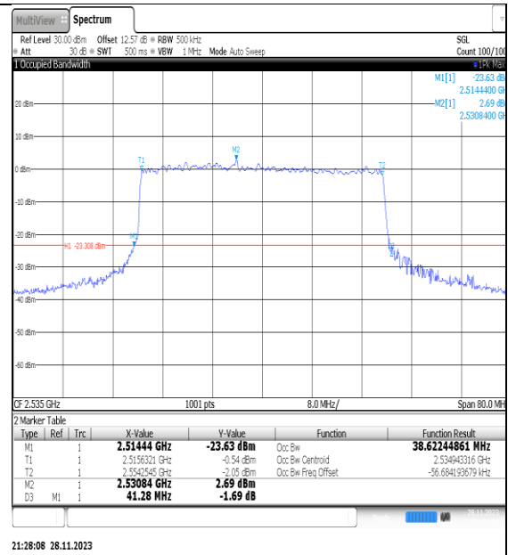
NTNV_N7_PC3_15_40_M_TID2_Ant#1
