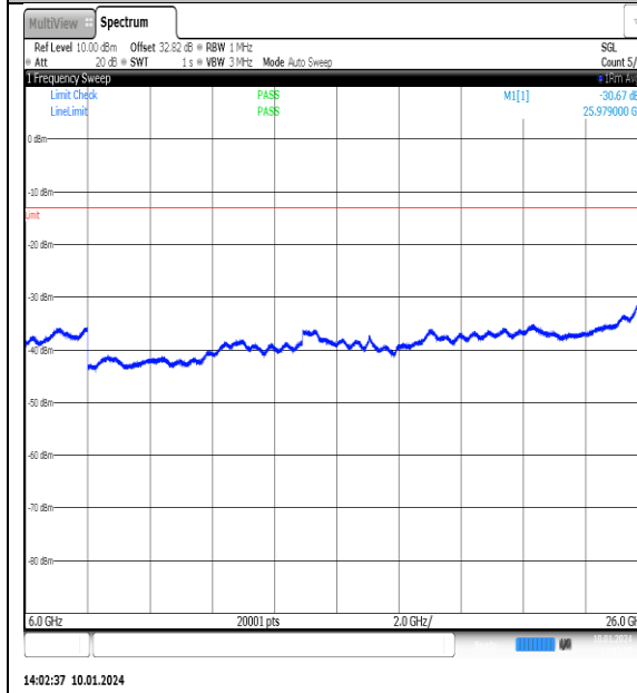
NTNV_N77-3700- 3980_PC2_30_100_L_TID15_NS_01_6000_2600 0_#1
