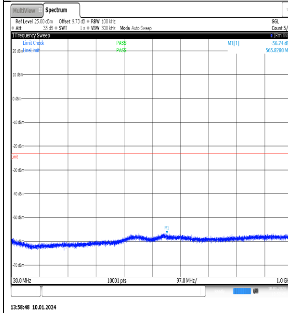
NTNV_N77-3700- 3980_PC2_30_100_L_TID14_NS_01_30_1000_# 1
