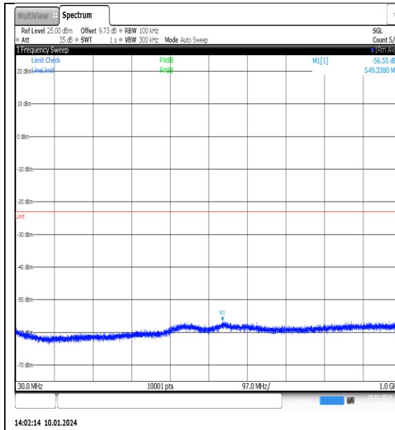
NTNV_N77-3700- 3980_PC2_30_100_L_TID15_NS_01_30_1000_# 1
