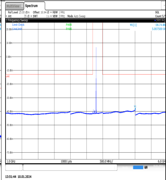
NTNV_N77-3700- 3980_PC2_30_100_L_TID12_NS_01_1000_6000 #1
