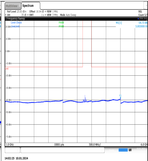
NTNV_N77-3700- 3980_PC2_30_100_L_TID15_NS_01_1000_6000 _#1
