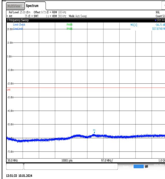
NTNV_N77-3700- 3980_PC2_30_100_L_TID12_NS_01_30_1000_# 1
