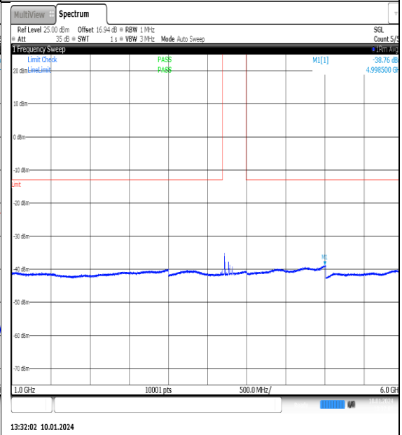
NTNV_N77-3700- 3980_PC2_30_100_L_TID8_NS_01_1000_6000_ #1
