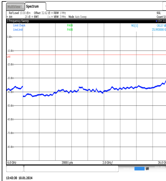
NTNV_N77-3700- 3980_PC2_30_100_L_TID10_NS_01_6000_2600 _0_#1
