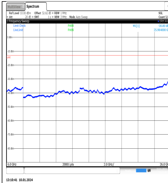
NTNV_N77-3700- 3980_PC2_30_100_L_TID2_NS_01_6000_26000 _#1
