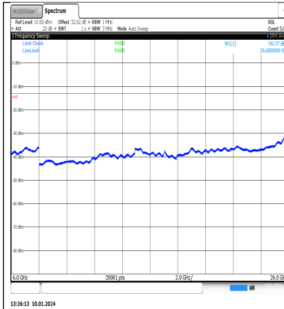
NTNV_N77-3700- 3980_PC2_30_100_L_TID6_NS_01_6000_26000 _#1
