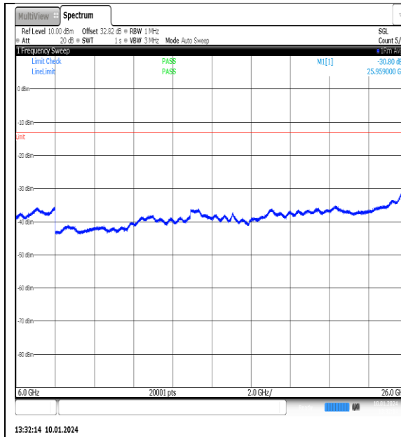
NTNV_N77-3700-3980_PC2_30_100_L_TID8_NS_01_6000_26000_#1
