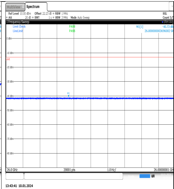
NTNV_N77-3700- 3980_PC2_30_100_L_TID10_NS_01_26000_400 _00_#1
