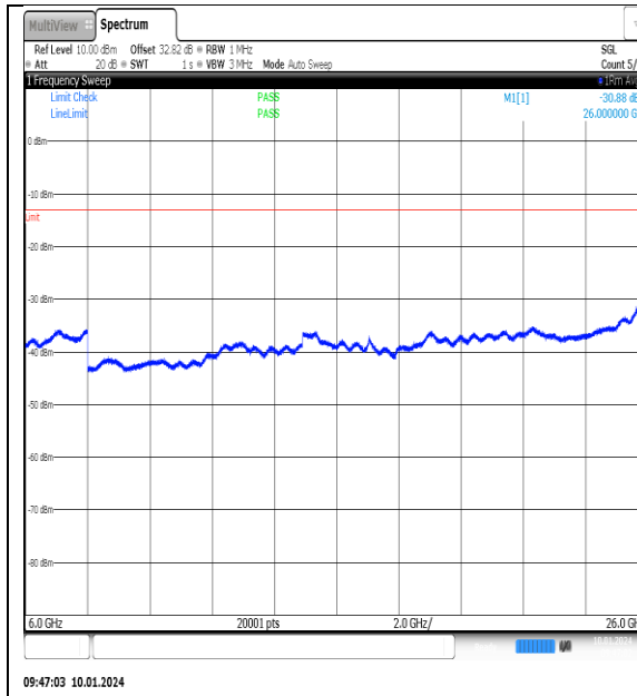
NTNV_N77-3700- 3980_PC2_30_90_L_TID3_NS_01_6000_26000_#1
