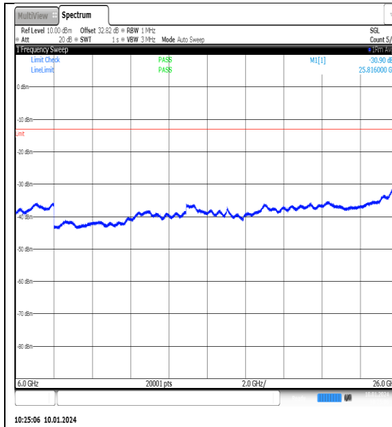
NTNV_N77-3700- 3980_PC2_30_90_L_TID13_NS_01_6000_26000 _#1
