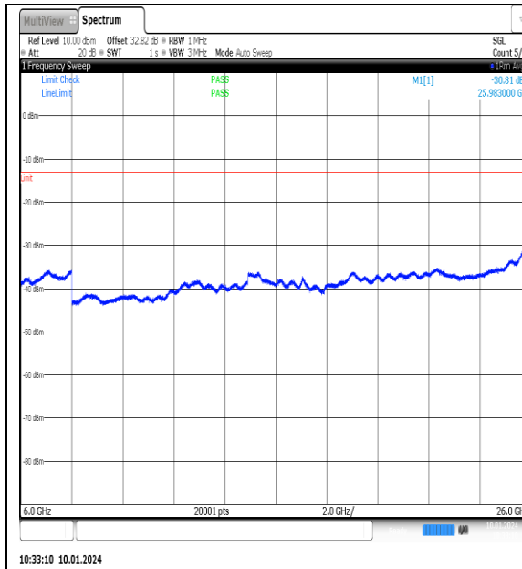
NTNV_N77-3700- 3980_PC2_30_90_L_TID15_NS_01_6000_26000 _#1
