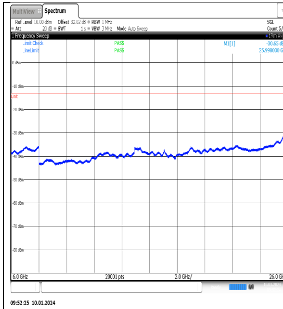
NTNV_N77-3700- 3980_PC2_30_90_L_TID5_NS_01_6000_26000_#1
