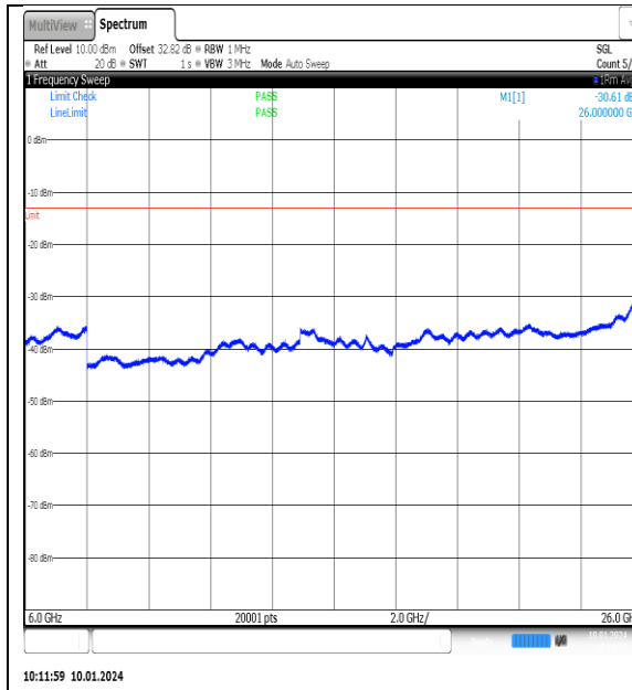
NTNV_N77-3700- 3980_PC2_30_90_L_TID9_NS_01_6000_26000_#1
