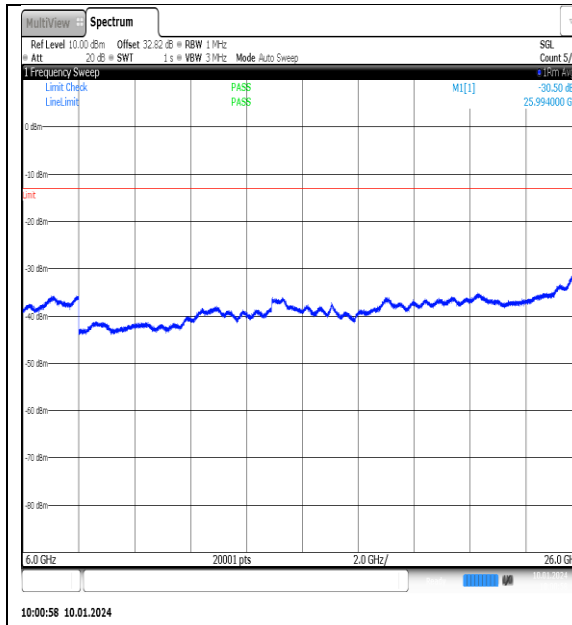
NTNV_N77-3700- 3980_PC2_30_90_L_TID7_NS_01_6000_26000_ #1
