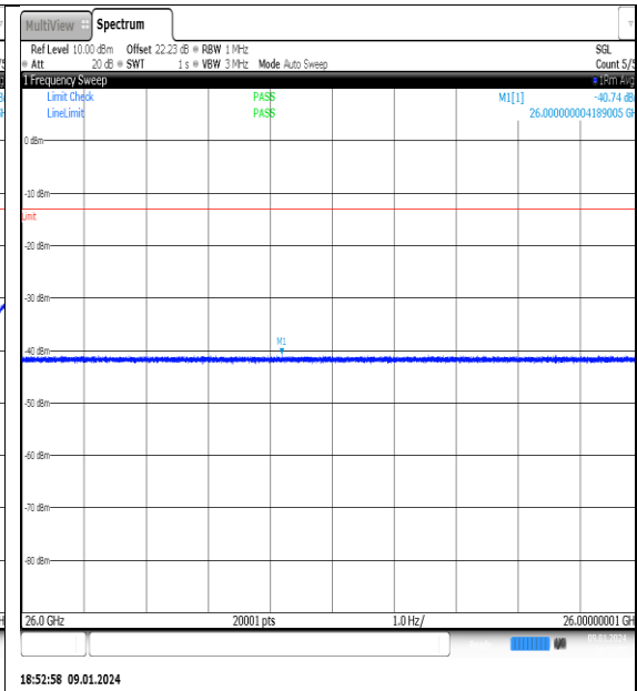
NTNV_N77-3700- 3980_PC2_30_80_L_TID13_NS_01_26000_4000 0_#1
