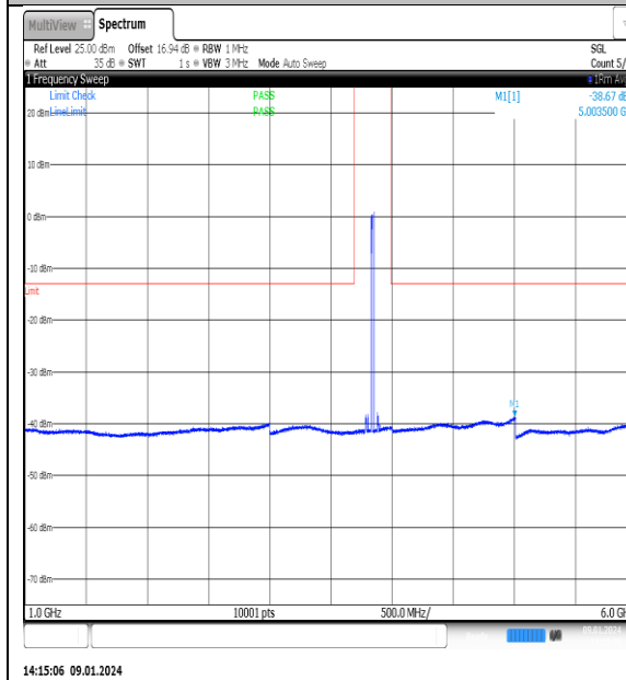
NTNV_N77-3700-3980_PC2_30_70_M_TID13_NS_01_1000_6000_#1
