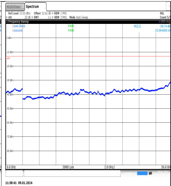
NTN_V_N77-3700- 3980_PC2_30_70_L_TID11_NS_01_6000_26000 #1
