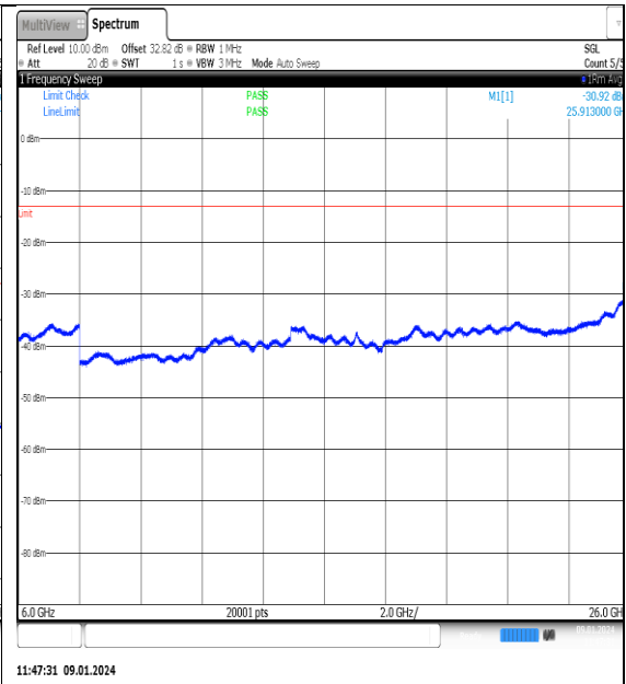
NTN V _N77-3700- 3980_PC2_30_70_L_TID9_NS_01_6000_26000_# #1
