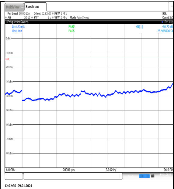
NTN_V_N77-3700- 3980_PC2_30_70_L_TID15_NS_01_6000_26000 #1
