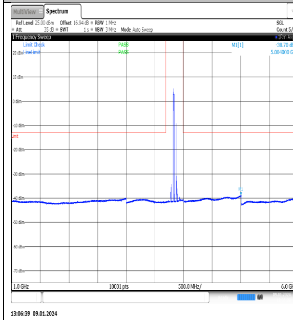
NTNV_N77-3700- 3980_PC2_30_70_M_TID7_NS_01_1000_6000_#1
