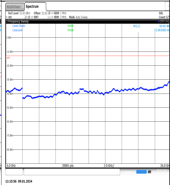
NTN_V_N77-3700- 3980_PC2_30_70_L_TID14_NS_01_6000_26000_#1
