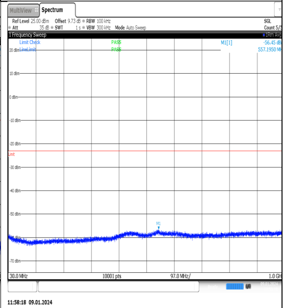
NTNV_N77-3700- 3980_PC2_30_70_L_TID11_NS_01_30_1000_#1
