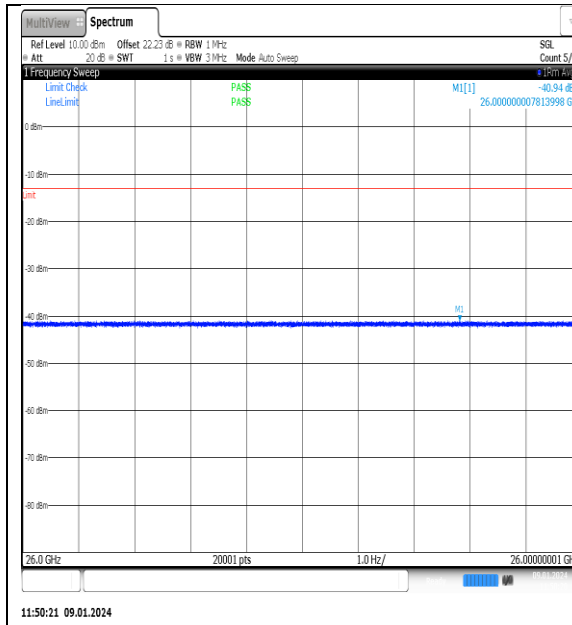
NTNV_N77-3700- 3980_PC2_30_70_L_TID10_NS_01_26000_4000 0_#1
