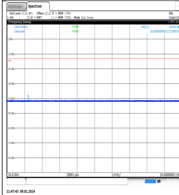
NTN V _N77-3700- 3980_PC2_30_70_L_TID9_NS_01_26000_40000_# #1
