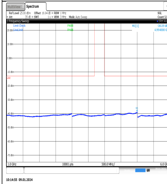
NTNV_N77-3700- 3980_PC2_30_60_H_TID5_NS_01_1000_6000_#1
