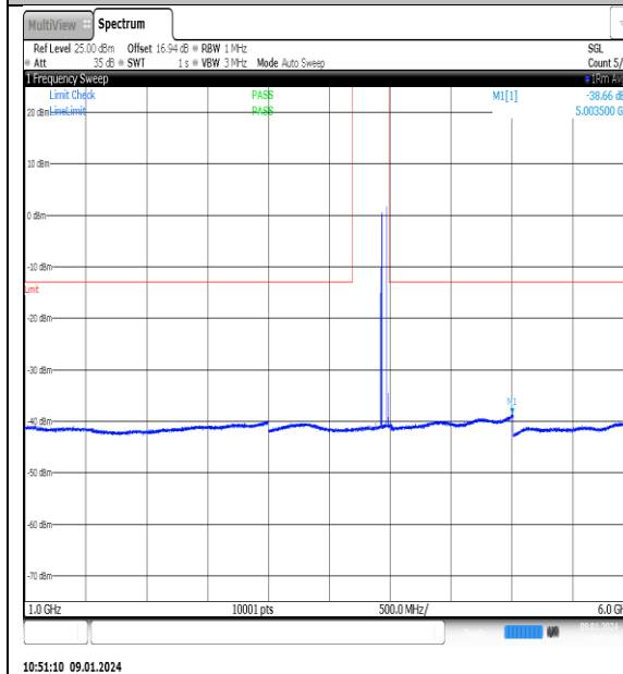
NTNV_N77-3700-3980_PC2_30_60_H_TID13_NS_01_1000_6000_#1
