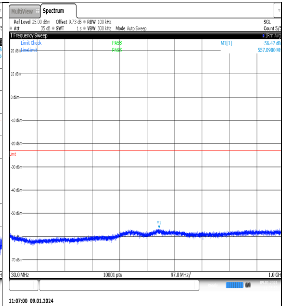
NTNV_N77-3700- 3980_PC2_30_70_L_TID2_NS_01_30_1000_#1
