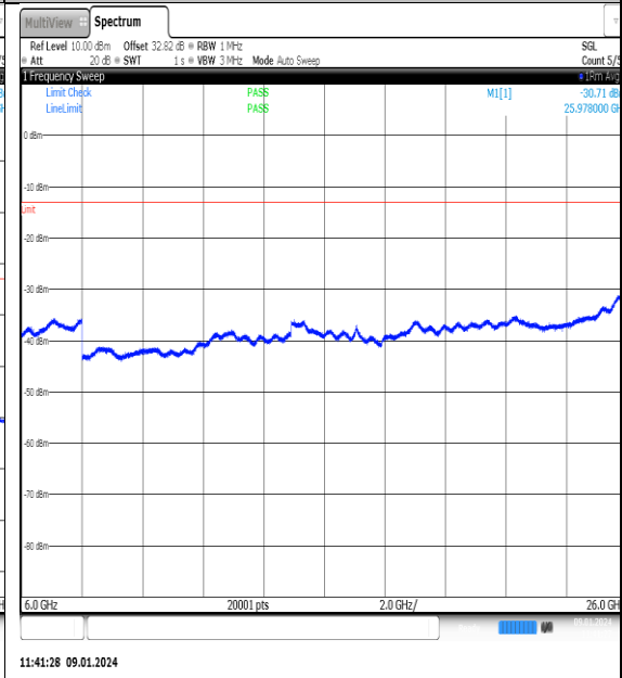
NTNV_N77-3700- 3980_PC2_30_70_L_TID8_NS_01_6000_26000_#1
