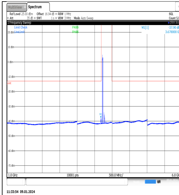
NTN_V_N77-3700- 3980_PC2_30_70_L_TID7_NS_01_1000_6000_# 1
