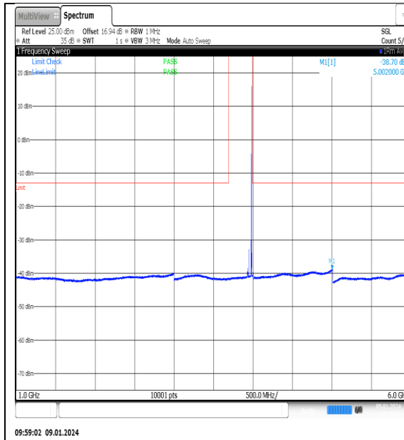
09:59:02 09.01.2024 NTN_V_N77-3700- 3980_PC2_30_60_H_TID3_NS_01_1000_6000_# 1
