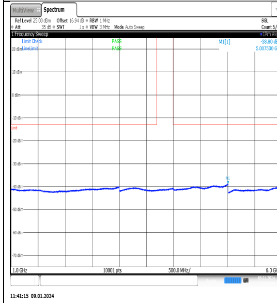
NTNV_N77-3700- 3980_PC2_30_70_L_TID8_NS_01_1000_6000_#1
