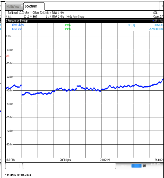
NTN_V_N77-3700- 3980_PC2_30_70_L_TID7_NS_01_6000_26000_# #1
