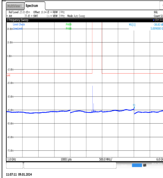
NTNV_N77-3700- 3980_PC2_30_70_L_TID2_NS_01_1000_6000_#1
