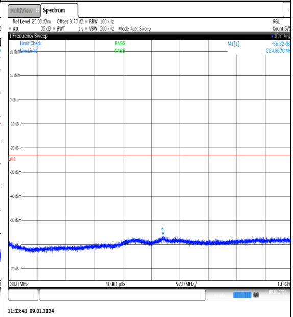
NTNV_N77-3700- 3980_PC2_30_70_L_TID7_NS_01_30_1000_#1
