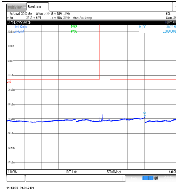
NTN_V_N77-3700- 3980_PC2_30_70_L_TID3_NS_01_1000_6000_# 1
