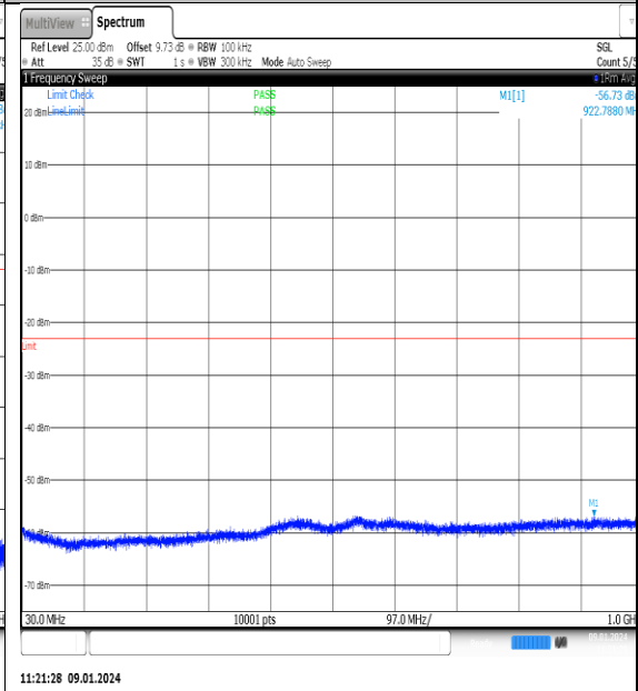
NTNV_N77-3700- 3980_PC2_30_70_L_TID5_NS_01_30_1000_#1
