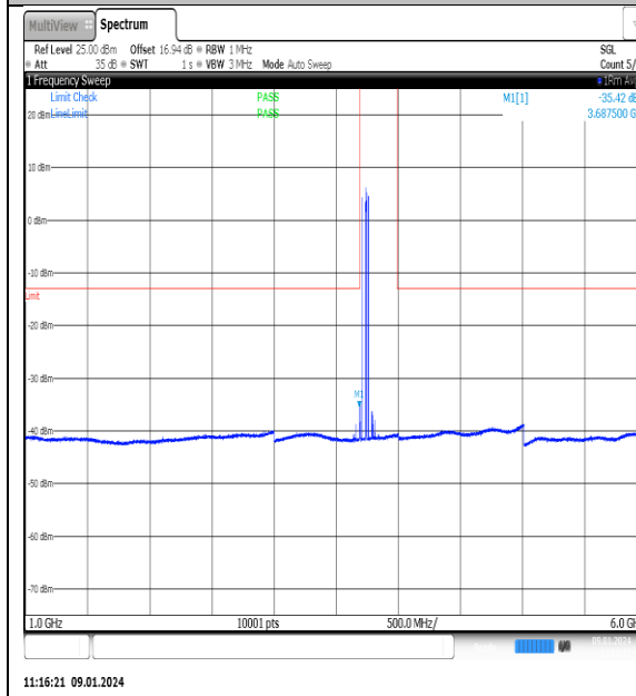
NTNV_N77-3700-3980_PC2_30_70_L_TID4_NS_01_1000_6000_#1
