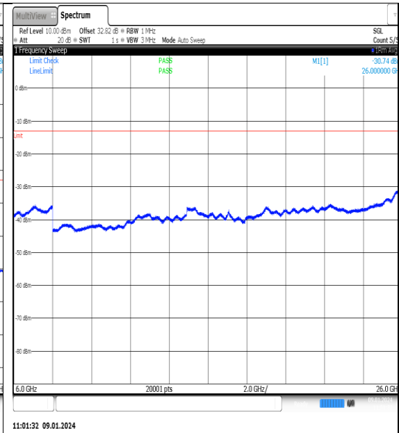
NTN_V_N77-3700- 3980_PC2_30_70_L_TID1_NS_01_6000_26000_# #1
