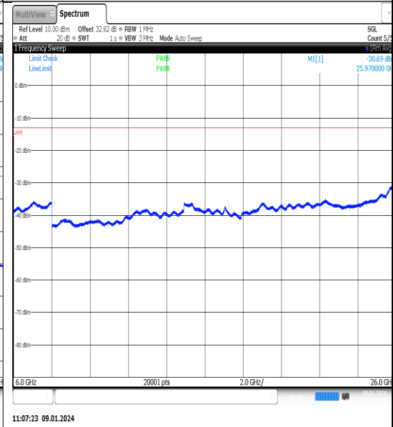
NTNV_N77-3700- 3980_PC2_30_70_L_TID2_NS_01_6000_26000_#1
