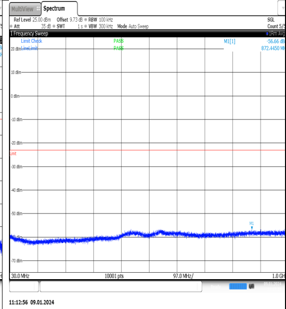
NTNV_N77-3700- 3980_PC2_30_70_L_TID3_NS_01_30_1000_#1
