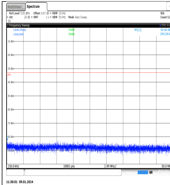
NTNV_N77-3700-3980_PC2_30_70_L_TID6_NS_01_0.15_30_#1
