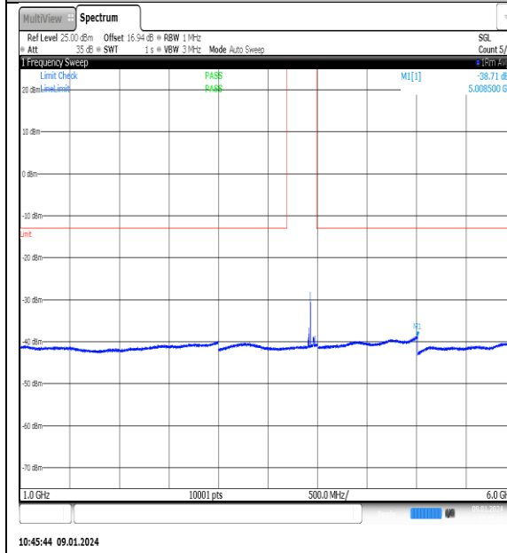
NTNV_N77-3700-3980_PC2_30_60_H_TID11_NS_01_1000_6000_#1
