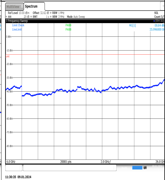
NTNV_N77-3700-3980_PC2_30_70_L_TID6_NS_01_6000_26000_#1
