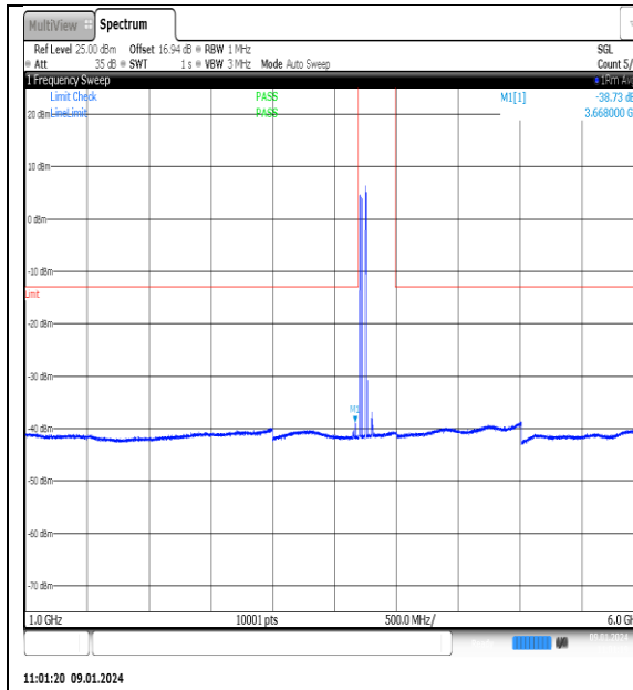
NTN_V_N77-3700- 3980_PC2_30_70_L_TID1_NS_01_1000_6000_# 1
