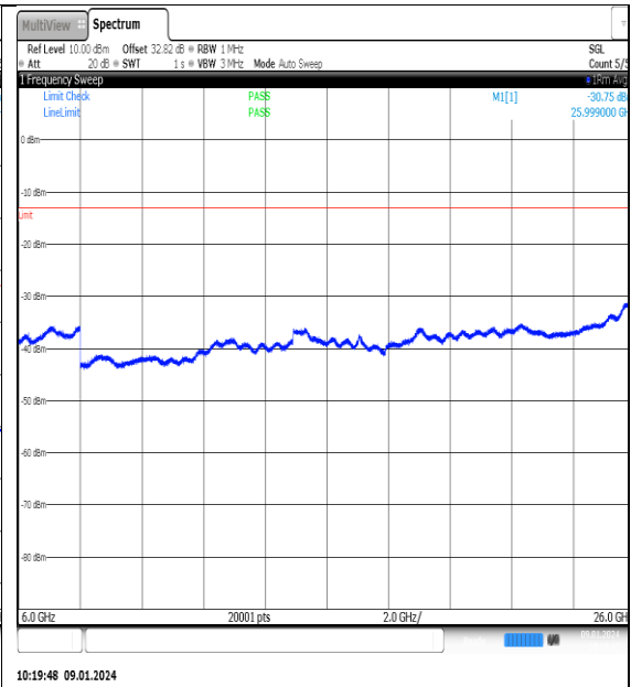
NTNV_N77-3700- 3980_PC2_30_60_H_TID6_NS_01_6000_26000_# #1
