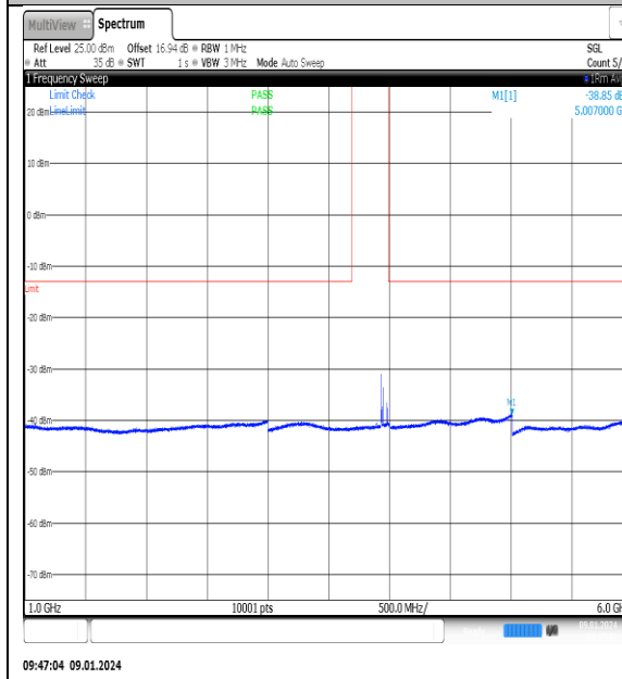
09:47:04 09.01.2024 NTNV_N77-3700- 3980_PC2_30_60_H_TID2_NS_01_1000_6000_#1
