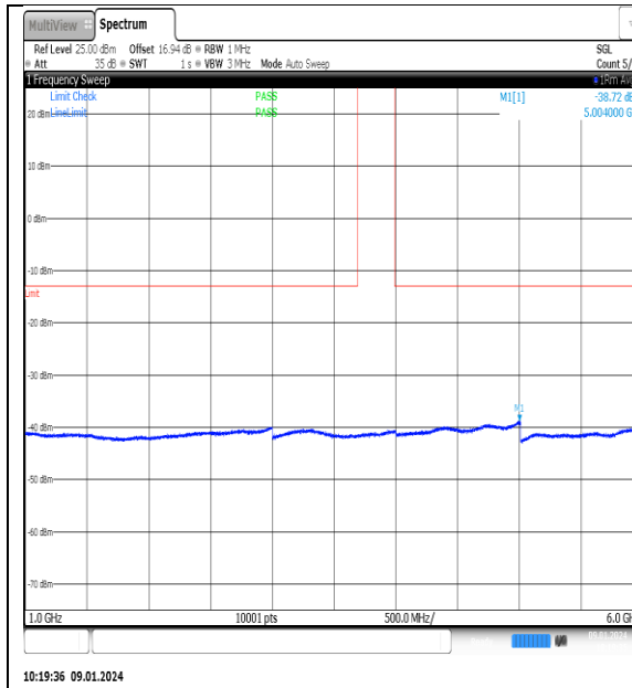
NTNV_N77-3700- 3980_PC2_30_60_H_TID6_NS_01_1000_6000_# 1
