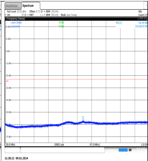
NTNV_N77-3700-3980_PC2_30_70_L_TID6_NS_01_30_1000_#1
