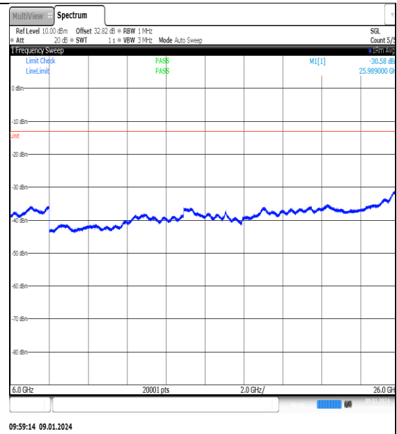
09:59:14 09.01.2024 NTN_V_N77-3700- 3980_PC2_30_60_H_TID3_NS_01_6000_26000_# #1
