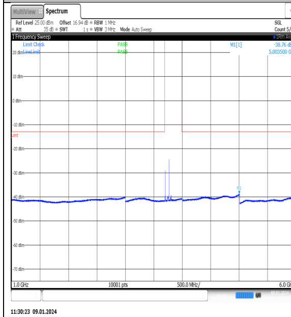
NTNV_N77-3700-3980_PC2_30_70_L_TID6_NS_01_1000_6000_#1
