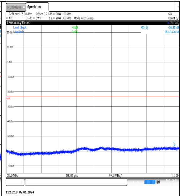
NTNV_N77-3700-3980_PC2_30_70_L_TID4_NS_01_30_1000_#1
