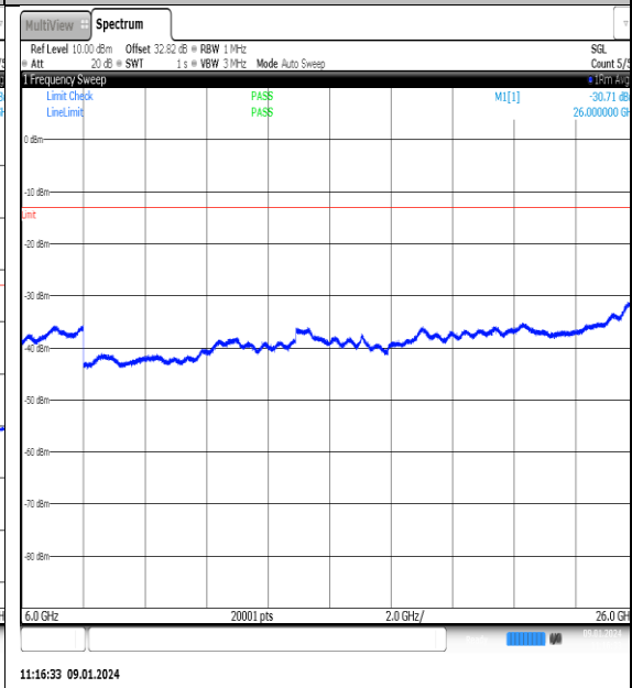
NTNV_N77-3700-3980_PC2_30_70_L_TID4_NS_01_6000_26000_#1
