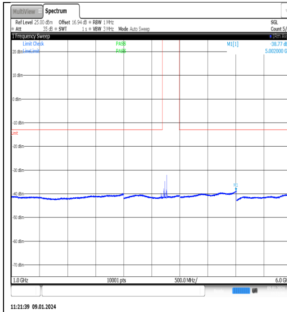
NTN_V_N77-3700- 3980_PC2_30_70_L_TID5_NS_01_1000_6000_# 1
