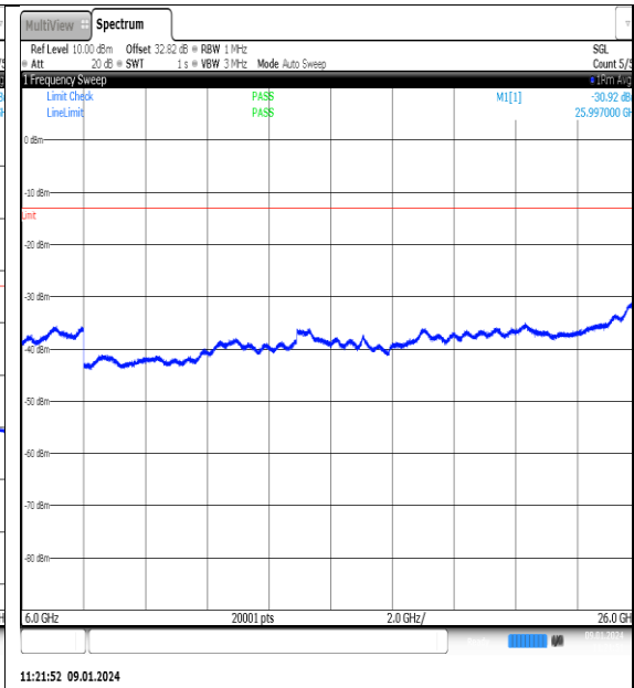
NTN_V_N77-3700- 3980_PC2_30_70_L_TID5_NS_01_6000_26000_# #1
