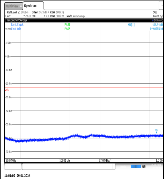
NTNV_N77-3700- 3980_PC2_30_70_L_TID1_NS_01_30_1000_#1
