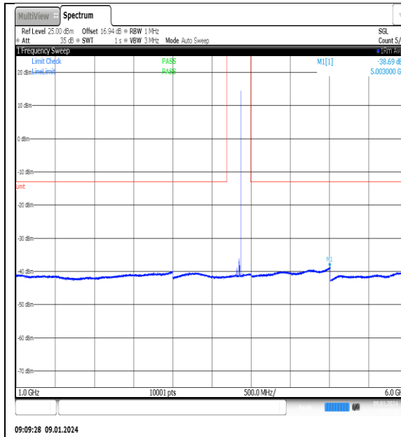
NTN_V_N77-3700- 3980_PC2_30_60_M_TID6_NS_01_1000_6000_# 1
