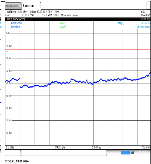
NTN_V_N77-3700- 3980_PC2_30_60_L_TID1_NS_01_6000_26000_# #1
