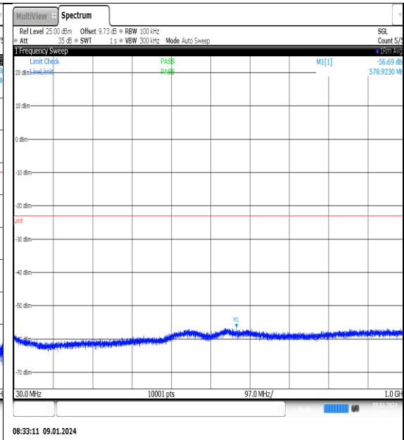
NTNV_N77-3700- 3980_PC2_30_60_L_TID12_NS_01_30_1000_#1
