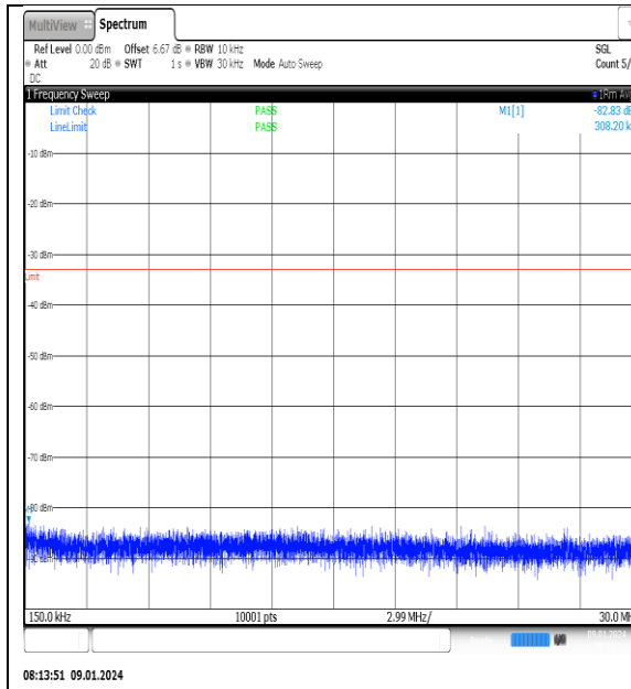
NTNV_N77-3700- 3980_PC2_30_60_L_TID6_NS_01_0.15_30_#1
