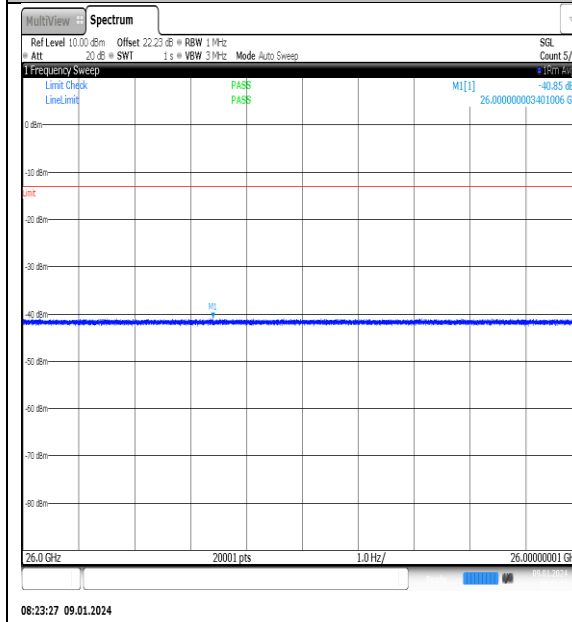
NTN_V_N77-3700- 3980_PC2_30_60_L_TID9_NS_01_26000_40000_# #1
