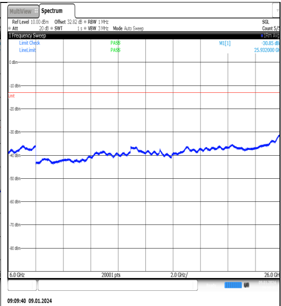
NTN_V_N77-3700- 3980_PC2_30_60_M_TID6_NS_01_6000_26000_# #1
