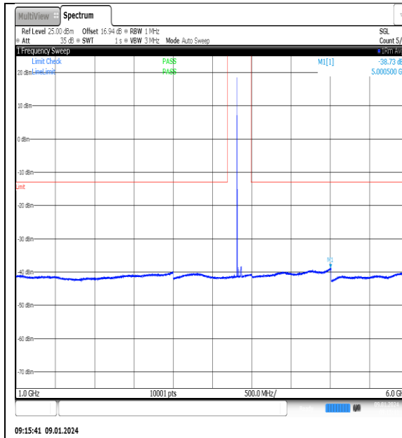
NTNV_N77-3700- 3980_PC2_30_60_M_TID8_NS_01_1000_6000_# 1
