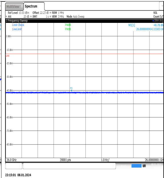
NTNV_N77-3700-3980_PC2_30_50_L_TID15_NS_01_26000_4000_0_#1
