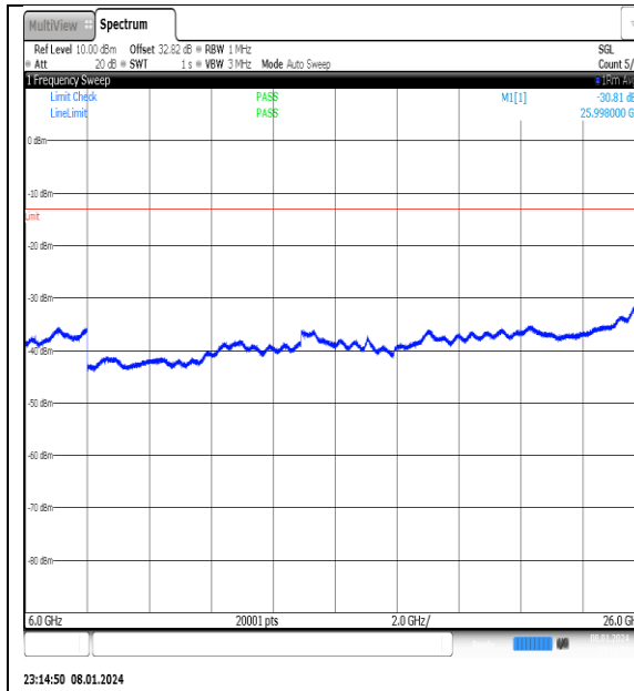
NTNV_N77-3700-3980_PC2_30_50_L_TID15_NS_01_6000_26000_#1
