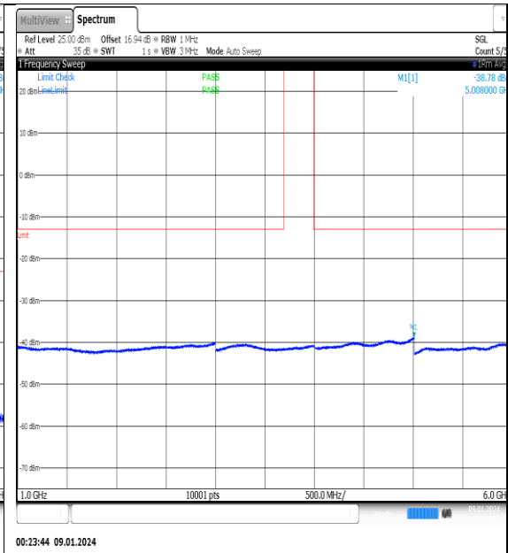
NTNV_N77-3700- 3980_PC2_30_50_H_TID4_NS_01_1000_6000_# 1
