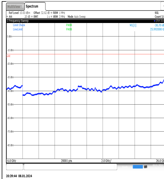
NTNV_N77-3700- 3980_PC2_30_40_L_TID12_NS_01_6000_26000 _#1
