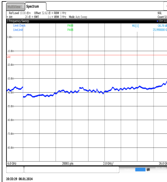
NTNV_N77-3700-3980_PC2_30_40_L_TID10_NS_01_6000_26000_#1
