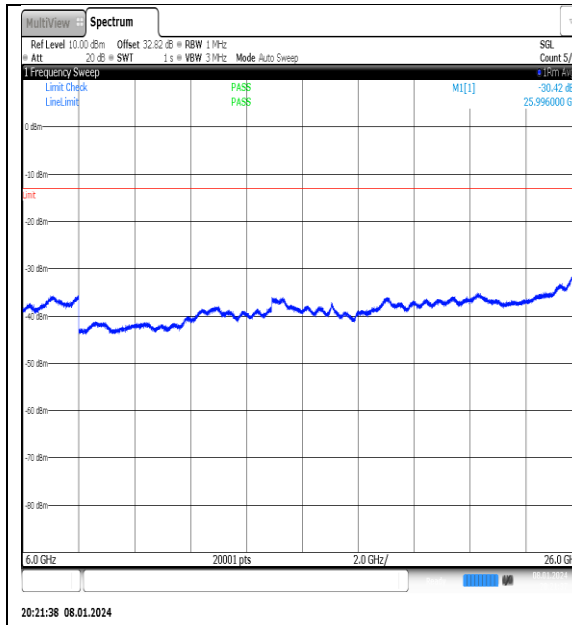
NTNV_N77-3700- 3980_PC2_30_40_L_TID6_NS_01_6000_26000_ #1
