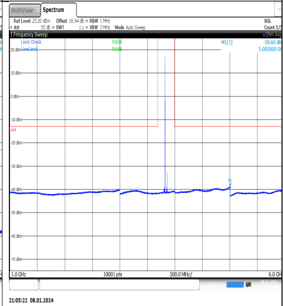
NTNV_N77-3700- 3980_PC2_30_40_M_TID5_NS_01_1000_6000_# 1
