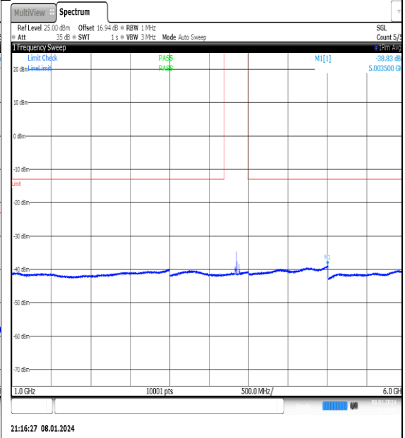
NTNV_N77-3700- 3980_PC2_30_40_M_TID9_NS_01_1000_6000_# 1
