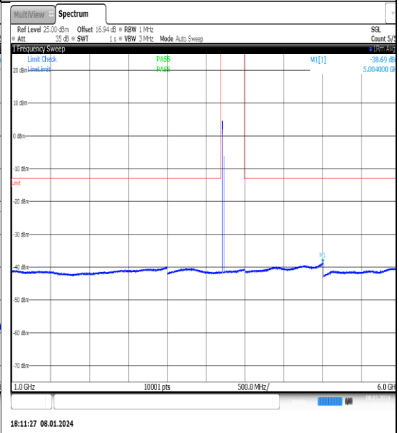
NTN_V_N77-3700- 3980_PC2_30_30_L_TID13_NS_01_1000_6000_ #1
