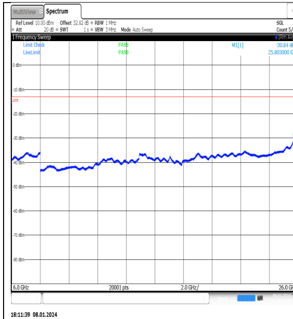
NTNV_N77-3700- 3980_PC2_30_30_L_TID13_NS_01_6000_26000 _#1
