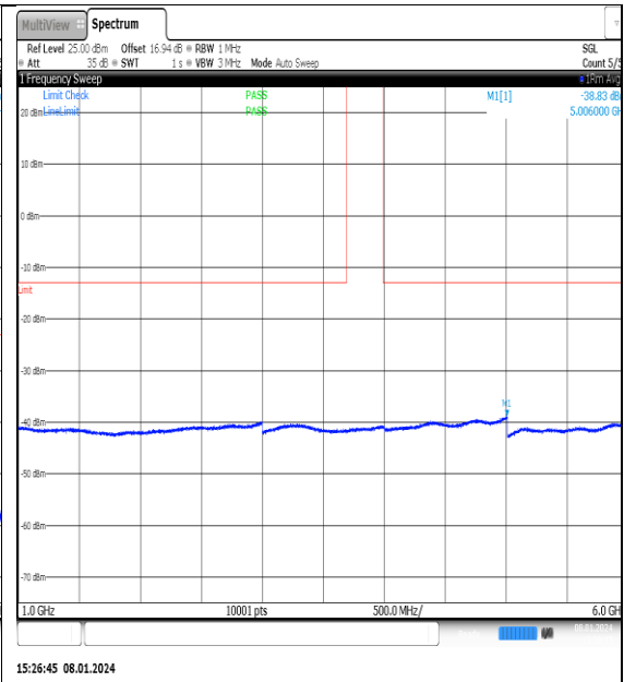
NTNV_N77-3700- 3980_PC2_30_25_H_TID13_NS_01_1000_6000_#1
