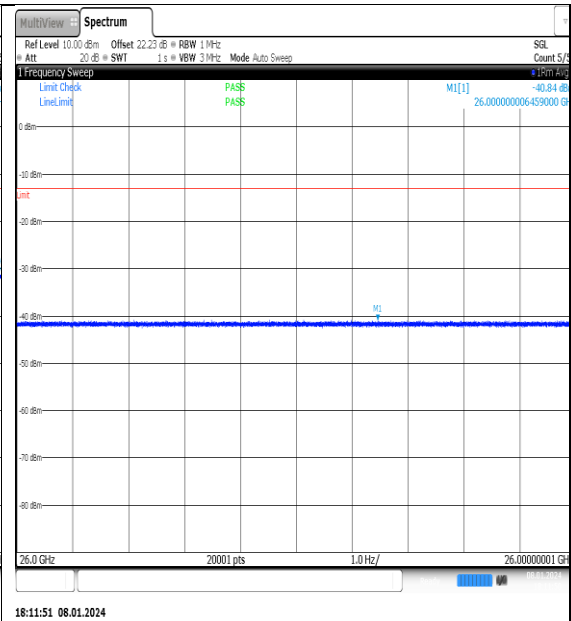
NTNV_N77-3700- 3980_PC2_30_30_L_TID13_NS_01_26000_4000 0_#1
