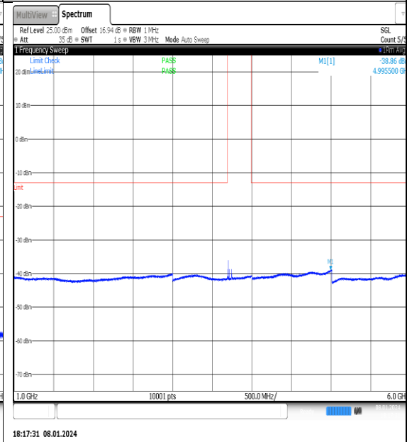
NTN_V_N77-3700- 3980_PC2_30_30_L_TID15_NS_01_1000_6000_ #1
