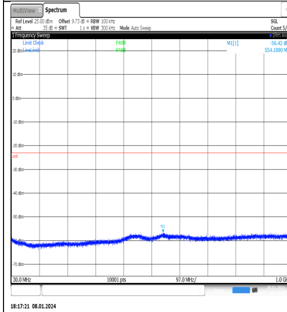
NTN_V_N77-3700- 3980_PC2_30_30_L_TID15_NS_01_30_1000_#1
