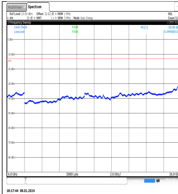
NTNV_N77-3700- 3980_PC2_30_30_L_TID15_NS_01_6000_26000 _#1
