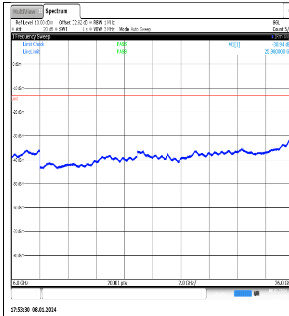
NTNV_N77-3700- 3980_PC2_30_30_L_TID7_NS_01_6000_26000_ #1
