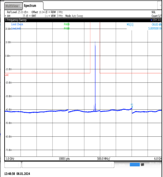
NTNV_N77-3700- 3980_PC2_30_25_M_TID7_NS_01_1000_6000_# 1
