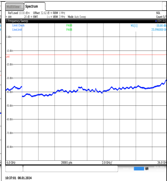
NTN_V_N77-3700- 3980_PC2_30_25_L_TID14_NS_01_6000_26000_ #1
