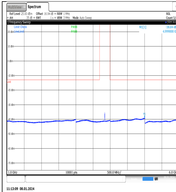
NTNV_N77-3700- 3980_PC2_30_25_M_TID5_NS_01_1000_6000_# 1
