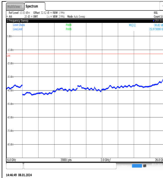
NTNV_N77-3700- 3980_PC2_30_25_H_TID6_NS_01_6000_26000_#1
