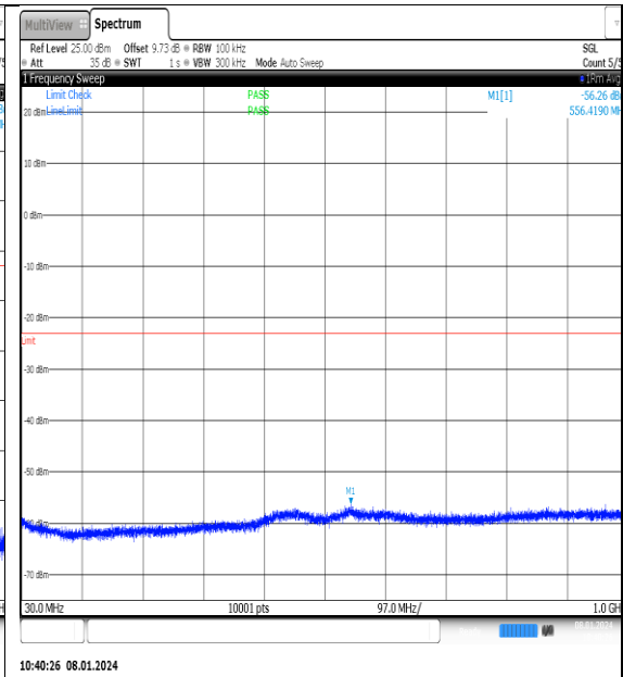
NTNV_N77-3700- 3980_PC2_30_25_L_TID15_NS_01_30_1000_#1
