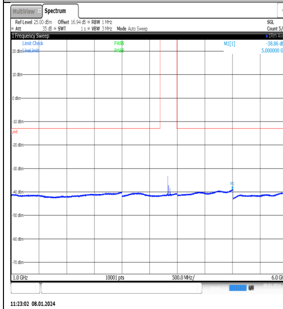
NTNV_N77-3700-3980_PC2_30_25_M_TID6_NS_01_1000_6000_#1
