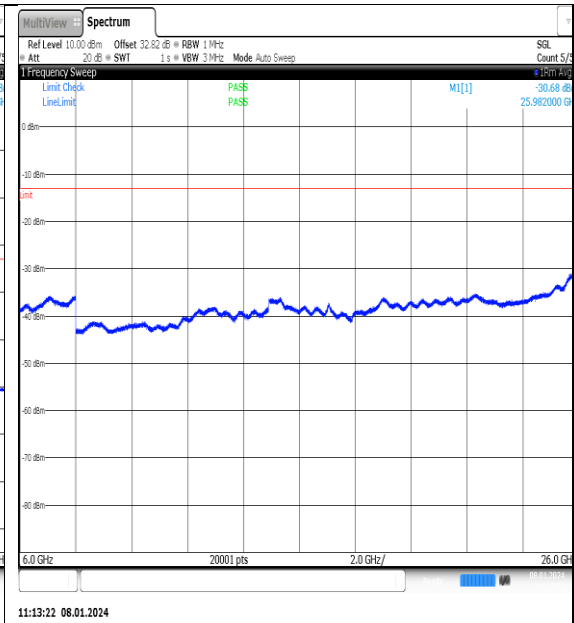
NTNV_N77-3700- 3980_PC2_30_25_M_TID5_NS_01_6000_26000_# 1
