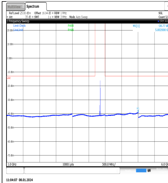
NTN_V_N77-3700- 3980_PC2_30_25_M_TID3_NS_01_1000_6000_# 1
