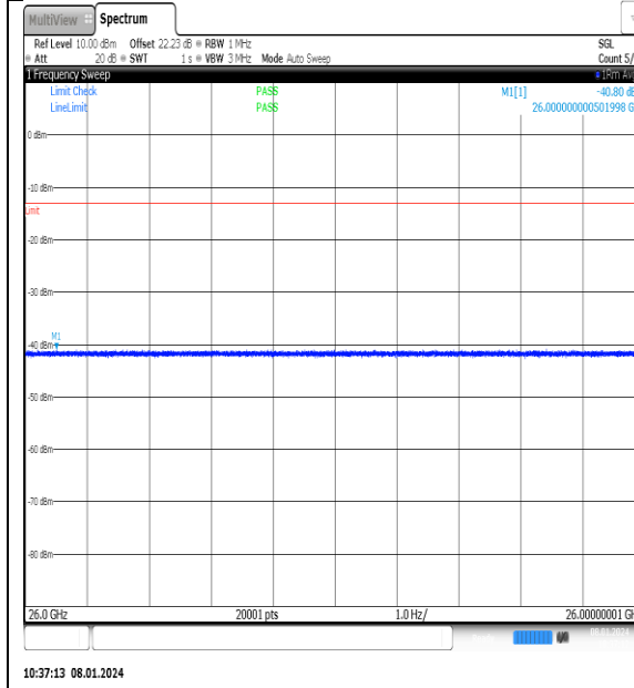
NTN_V_N77-3700- 3980_PC2_30_25_L_TID14_NS_01_26000_4000_ 0_#1
