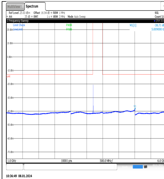
NTN_V_N77-3700- 3980_PC2_30_25_L_TID14_NS_01_1000_6000_ #1
