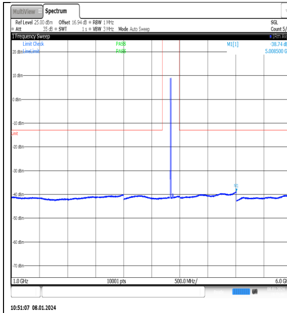
NTN_V_N77-3700- 3980_PC2_30_25_M_TID1_NS_01_1000_6000_# 1
