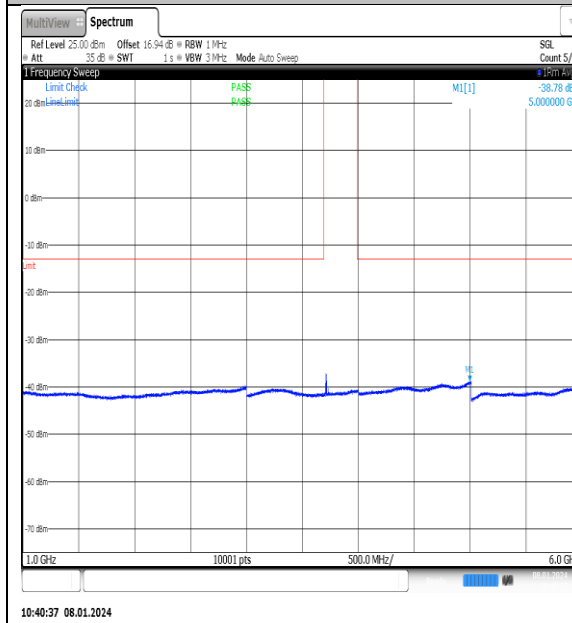
NTNV_N77-3700- 3980_PC2_30_25_L_TID15_NS_01_1000_6000_#1
