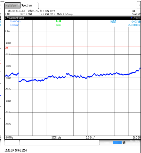
NTN_V_N77-3700- 3980_PC2_30_25_M_TID1_NS_01_6000_26000_# #1
