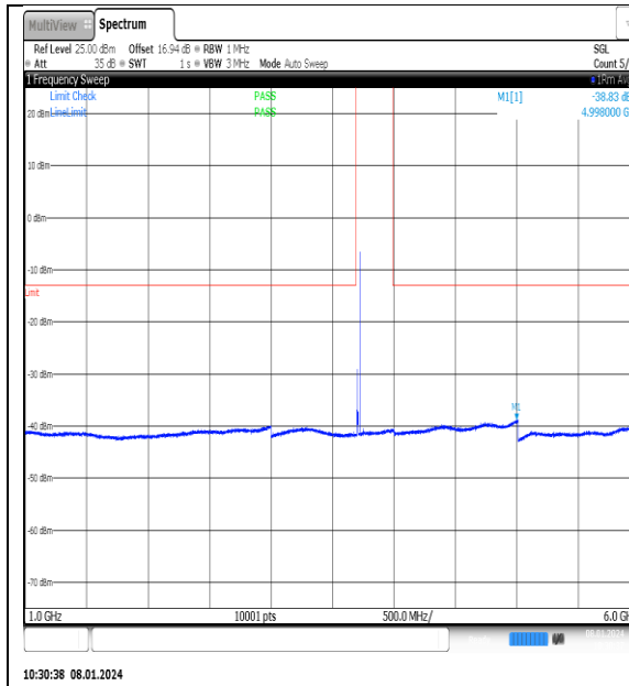
NTN_V_N77-3700- 3980_PC2_30_25_L_TID12_NS_01_1000_6000_ #1
