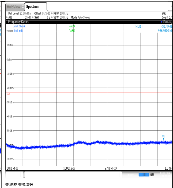
NTNV_N77-3700- 3980_PC2_30_25_L_TID5_NS_01_30_1000_#1
