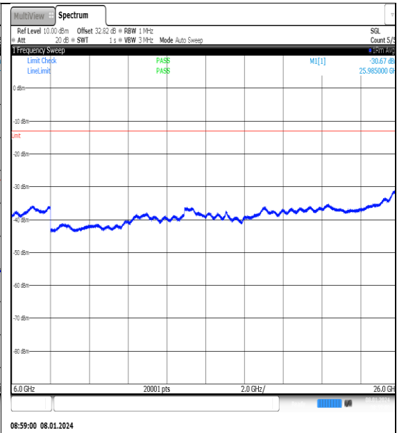
NTN_V_N77-3700- 3980_PC2_30_20_H_TID3_NS_01_6000_26000_# #1
