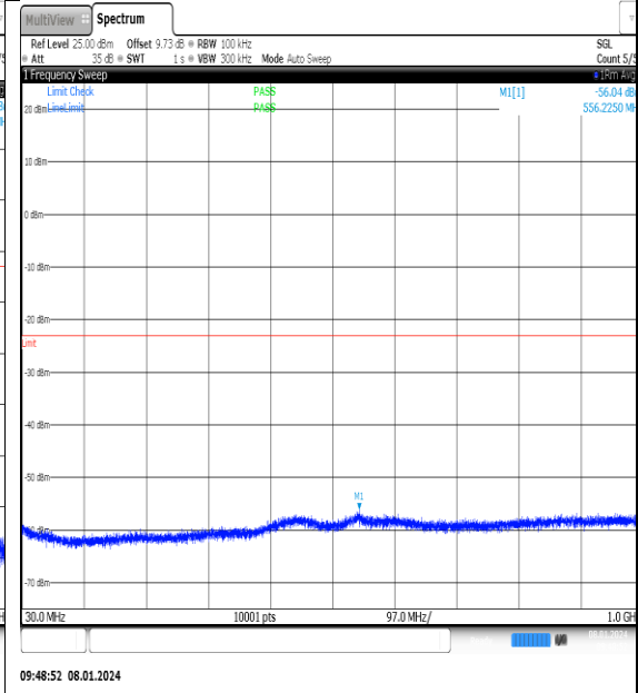
NTNV_N77-3700- 3980_PC2_30_25_L_TID2_NS_01_30_1000_#1
