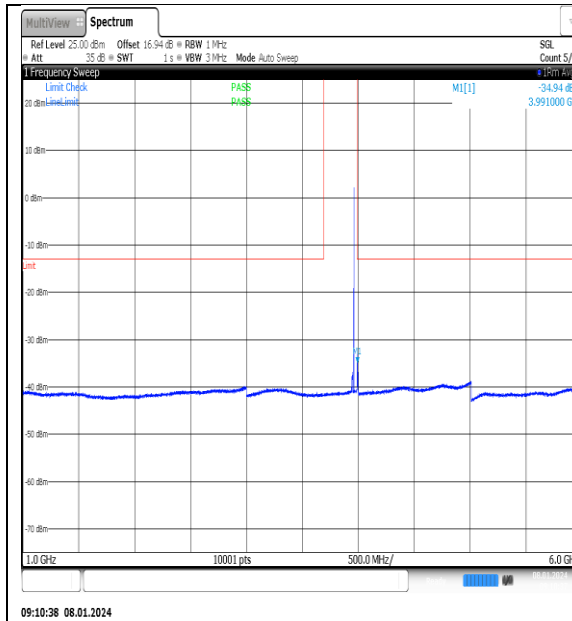
NTN_V_N77-3700- 3980_PC2_30_20_H_TID7_NS_01_1000_6000_# 1
