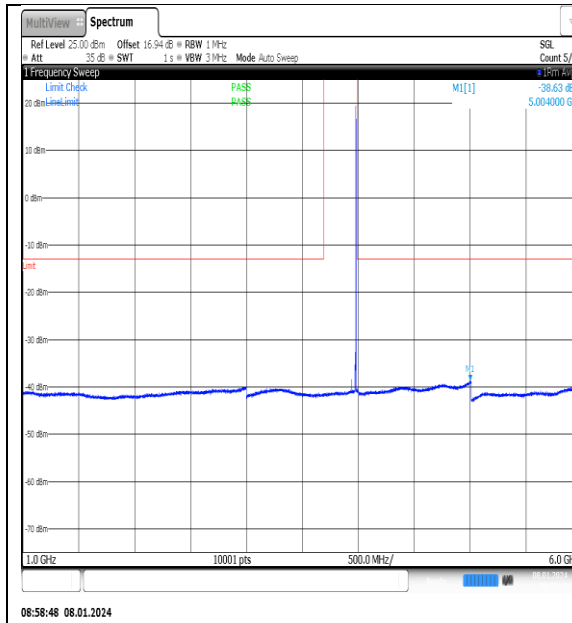
NTN_V_N77-3700- 3980_PC2_30_20_H_TID3_NS_01_1000_6000_# 1
