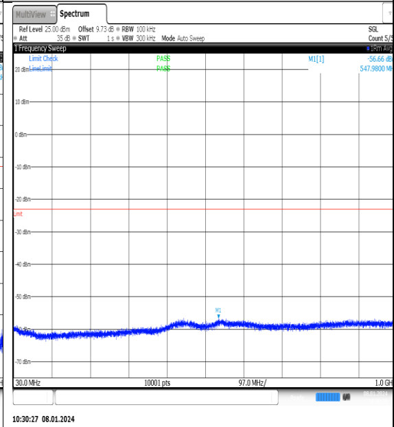
NTNV_N77-3700- 3980_PC2_30_25_L_TID12_NS_01_30_1000_#1
