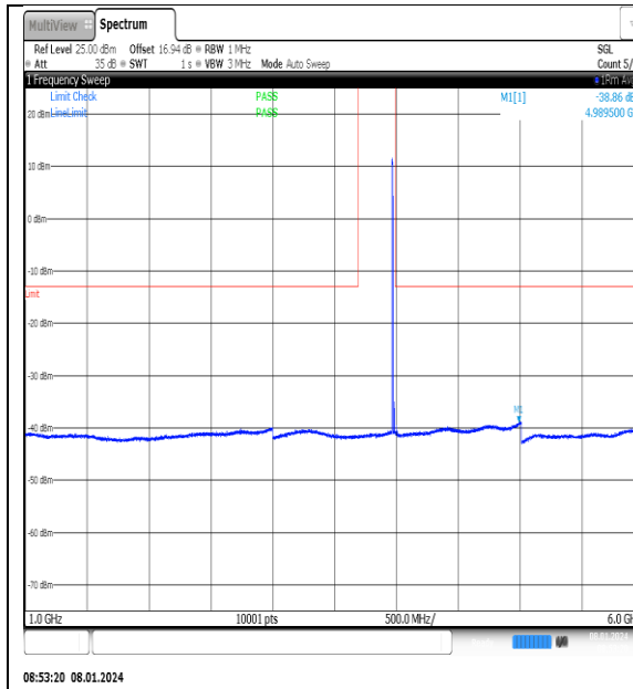
NTN_V_N77-3700- 3980_PC2_30_20_H_TID1_NS_01_1000_6000_# 1
