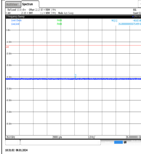
NTN_V_N77-3700- 3980_PC2_30_25_L_TID12_NS_01_26000_4000 0_#1
