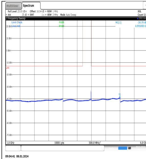
NTNV_N77-3700- 3980_PC2_30_20_H_TID5_NS_01_1000_6000_# 1
