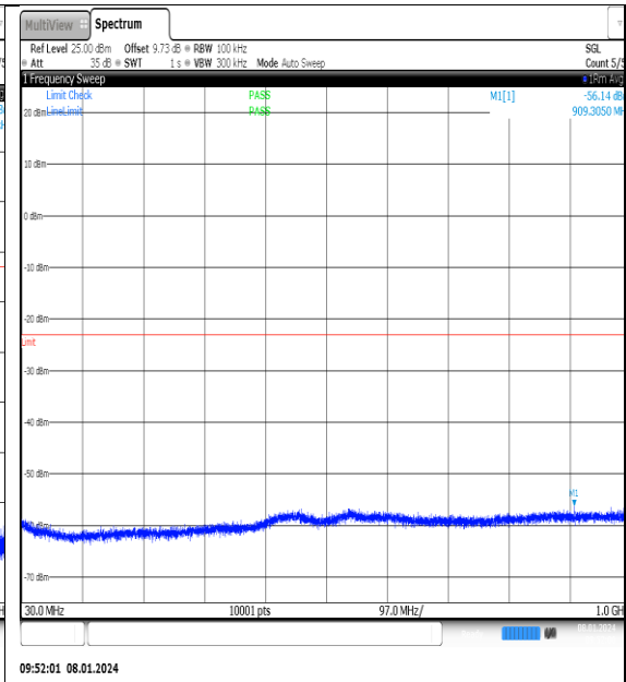
NTNV_N77-3700- 3980_PC2_30_25_L_TID3_NS_01_30_1000_#1
