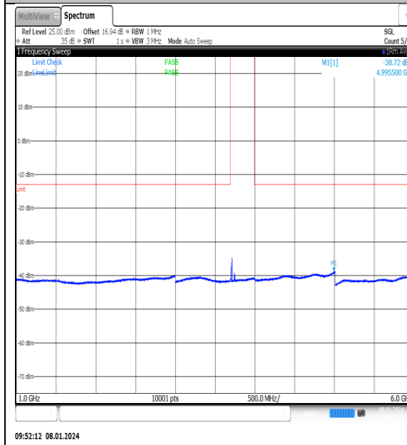
NTNV_N77-3700- 3980_PC2_30_25_L_TID3_NS_01_1000_6000_#1
