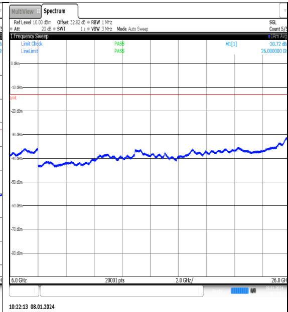
NTN_V_N77-3700- 3980_PC2_30_25_L_TID10_NS_01_6000_26000 #1
