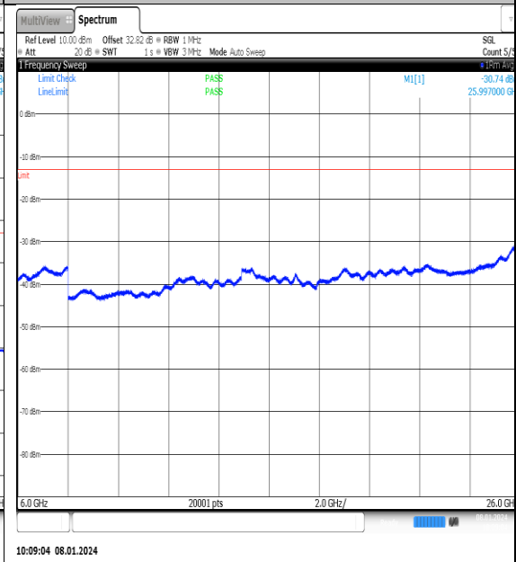
NTNV_N77-3700- 3980_PC2_30_25_L_TID7_NS_01_6000_26000_#1
