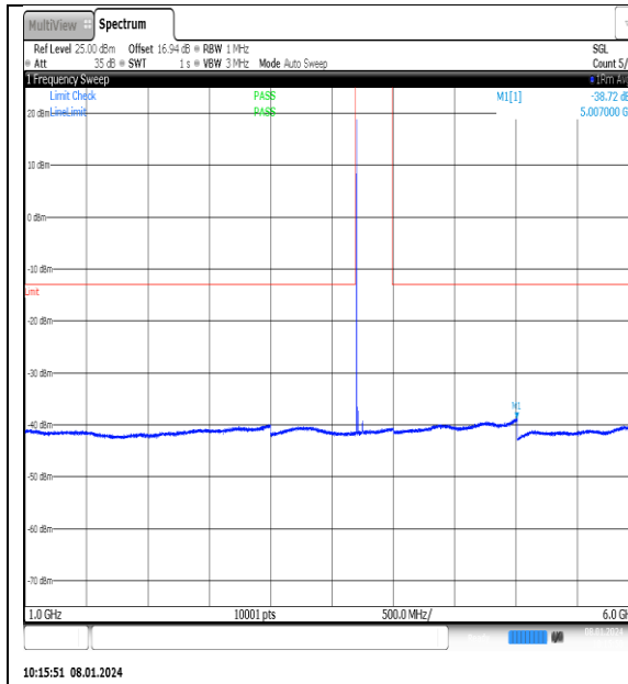
NTN_V_N77-3700- 3980_PC2_30_25_L_TID8_NS_01_1000_6000_# 1
