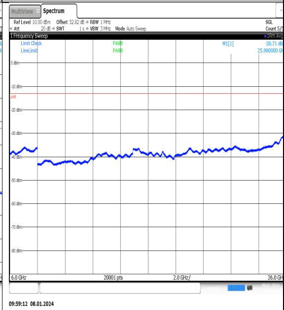
NTNV_N77-3700- 3980_PC2_30_25_L_TID5_NS_01_6000_26000_#1
