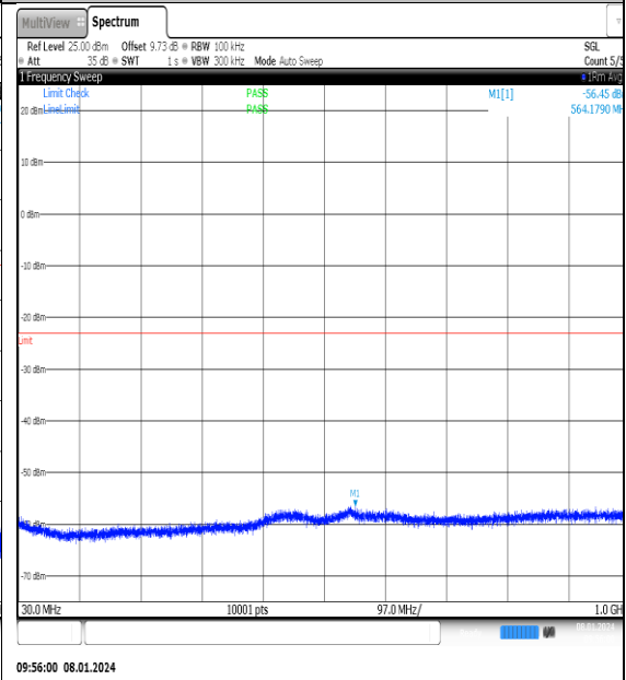
NTNV_N77-3700- 3980_PC2_30_25_L_TID4_NS_01_30_1000_#1
