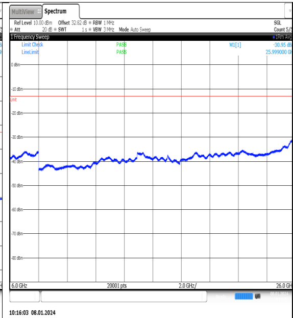
NTN_V_N77-3700- 3980_PC2_30_25_L_TID8_NS_01_6000_26000_# #1
