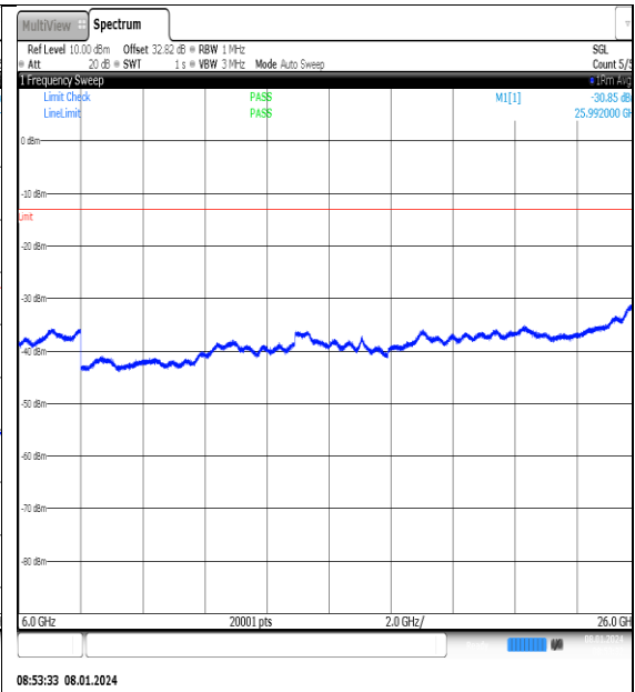
NTN_V_N77-3700- 3980_PC2_30_20_H_TID1_NS_01_6000_26000_# #1
