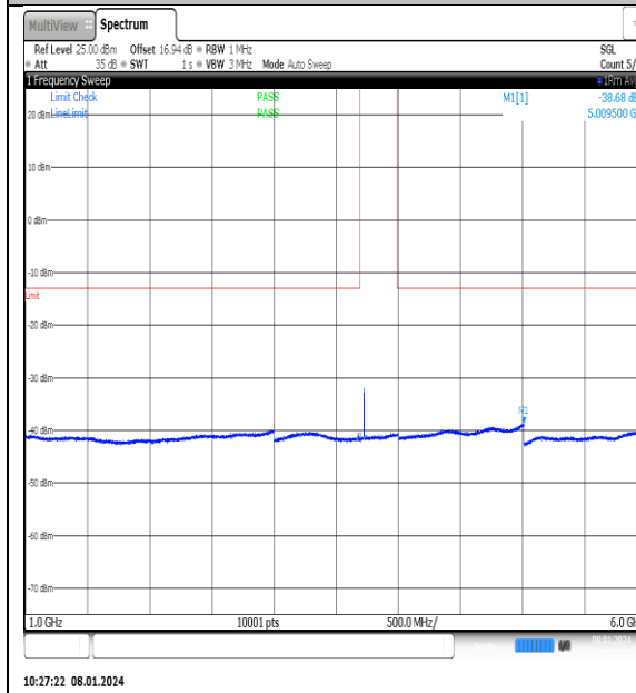
NTNV_N77-3700- 3980_PC2_30_25_L_TID11_NS_01_1000_6000_#1
