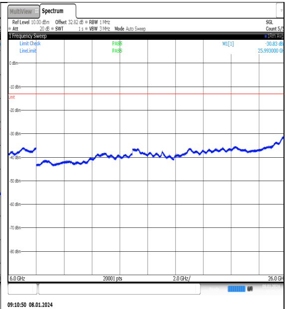
NTN_V_N77-3700- 3980_PC2_30_20_H_TID7_NS_01_6000_26000_# #1
