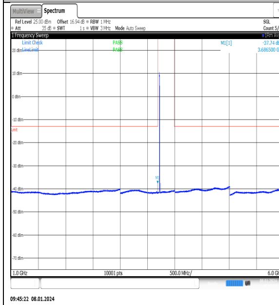
NTNV_N77-3700- 3980_PC2_30_25_L_TID1_NS_01_1000_6000_#
