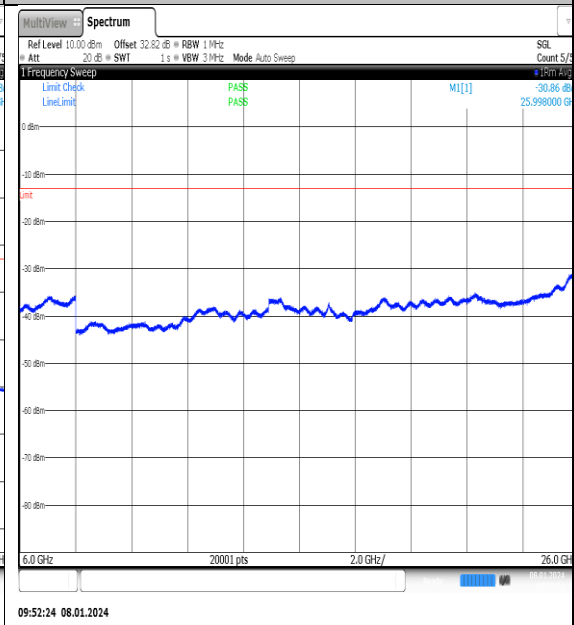
NTNV_N77-3700- 3980_PC2_30_25_L_TID3_NS_01_6000_26000_#1
