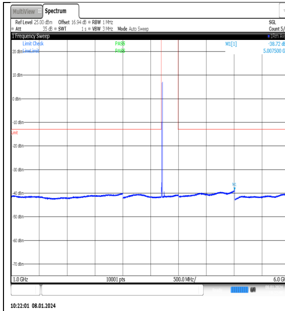
NTN_V_N77-3700- 3980_PC2_30_25_L_TID10_NS_01_1000_6000_ #1
