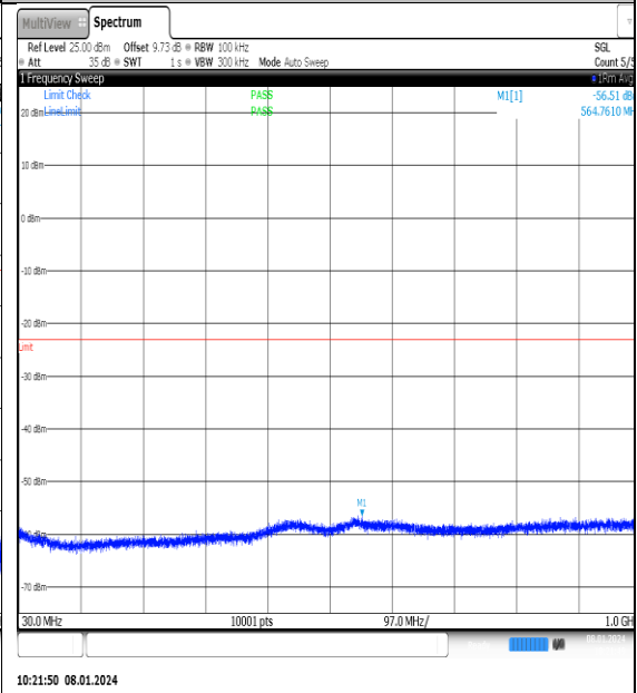
NTNV_N77-3700- 3980_PC2_30_25_L_TID10_NS_01_30_1000_#1
