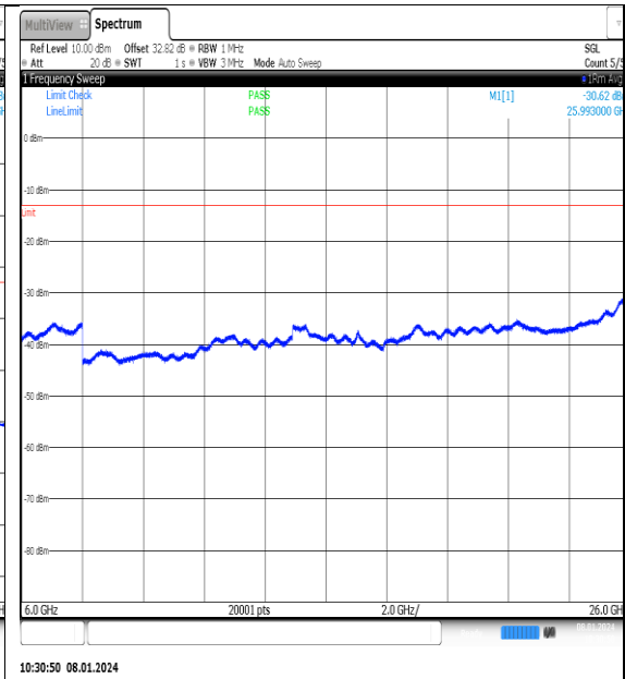
NTN_V_N77-3700- 3980_PC2_30_25_L_TID12_NS_01_6000_26000 #1
