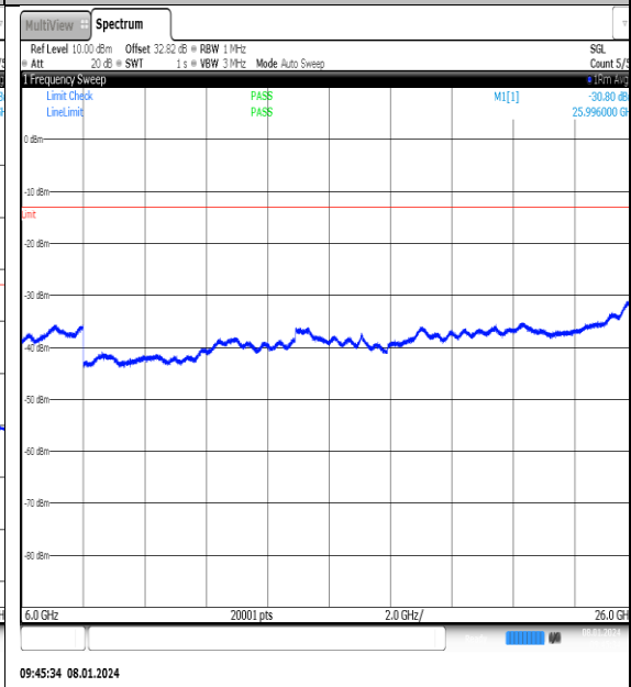
NTNV_N77-3700- 3980_PC2_30_25_L_TID1_NS_01_6000_26000_#1
