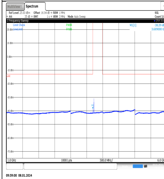
NTNV_N77-3700- 3980_PC2_30_25_L_TID5_NS_01_1000_6000_#
