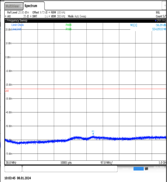
NTNV_N77-3700- 3980_PC2_30_25_L_TID6_NS_01_30_1000_#1
