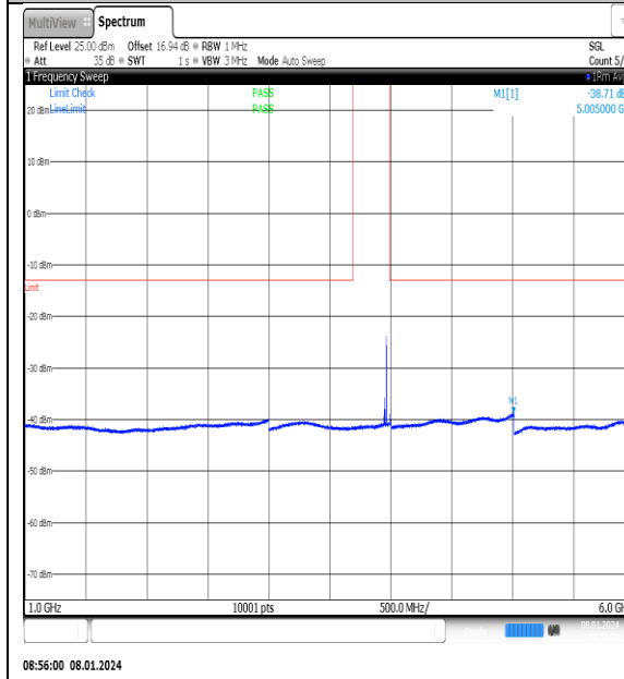
NTNV_N77-3700- 3980_PC2_30_20_H_TID2_NS_01_1000_6000_#1
