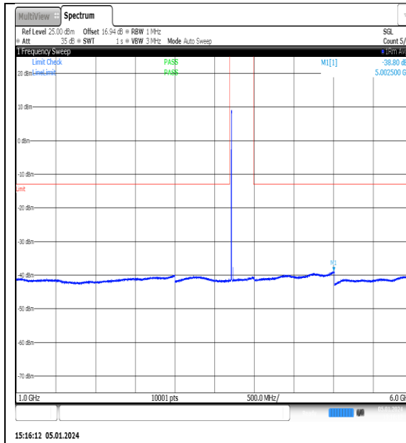
NTN V _N77-3700- 3980_PC2_30_20_L_TID7_NS_01_1000_6000_# 1
