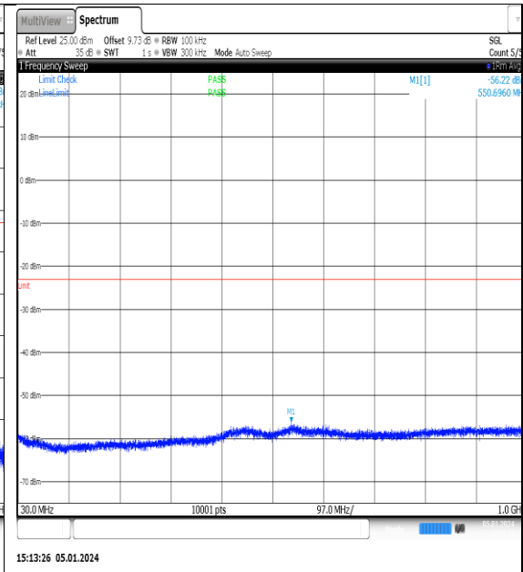
NTNV_N77-3700- 3980_PC2_30_20_L_TID6_NS_01_30_1000_#1
