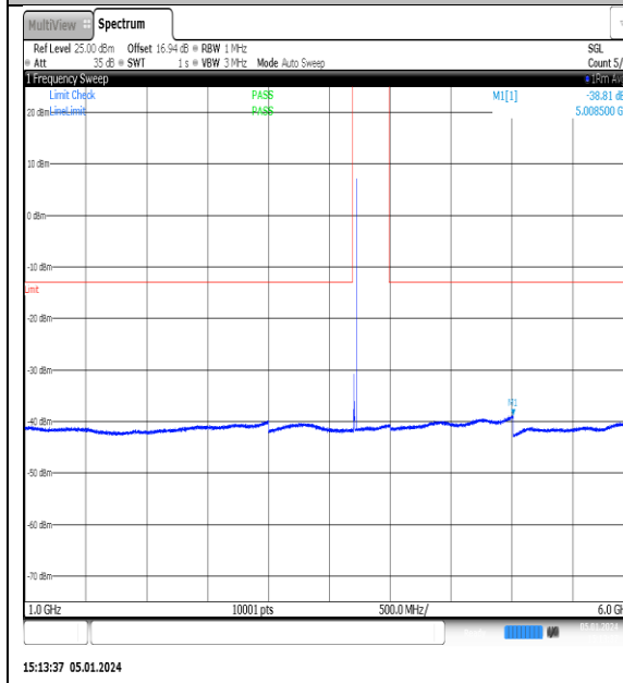
NTNV_N77-3700- 3980_PC2_30_20_L_TID6_NS_01_1000_6000_#1
