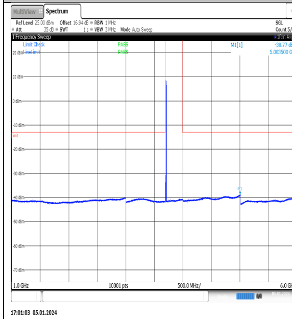
NTNV_N77-3700-3980_PC2_30_20_L_TID10_NS_01_1000_6000_#1
