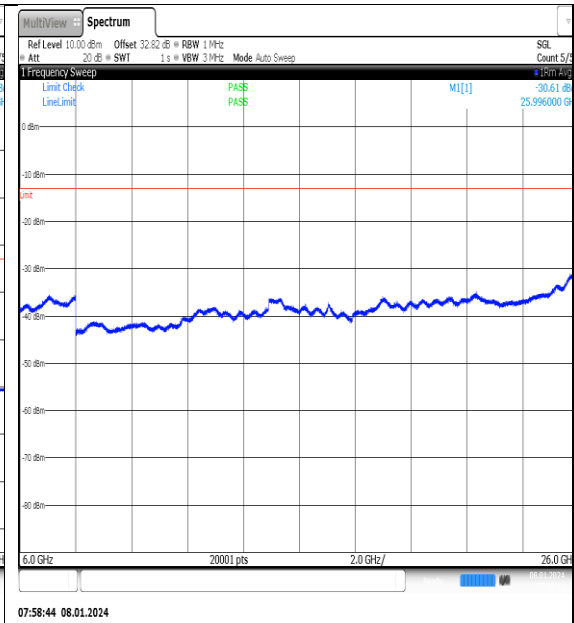
NTN_V_N77-3700- 3980_PC2_30_20_L_TID15_NS_01_6000_26000 #1
