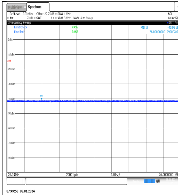
NTNV_N77-3700- 3980_PC2_30_20_L_TID12_NS_01_26000_4000 0_#1
