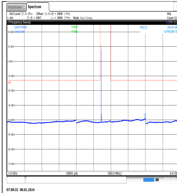
NTN_V_N77-3700- 3980_PC2_30_20_L_TID15_NS_01_1000_6000_ #1
