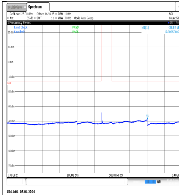
NTNV_N77-3700- 3980_PC2_30_20_L_TID5_NS_01_1000_6000_# 1
