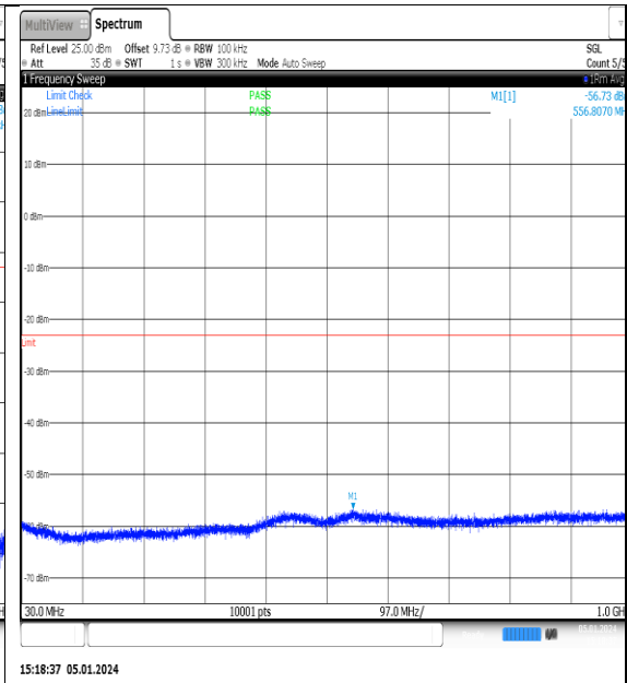
NTNV_N77-3700-3980_PC2_30_20_L_TID8_NS_01_30_1000_#1
