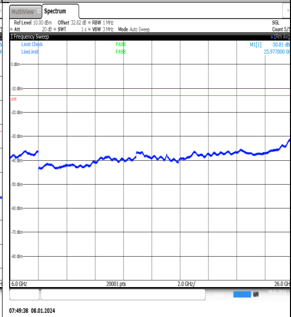
NTNV_N77-3700- 3980_PC2_30_20_L_TID12_NS_01_6000_26000_#1
