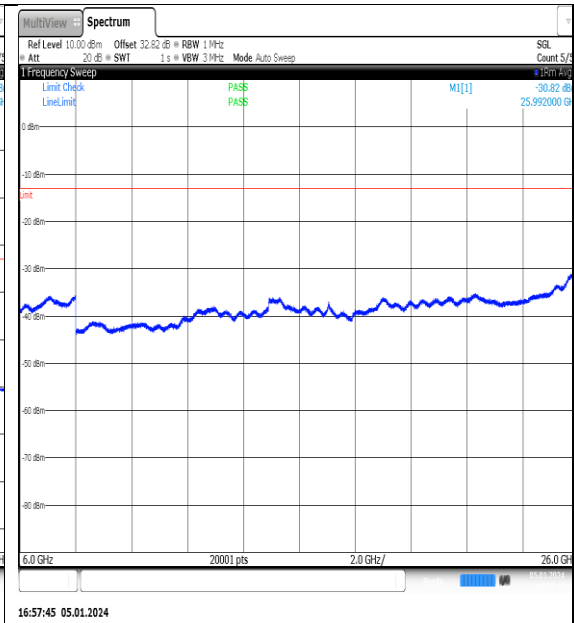
NTN_V_N77-3700- 3980_PC2_30_20_L_TID9_NS_01_6000_26000_# #1
