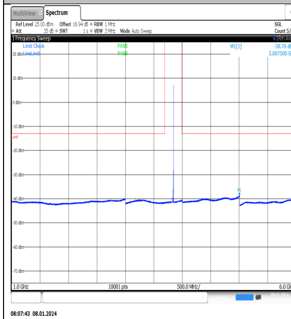
NTNV_N77-3700- 3980_PC2_30_20_M_TID3_NS_01_1000_6000_# 1
