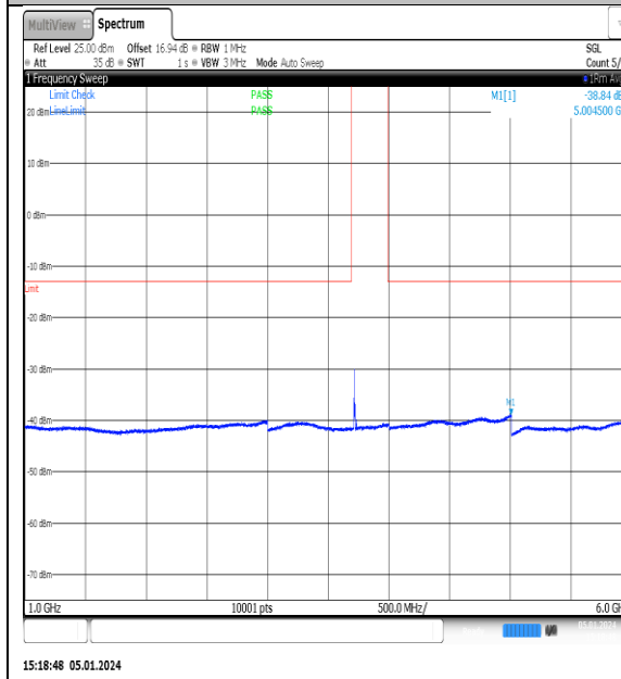
NTNV_N77-3700-3980_PC2_30_20_L_TID8_NS_01_1000_6000_#1
