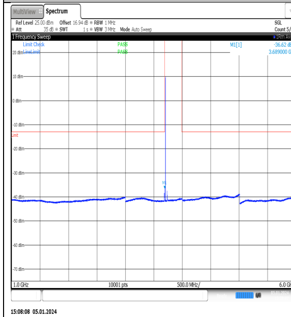
NTNV_N77-3700- 3980_PC2_30_20_L_TID4_NS_01_1000_6000_# 1
