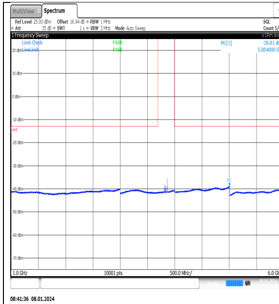
NTN_V_N77-3700- 3980_PC2_30_20_M_TID12_NS_01_1000_6000_ #1
