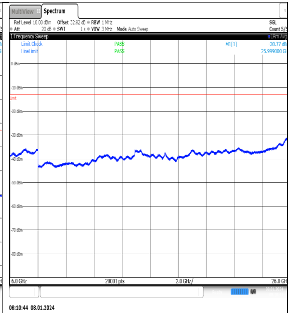
NTN_V_N77-3700- 3980_PC2_30_20_M_TID4_NS_01_6000_26000_# #1
