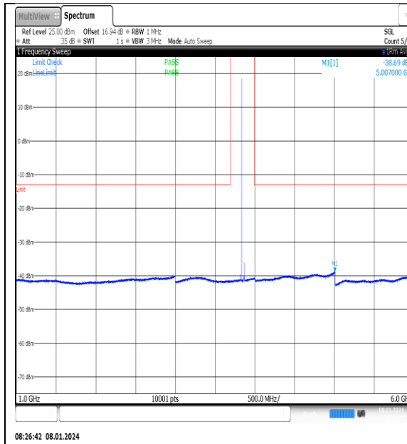
NTN_V_N77-3700- 3980_PC2_30_20_M_TID8_NS_01_1000_6000_# 1
