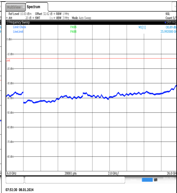
NTN_V_N77-3700- 3980_PC2_30_20_L_TID13_NS_01_6000_26000_ #1
