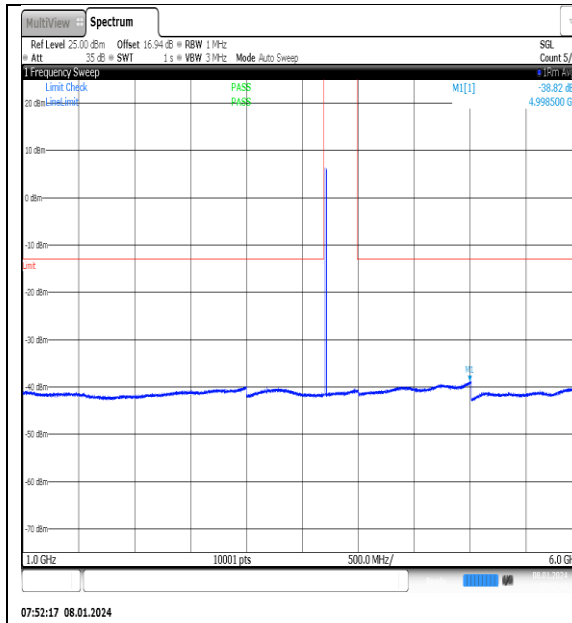
NTN_V_N77-3700- 3980_PC2_30_20_L_TID13_NS_01_1000_6000_ #1
