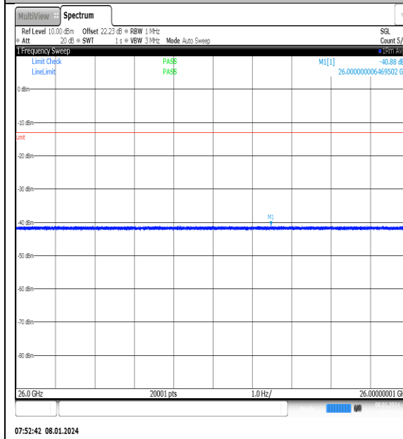
NTN_V_N77-3700- 3980_PC2_30_20_L_TID13_NS_01_26000_4000_ 0_#1
