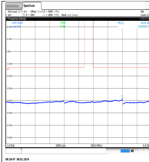
NTNV_N77-3700- 3980_PC2_30_20_M_TID6_NS_01_1000_6000_# 1
