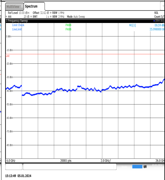
NTNV_N77-3700- 3980_PC2_30_20_L_TID6_NS_01_6000_26000_#1
