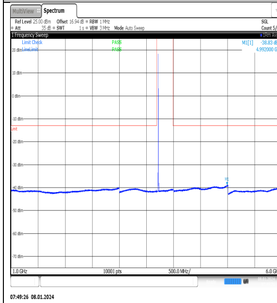
NTNV_N77-3700- 3980_PC2_30_20_L_TID12_NS_01_1000_6000_#1
