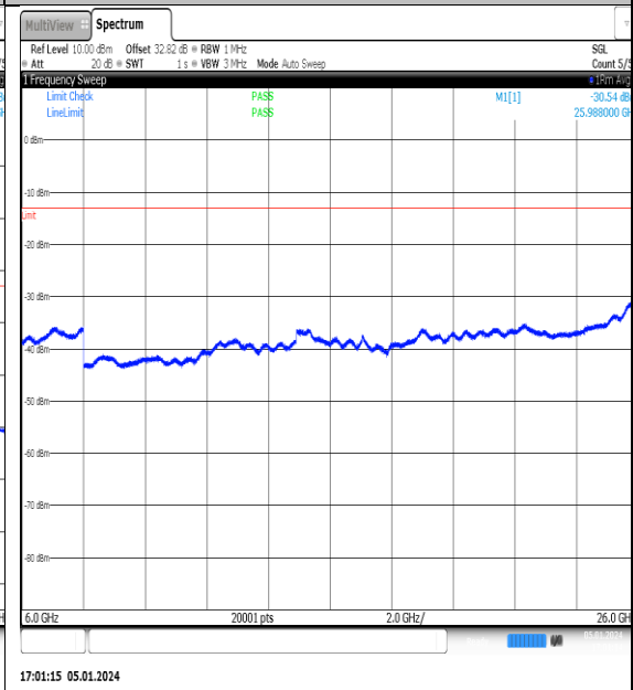
NTNV_N77-3700-3980_PC2_30_20_L_TID10_NS_01_6000_26000_#1
