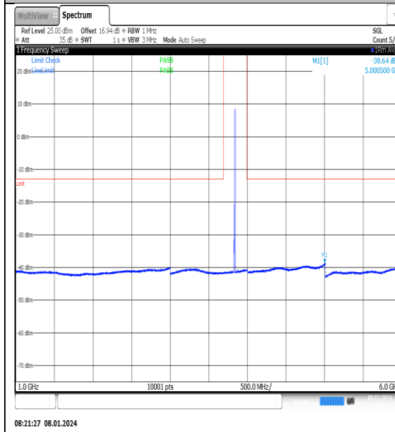
NTNV_N77-3700- 3980_PC2_30_20_M_TID7_NS_01_1000_6000_#1
