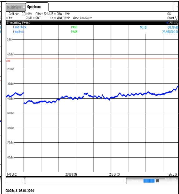
NTN_V_N77-3700- 3980_PC2_30_20_M_TID2_NS_01_6000_26000_# #1
