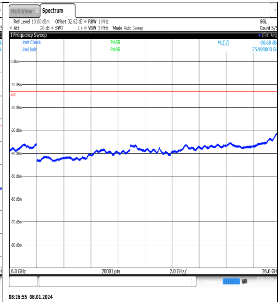
NTN_V_N77-3700- 3980_PC2_30_20_M_TID8_NS_01_6000_26000_# #1
