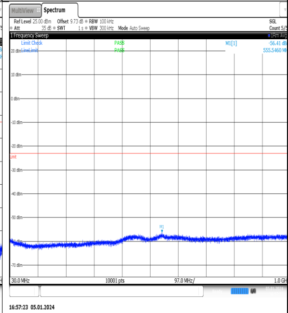
NTNV_N77-3700- 3980_PC2_30_20_L_TID9_NS_01_30_1000_#1
