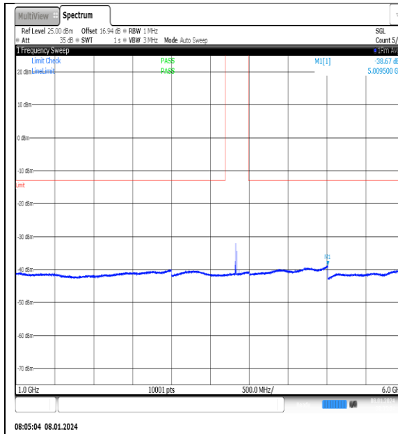
NTN_V_N77-3700- 3980_PC2_30_20_M_TID2_NS_01_1000_6000_# 1
