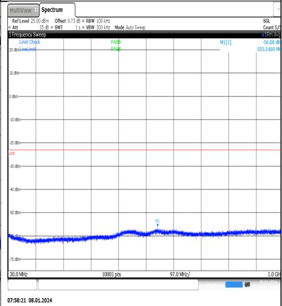
NTNV_N77-3700- 3980_PC2_30_20_L_TID15_NS_01_30_1000_#1
