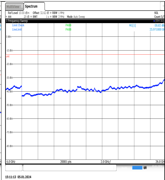
NTNV_N77-3700- 3980_PC2_30_20_L_TID5_NS_01_6000_26000_# #1
