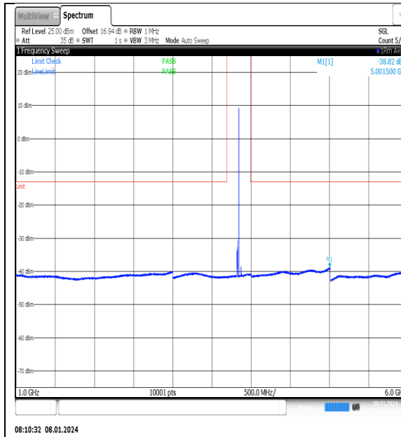
NTN_V_N77-3700- 3980_PC2_30_20_M_TID4_NS_01_1000_6000_# 1
