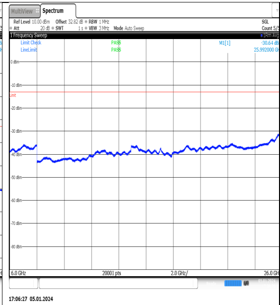
NTN_V_N77-3700- 3980_PC2_30_20_L_TID11_NS_01_6000_26000 #1
