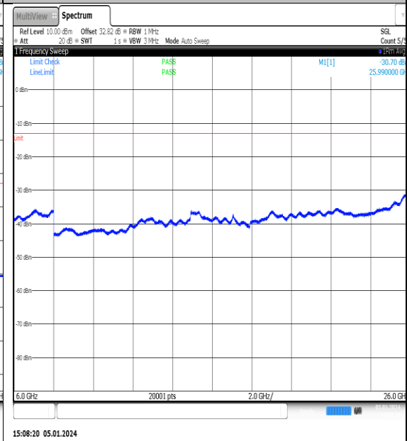
NTNV_N77-3700- 3980_PC2_30_20_L_TID4_NS_01_6000_26000_# 1
