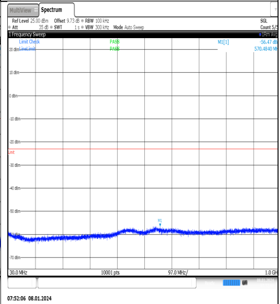
NTNV_N77-3700- 3980_PC2_30_20_L_TID13_NS_01_30_1000_#1
