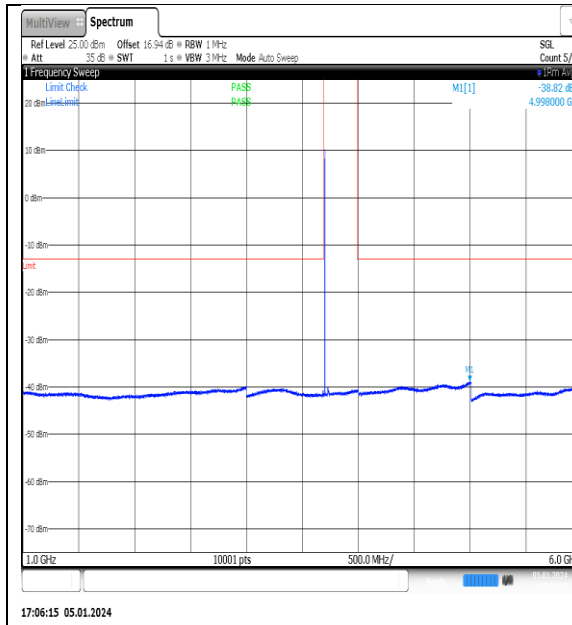
NTN_V_N77-3700- 3980_PC2_30_20_L_TID11_NS_01_1000_6000_ #1
