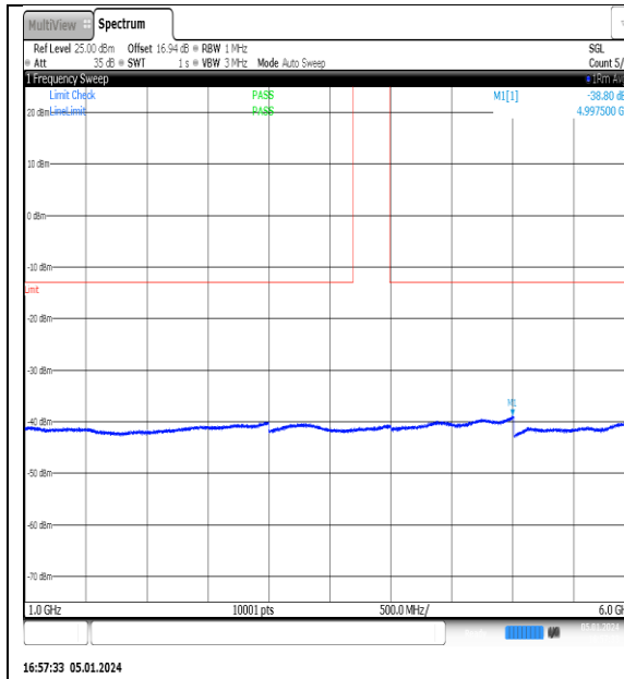
NTN_V_N77-3700- 3980_PC2_30_20_L_TID9_NS_01_1000_6000_# 1
