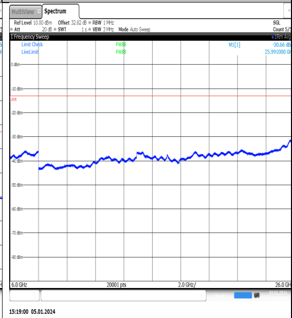
NTNV_N77-3700-3980_PC2_30_20_L_TID8_NS_01_6000_26000_#1
