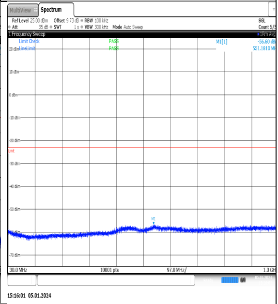
NTNV_N77-3700- 3980_PC2_30_20_L_TID7_NS_01_30_1000_#1
