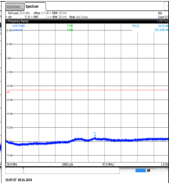
NTNV_N77-3700- 3980_PC2_30_20_L_TID4_NS_01_30_1000_#1
