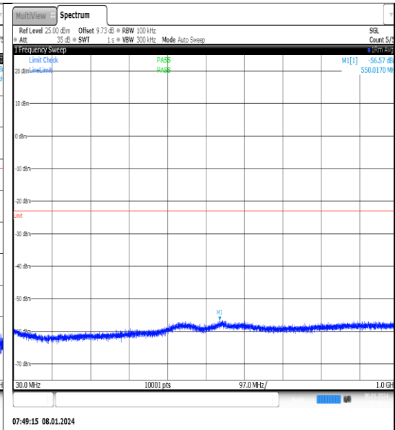
NTNV_N77-3700- 3980_PC2_30_20_L_TID12_NS_01_30_1000_#1
