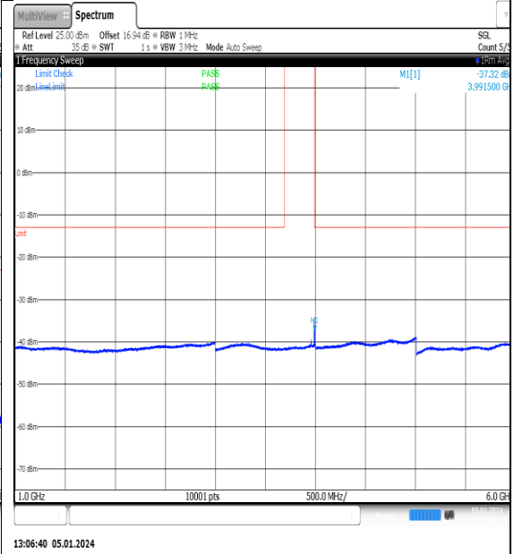
NTNV_N77-3700- 3980_PC2_30_15_H_TID3_NS_01_1000_6000_# 1
