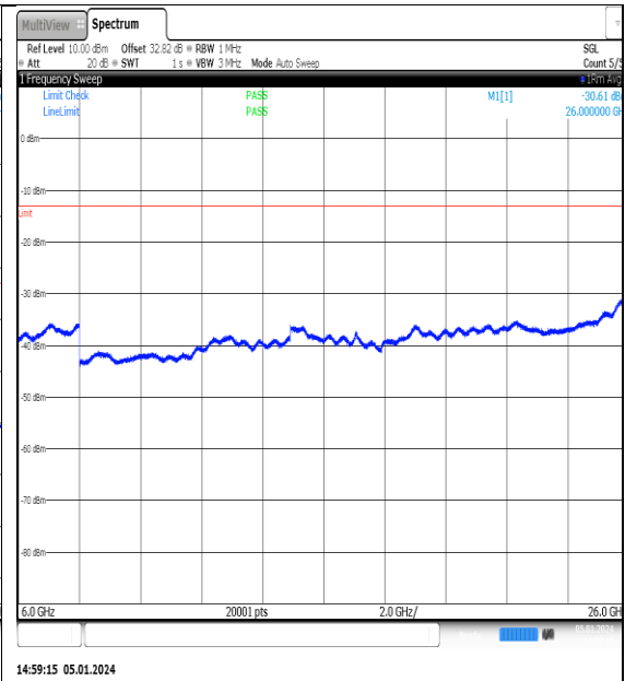
NTN_V_N77-3700- 3980_PC2_30_20_L_TID1_NS_01_6000_26000_# #1
