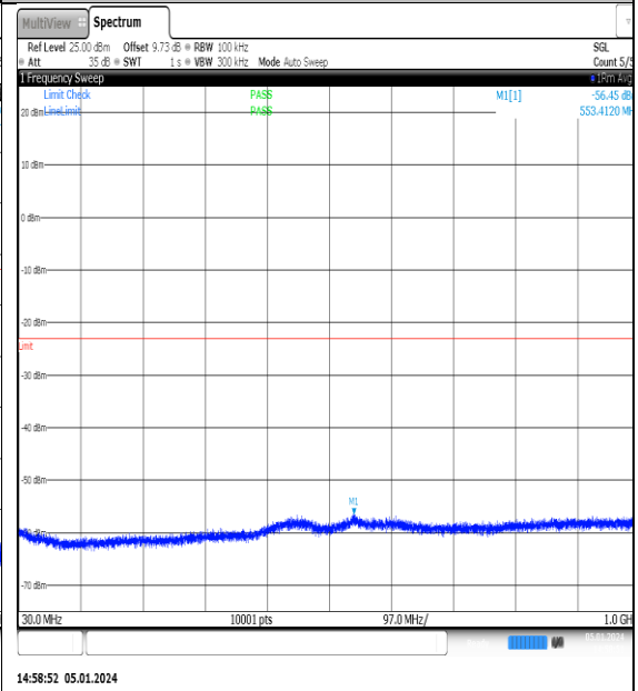
NTNV_N77-3700- 3980_PC2_30_20_L_TID1_NS_01_30_1000_#1
