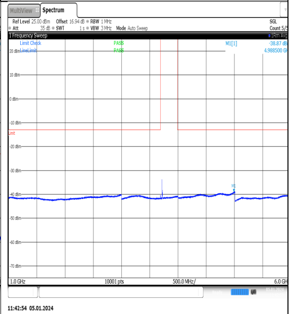
NTN_V_N77-3700- 3980_PC2_30_15_L_TID13_NS_01_1000_6000_ #1
