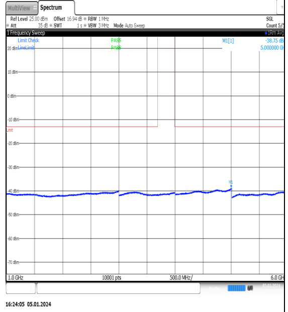
NTNV_N77-3700- 3980_PC2_30_10_M_TID3_NS_01_1000_6000_# 1
