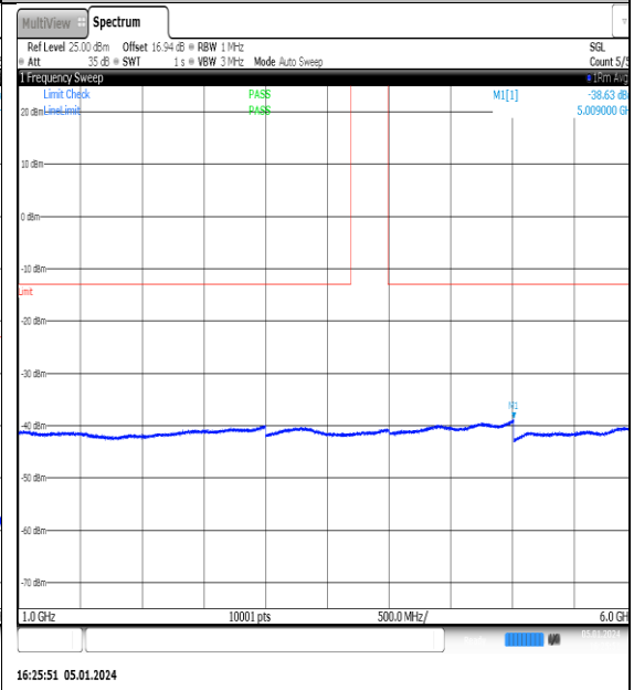
NTNV_N77-3700- 3980_PC2_30_10_M_TID5_NS_01_1000_6000_# 1
