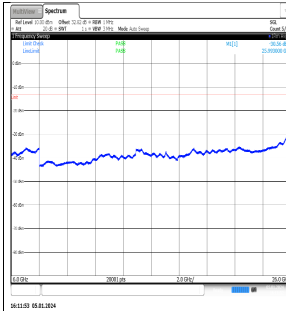
NTNV_N77-3700- 3980_PC2_30_10_L_TID4_NS_01_6000_26000_ #1
