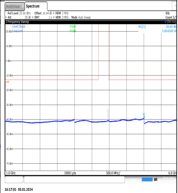
NTNV_N77-3700- 3980_PC2_30_10_L_TID10_NS_01_1000_6000_ #1
