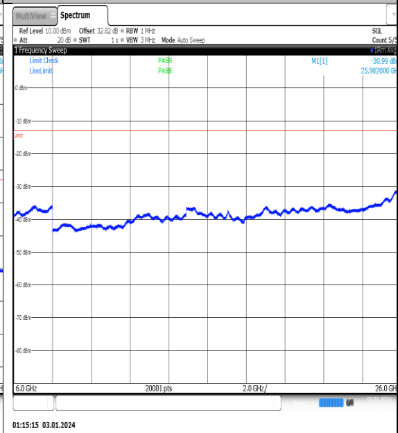
NTNV_N77-3450- 3550_PC2_30_100_M_TID12_NS_01_6000_2600 0_#1
