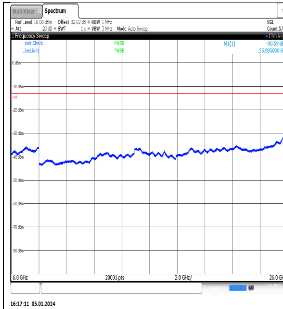
NTNV_N77-3700- 3980_PC2_30_10_L_TID10_NS_01_6000_26000 _#1
