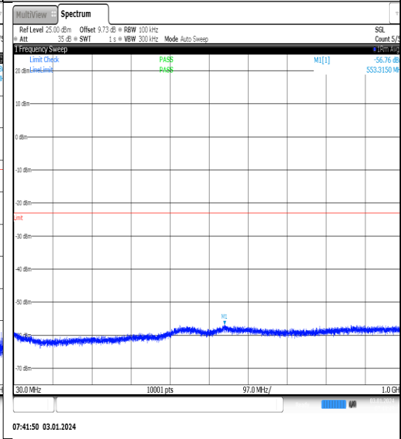
NTNV_N77-3450- 3550_PC2_30_60_L_TID1_NS_01_30_1000_#1
