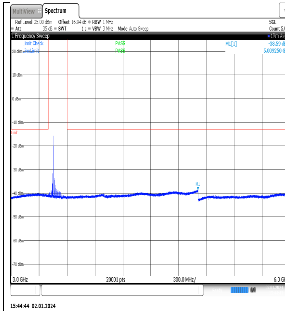
NTNV_N77-3450- 3550_PC2_30_90_L_TID8_NS_01_3000_6000_# 1
