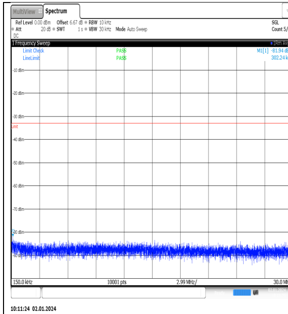
NTNV_N77-3450- 3550_PC2_30_90_L_TID2_NS_01_0.15_30_#1
