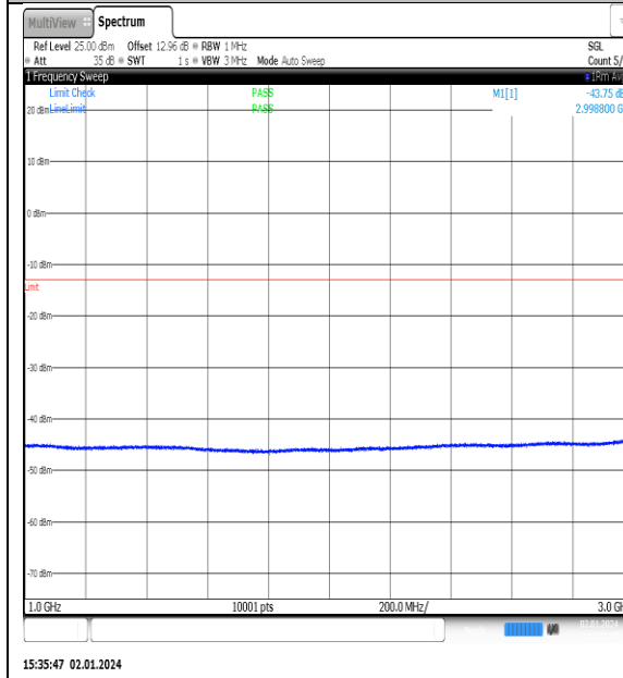
NTNV_N77-3450- 3550_PC2_30_90_L_TID5_NS_01_1000_3000_#1
