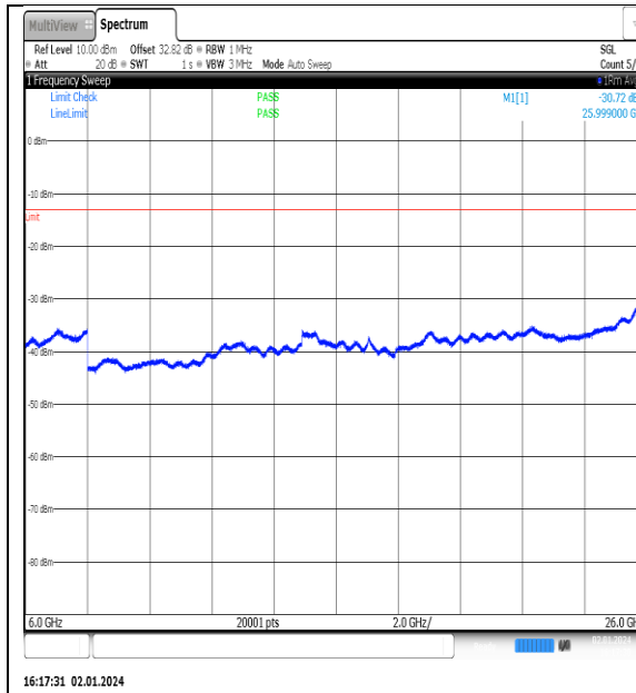
NTNV_N77-3450- 3550_PC2_30_90_M_TID2_NS_01_6000_26000_#1
