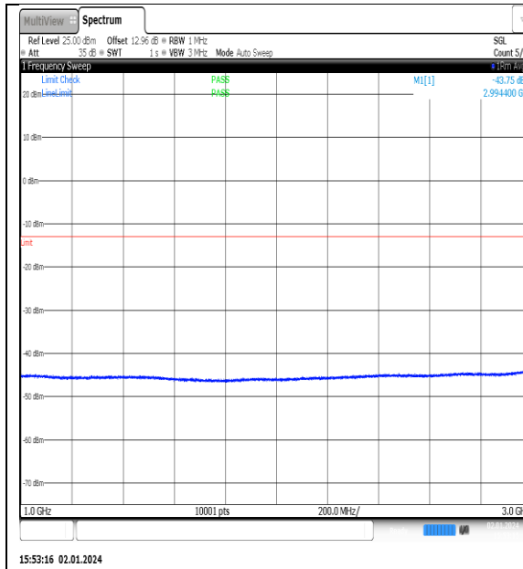
NTNV_N77-3450- 3550_PC2_30_90_L_TID11_NS_01_1000_3000_ #1
