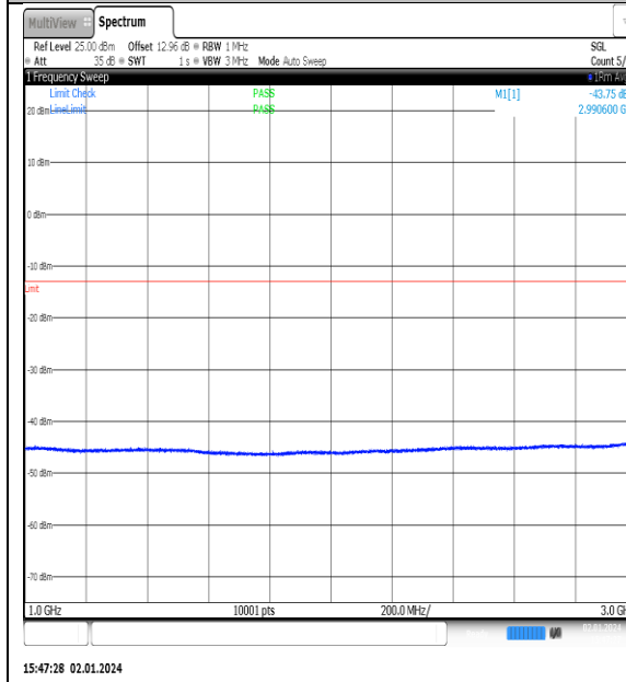
NTNV_N77-3450- 3550_PC2_30_90_L_TID9_NS_01_1000_3000_# 1
