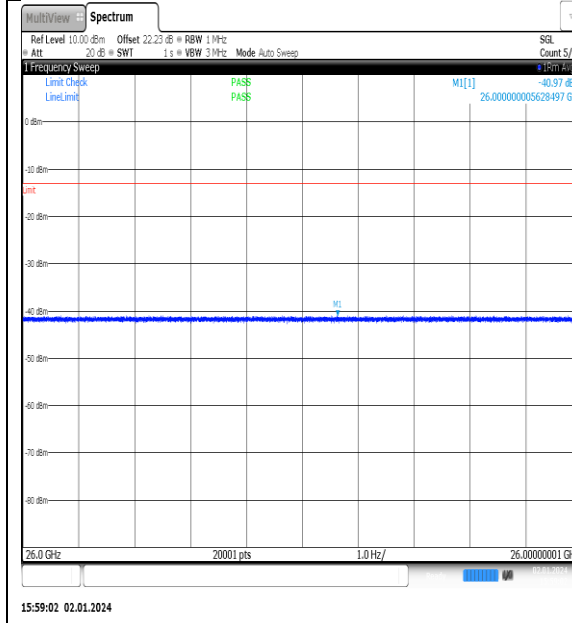
NTNV_N77-3450- 3550_PC2_30_90_L_TID12_NS_01_26000_4000_ 0_#1
