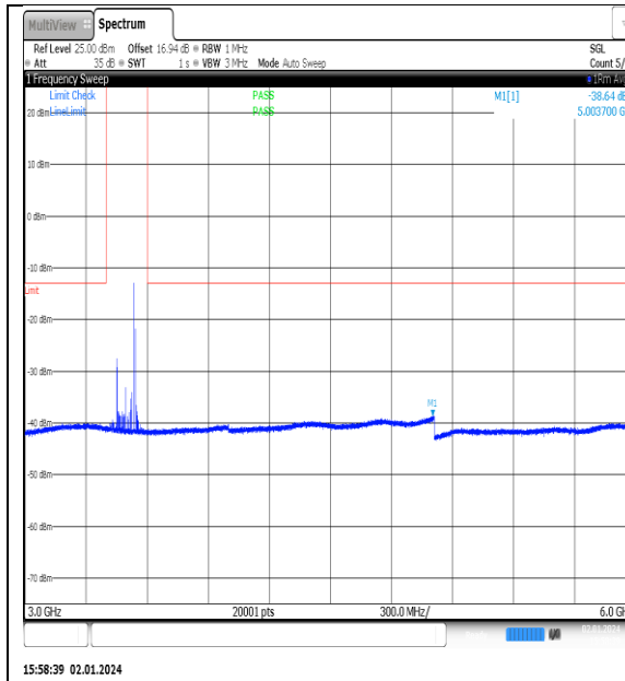
NTNV_N77-3450- 3550_PC2_30_90_L_TID12_NS_01_3000_6000_ #1
