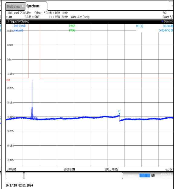
NTNV_N77-3450- 3550_PC2_30_90_M_TID2_NS_01_3000_6000_# 1
