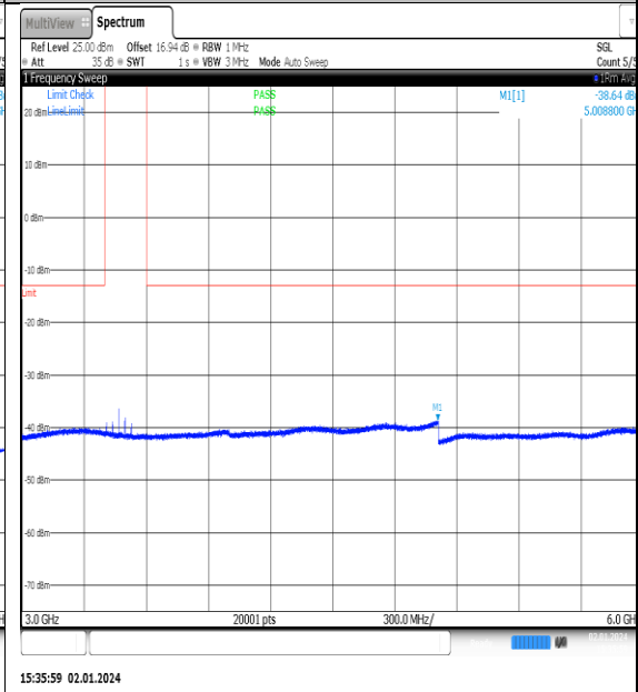
NTNV_N77-3450- 3550_PC2_30_90_L_TID5_NS_01_3000_6000_#1
