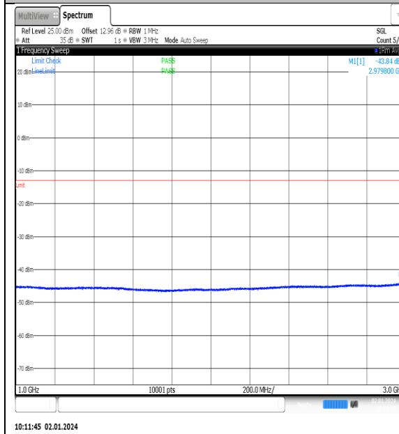
NTNV_N77-3450- 3550_PC2_30_90_L_TID2_NS_01_1000_3000_# 1
