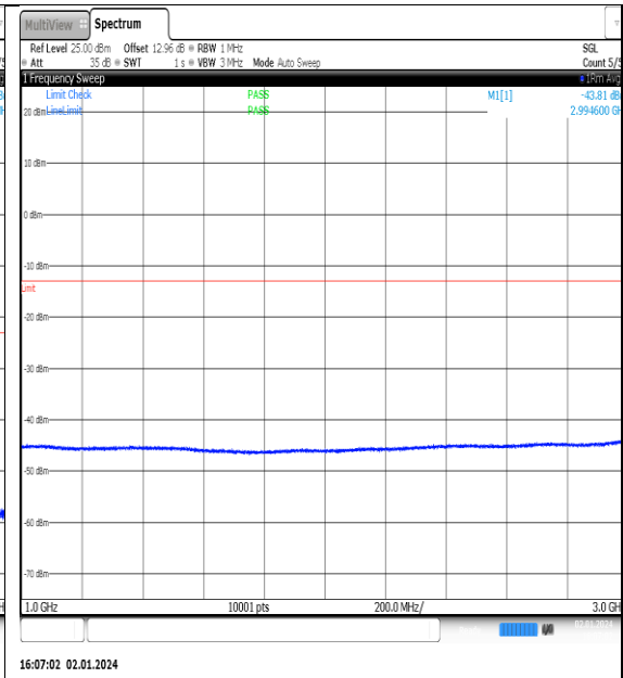
NTVN_N77-3450- 3550_PC2_30_90_L_TID14_NS_01_1000_3000_#1
