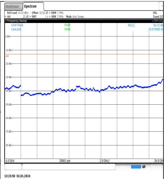
NTN_V_N77-3450- 3550_PC2_30_90_L_TID4_NS_01_6000_26000_# #1
