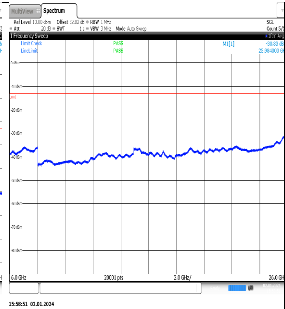
NTNV_N77-3450- 3550_PC2_30_90_L_TID12_NS_01_6000_26000_ #1
