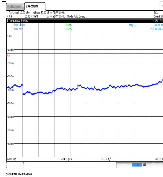
NTNV_N77-3450- 3550_PC2_30_90_L_TID13_NS_01_6000_26000 _#1
