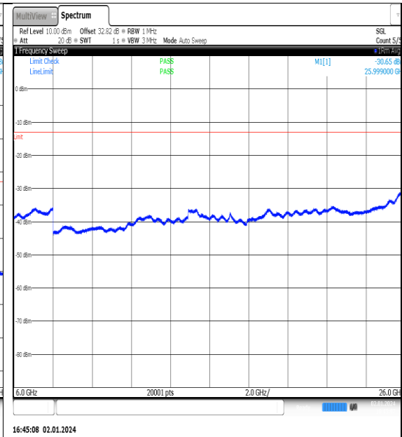
NTN_V_N77-3450- 3550_PC2_30_90_M_TID9_NS_01_6000_26000_# #1
