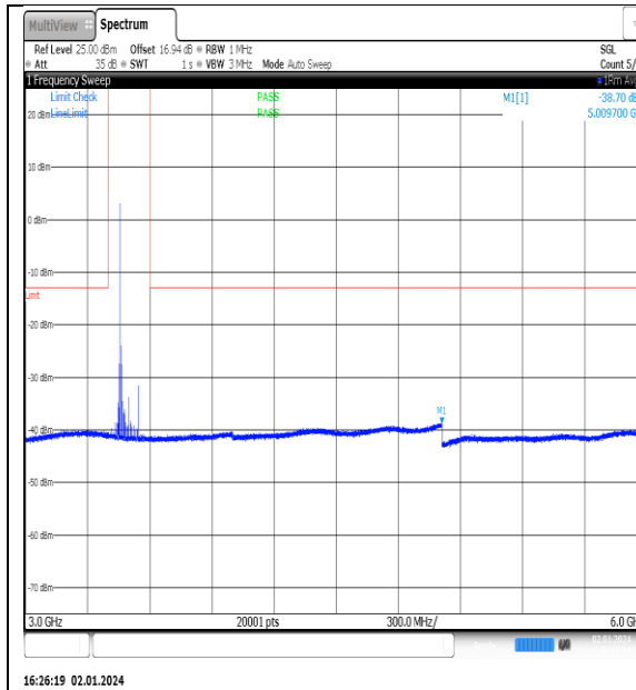
NTNV_N77-3450- 3550_PC2_30_90_M_TID5_NS_01_3000_6000_# 1
