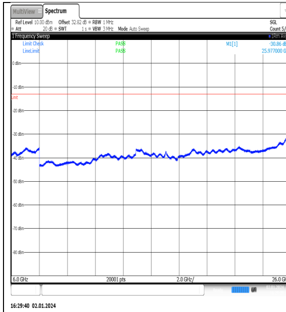
NTNV_N77-3450- 3550_PC2_30_90_M_TID6_NS_01_6000_26000_#1
