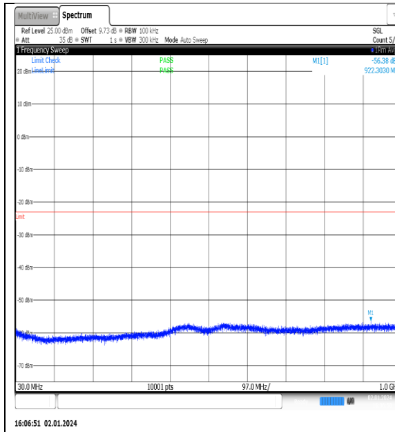
NTVN_N77-3450- 3550_PC2_30_90_L_TID14_NS_01_30_1000_#1
