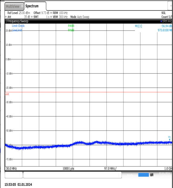
NTNV_N77-3450- 3550_PC2_30_90_L_TID11_NS_01_30_1000_#1
