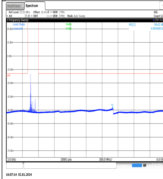
NTVN_N77-3450- 3550_PC2_30_90_L_TID14_NS_01_3000_6000_#1
