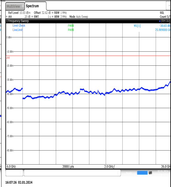
NTVN_N77-3450- 3550_PC2_30_90_L_TID14_NS_01_6000_26000_#1
