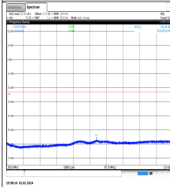
NTNV_N77-3450- 3550_PC2_30_90_L_TID12_NS_01_30_1000_#1
