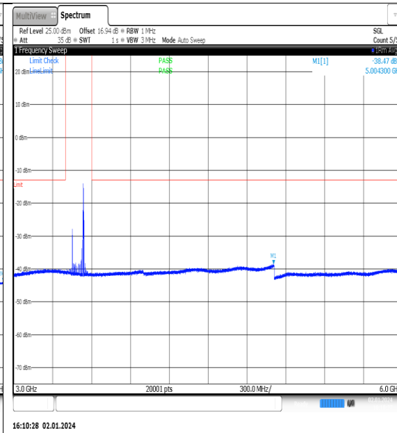
NTNV_N77-3450- 3550_PC2_30_90_L_TID15_NS_01_3000_6000_ #1
