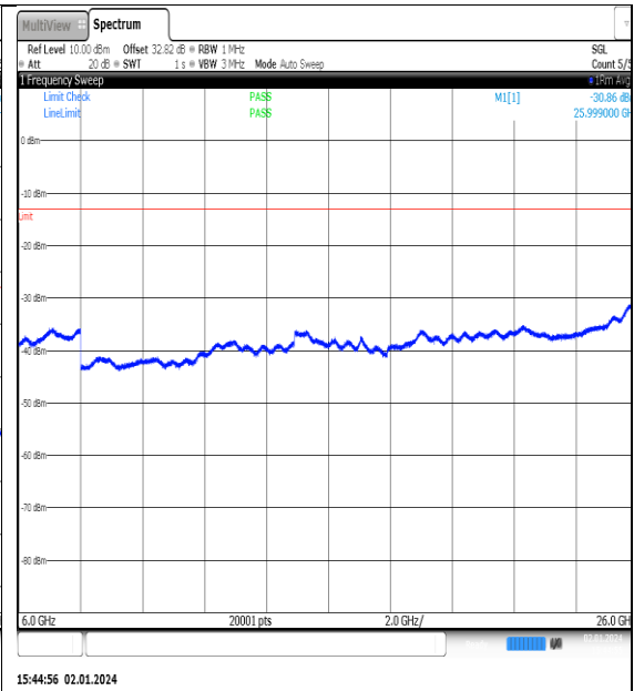
NTNV_N77-3450- 3550_PC2_30_90_L_TID8_NS_01_6000_26000_# #1
