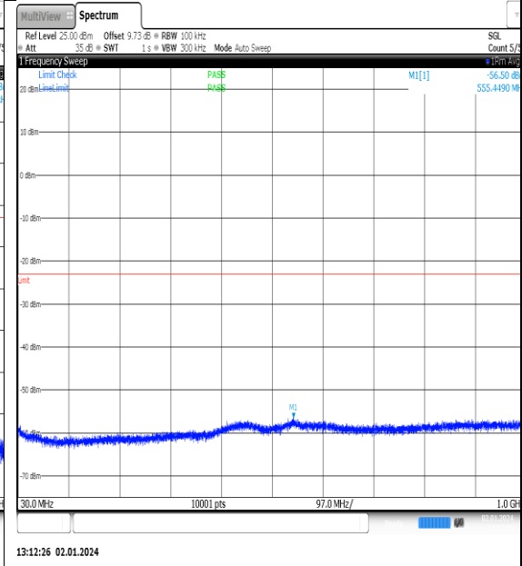
NTNV_N77-3450- 3550_PC2_30_90_L_TID3_NS_01_30_1000_#1
