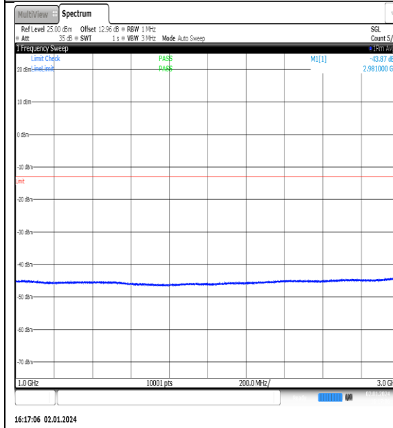
NTNV_N77-3450- 3550_PC2_30_90_M_TID2_NS_01_1000_3000_# 1
