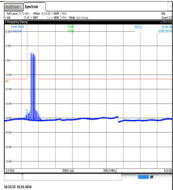
NTN_V_N77-3450- 3550_PC2_30_90_M_TID4_NS_01_3000_6000_# 1
