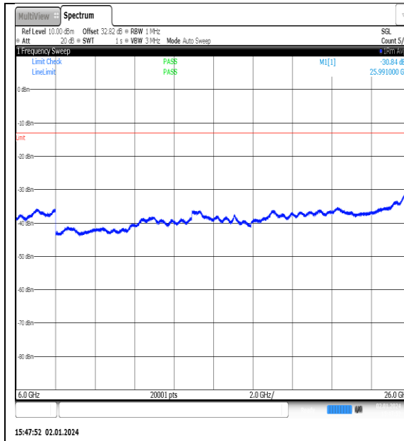
NTNV_N77-3450- 3550_PC2_30_90_L_TID9_NS_01_6000_26000_ #1
