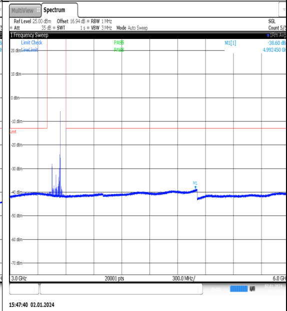
NTNV_N77-3450- 3550_PC2_30_90_L_TID9_NS_01_3000_6000_# 1
