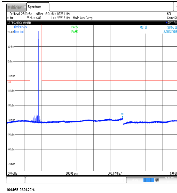
NTN_V_N77-3450- 3550_PC2_30_90_M_TID9_NS_01_3000_6000_# 1
