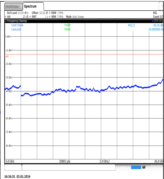
NTNV_N77-3450- 3550_PC2_30_90_M_TID5_NS_01_6000_26000_# 1
