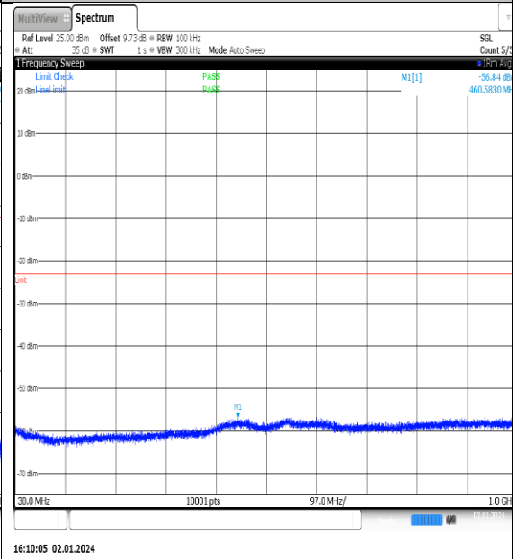
NTNV_N77-3450- 3550_PC2_30_90_L_TID15_NS_01_30_1000_#1
