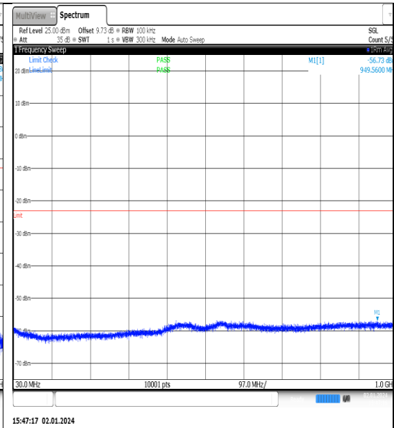
NTNV_N77-3450- 3550_PC2_30_90_L_TID9_NS_01_30_1000_#1
