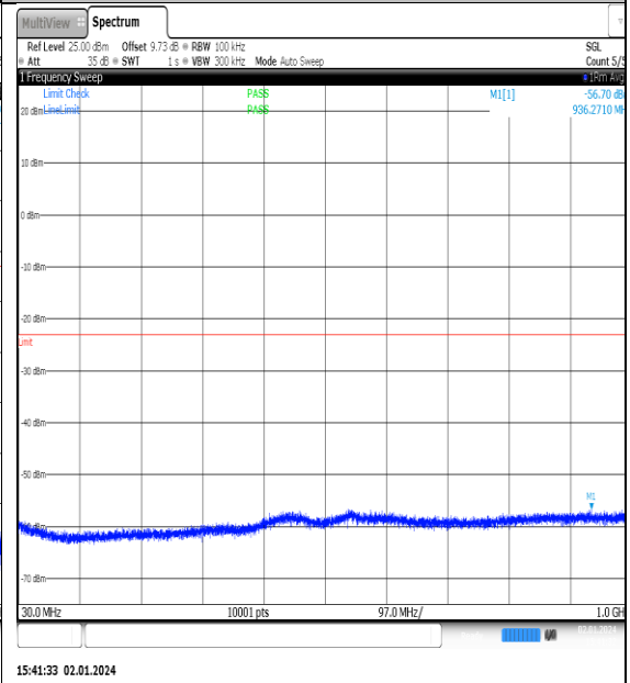
NTNV_N77-3450- 3550_PC2_30_90_L_TID7_NS_01_30_1000_#1
