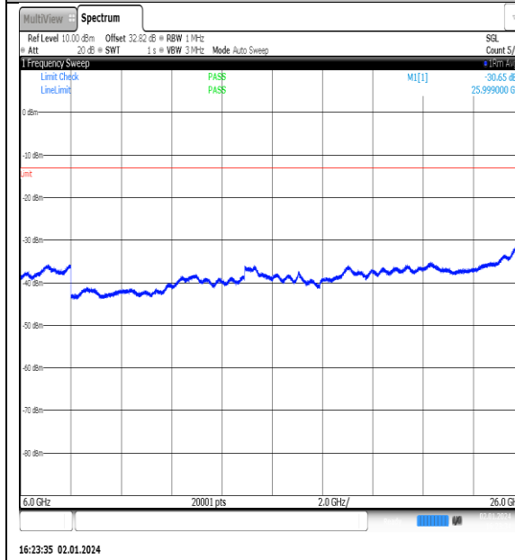
NTN_V_N77-3450- 3550_PC2_30_90_M_TID4_NS_01_6000_26000_# #1
