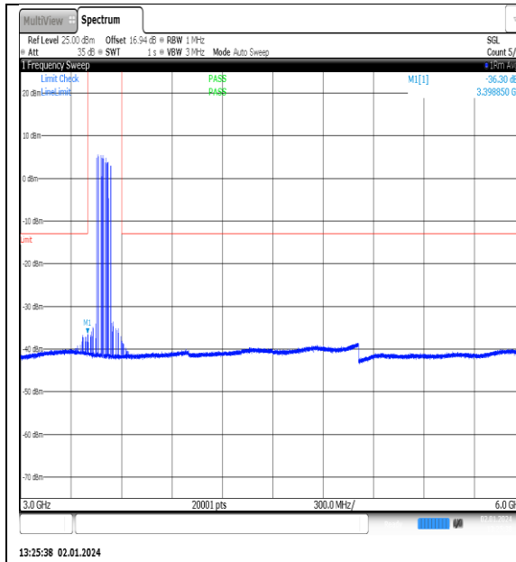
NTN_V_N77-3450- 3550_PC2_30_90_L_TID4_NS_01_3000_6000_# 1
