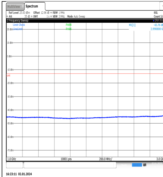
NTN_V_N77-3450- 3550_PC2_30_90_M_TID4_NS_01_1000_3000_# 1
