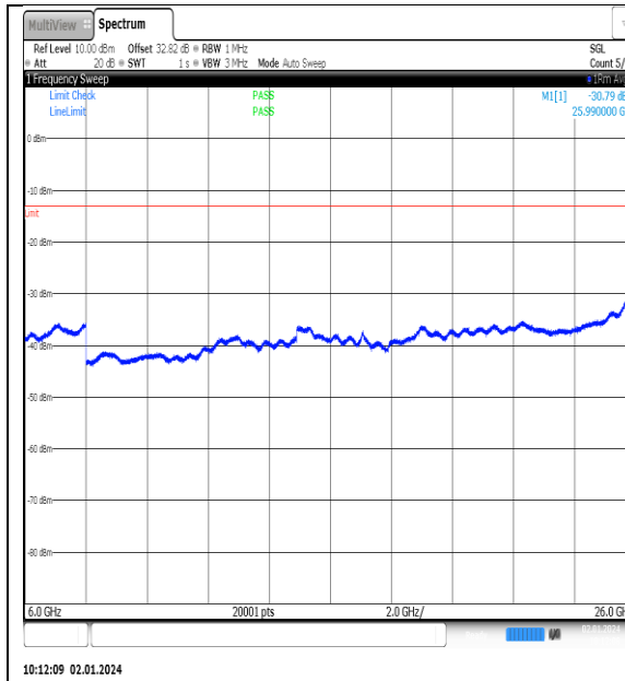
NTNV_N77-3450- 3550_PC2_30_90_L_TID2_NS_01_6000_26000_ #1
