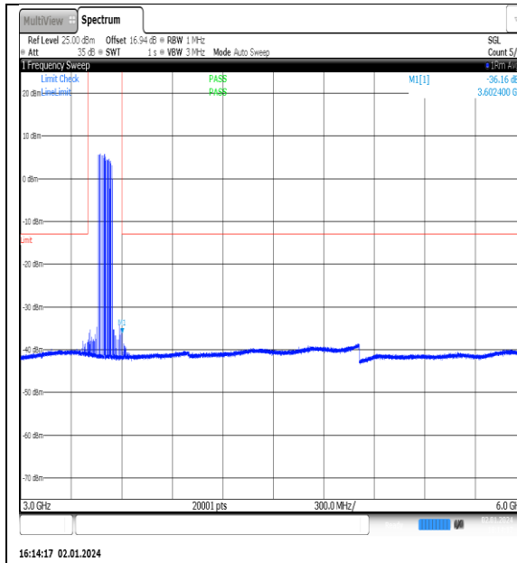
NTN_V_N77-3450- 3550_PC2_30_90_M_TID1_NS_01_3000_6000_# 1
