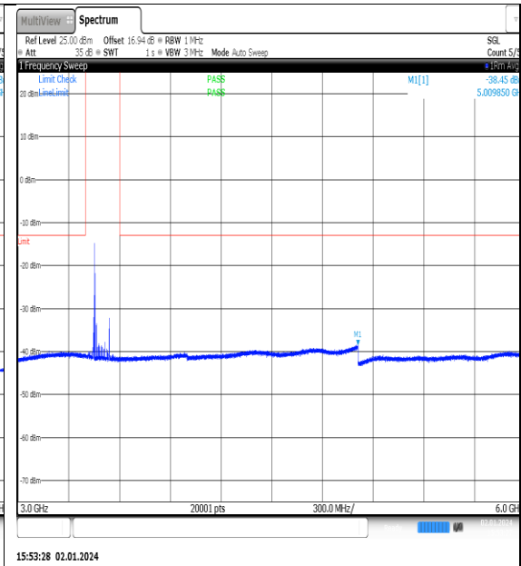
NTNV_N77-3450- 3550_PC2_30_90_L_TID11_NS_01_3000_6000_ #1
