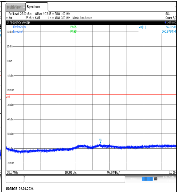
NTNV_N77-3450- 3550_PC2_30_90_L_TID5_NS_01_30_1000_#1
