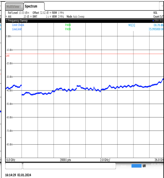
NTN_V_N77-3450- 3550_PC2_30_90_M_TID1_NS_01_6000_26000_# #1
