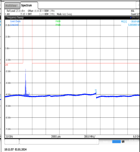
NTNV_N77-3450- 3550_PC2_30_90_L_TID2_NS_01_3000_6000_# 1
