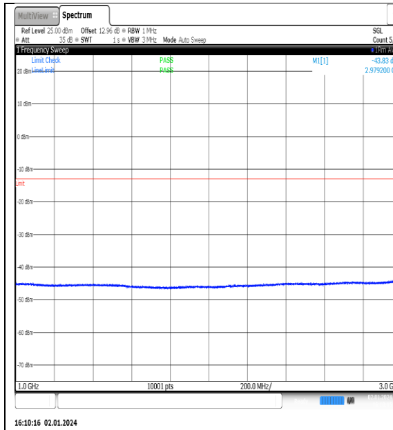
NTNV_N77-3450- 3550_PC2_30_90_L_TID15_NS_01_1000_3000_ #1
