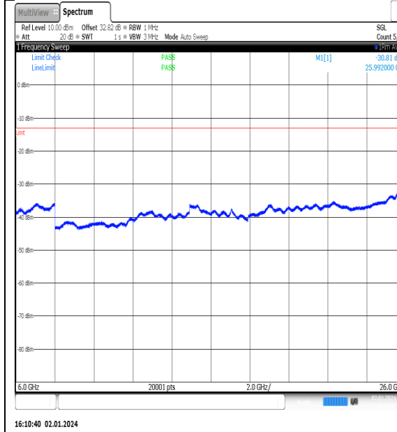
NTNV_N77-3450- 3550_PC2_30_90_L_TID15_NS_01_6000_26000 #1
