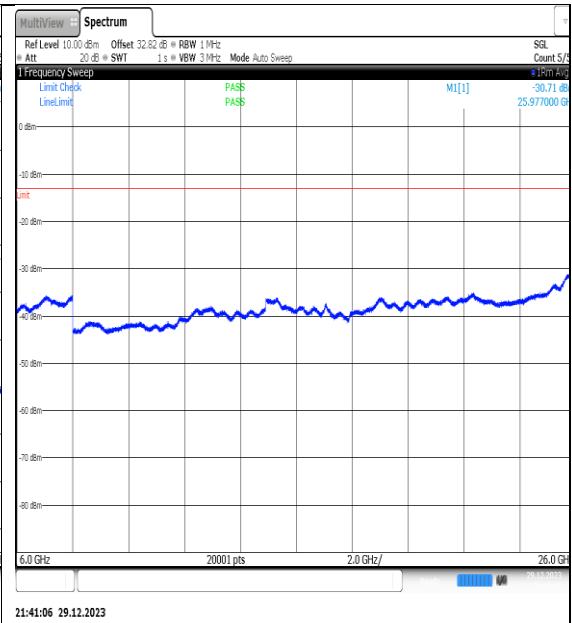
NTNV_N77-3450- 3550_PC2_30_80_H_TID5_NS_01_6000_26000_# 1
