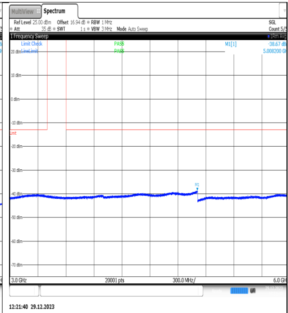
NTNV_N77-3450- 3550_PC2_30_80_M_TID5_NS_01_3000_6000_# 1
