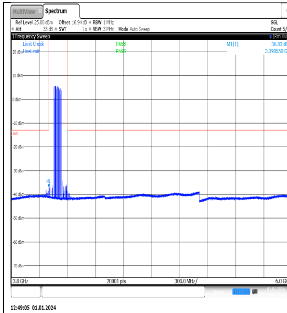
NTN_V_N77-3450- 3550_PC2_30_90_L_TID1_NS_01_3000_6000_# 1
