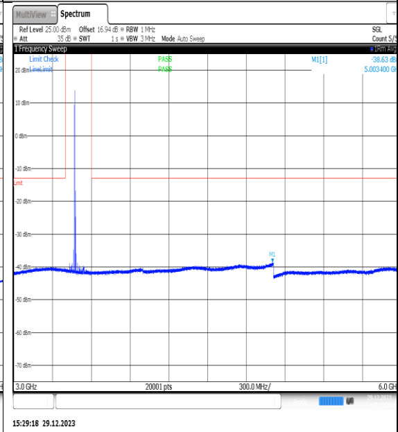
NTNV_N77-3450- 3550_PC2_30_80_H_TID2_NS_01_3000_6000_#
