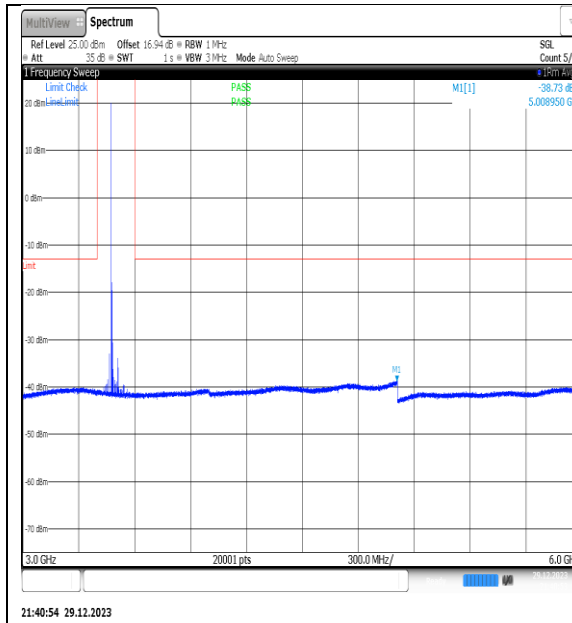
NTNV_N77-3450- 3550_PC2_30_80_H_TID5_NS_01_3000_6000_# 1
