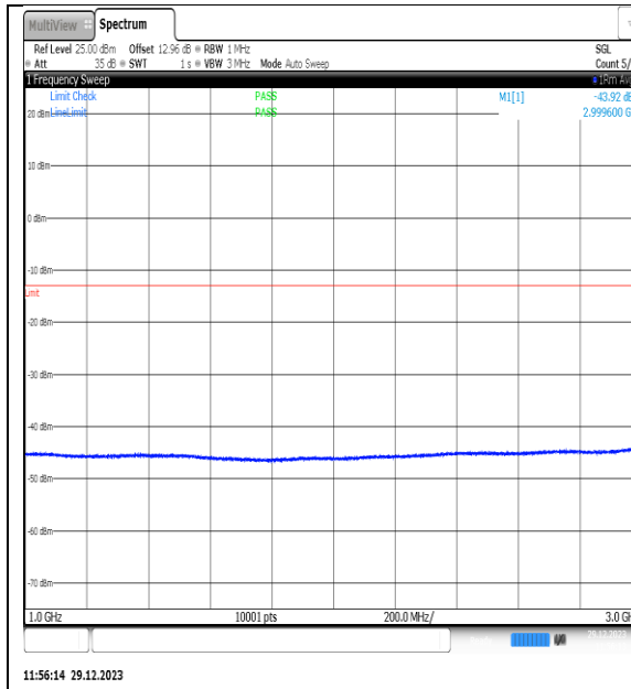
NTN_V_N77-3450- 3550_PC2_30_80_M_TID1_NS_01_1000_3000_# 1
