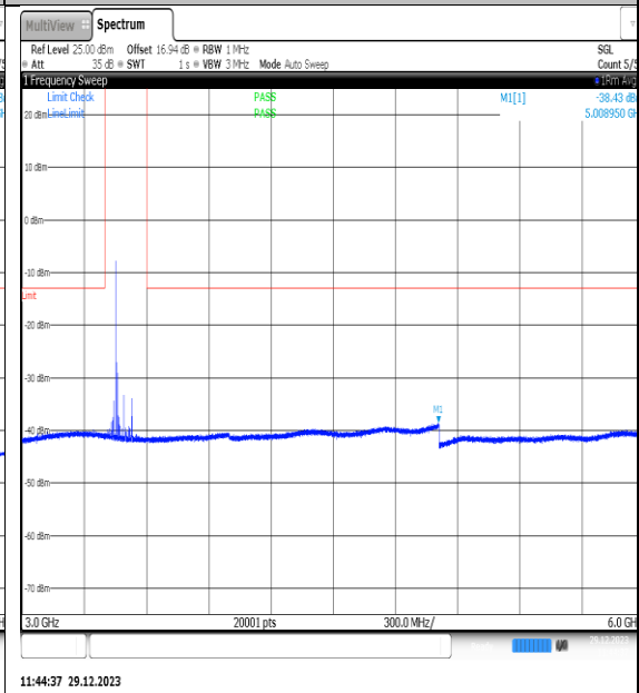
NTNV_N77-3450-3550_PC2_30_80_L_TID14_NS_01_3000_6000_#1
