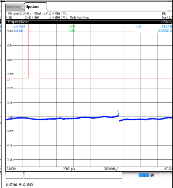
NTNV_N77-3450-3550_PC2_30_80_L_TID10_NS_01_3000_6000_#1
