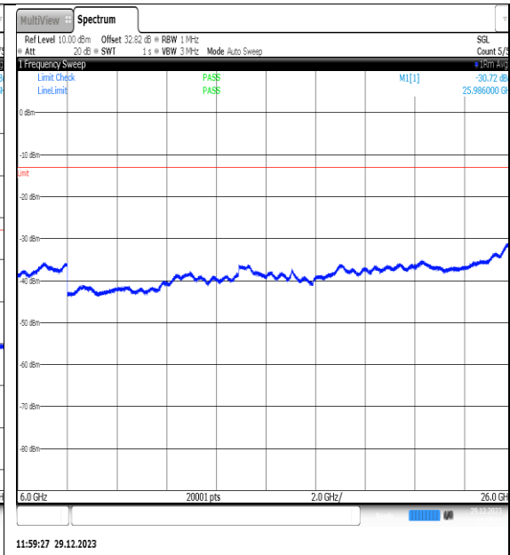
NTNV_N77-3450- 3550_PC2_30_80_M_TID2_NS_01_6000_26000_# #1
