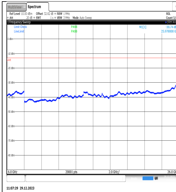
NTNV_N77-3450- 3550_PC2_30_80_L_TID10_NS_01_6000_26000 #1
