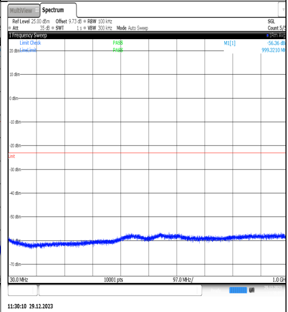
NTNV_N77-3450- 3550_PC2_30_80_L_TID12_NS_01_30_1000_#1
