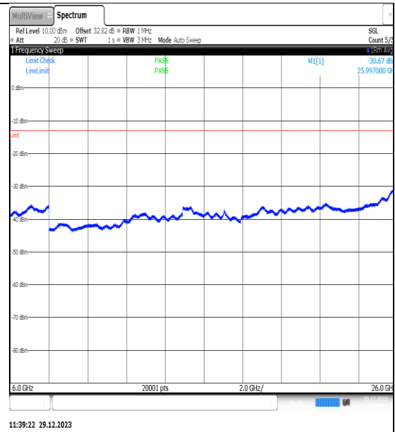
NTNV_N77-3450- 3550_PC2_30_80_L_TID13_NS_01_6000_26000_#1
