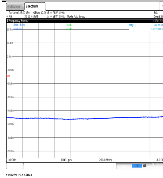
NTNV_N77-3450-3550_PC2_30_80_L_TID10_NS_01_1000_3000_#1
