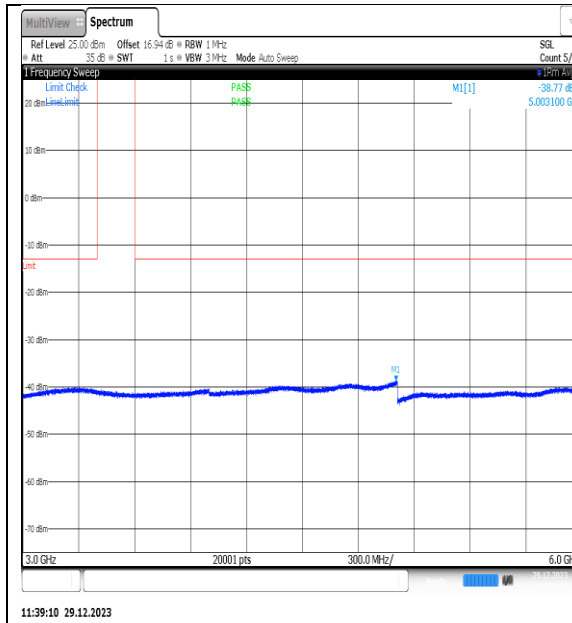
NTNV_N77-3450- 3550_PC2_30_80_L_TID13_NS_01_3000_6000_#1
