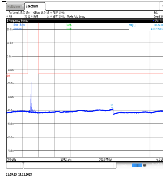
NTNV_N77-3450- 3550_PC2_30_80_M_TID2_NS_01_3000_6000_# 1
