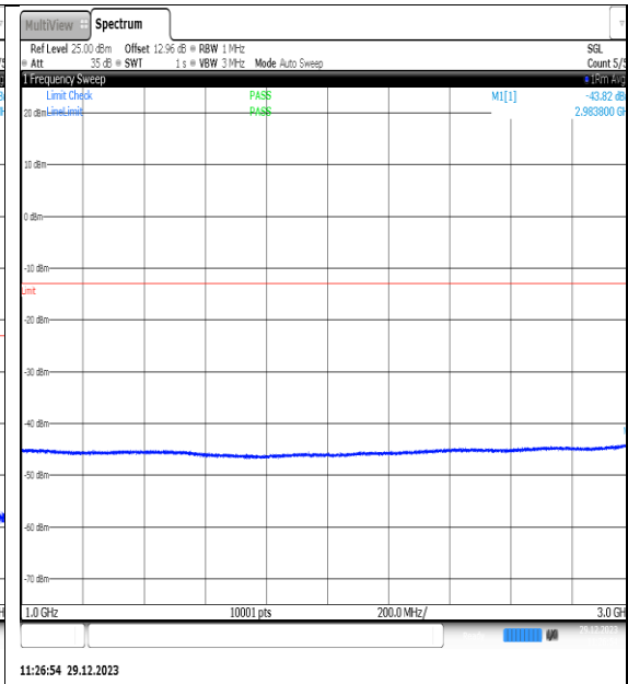
NTNV_N77-3450- 3550_PC2_30_80_L_TID11_NS_01_1000_3000_#1
