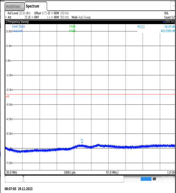
NTNV_N77-3450- 3550_PC2_30_80_L_TID4_NS_01_30_1000_#1
