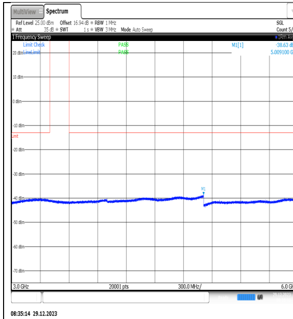
NTNV_N77-3450- 3550_PC2_30_80_L_TID5_NS_01_3000_6000_# 1
