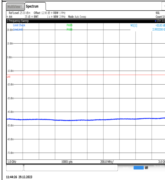
NTNV_N77-3450-3550_PC2_30_80_L_TID14_NS_01_1000_3000_#1
