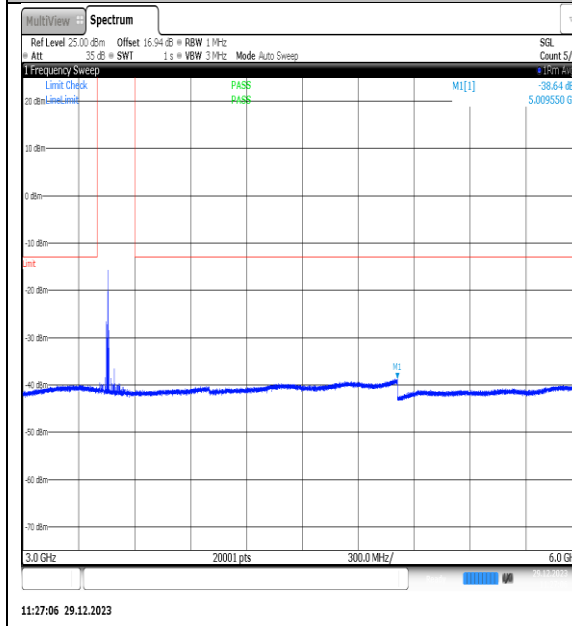
NTNV_N77-3450- 3550_PC2_30_80_L_TID11_NS_01_3000_6000_#1
