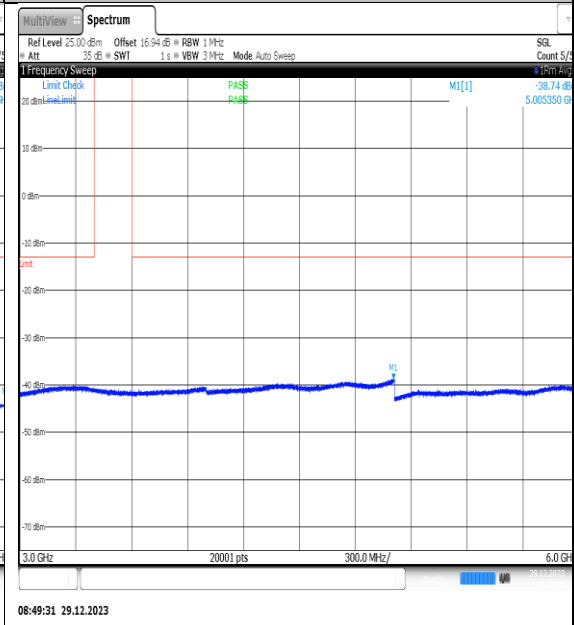
NTNV_N77-3450- 3550_PC2_30_80_L_TID6_NS_01_3000_6000_#
