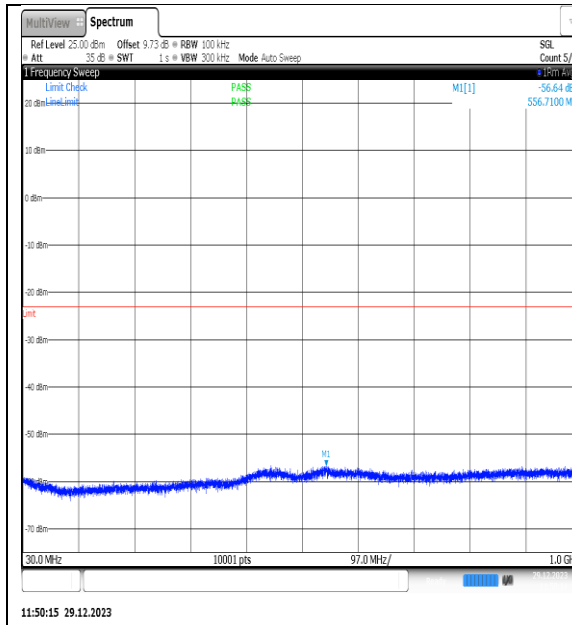
NTN_V_N77-3450- 3550_PC2_30_80_L_TID15_NS_01_30_1000_#1
