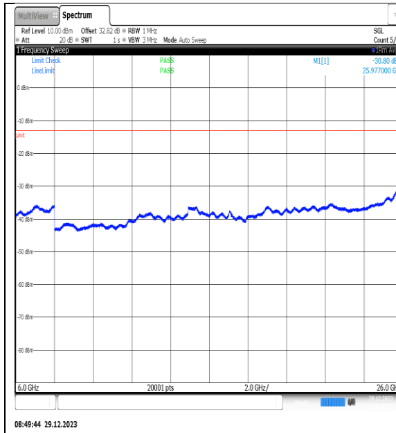
NTNV_N77-3450- 3550_PC2_30_80_L_TID6_NS_01_6000_26000_ #1
