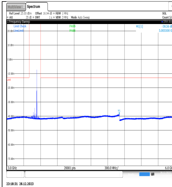
NTN_V_N77-3450- 3550_PC2_30_70_M_TID15_NS_01_3000_6000_ #1
