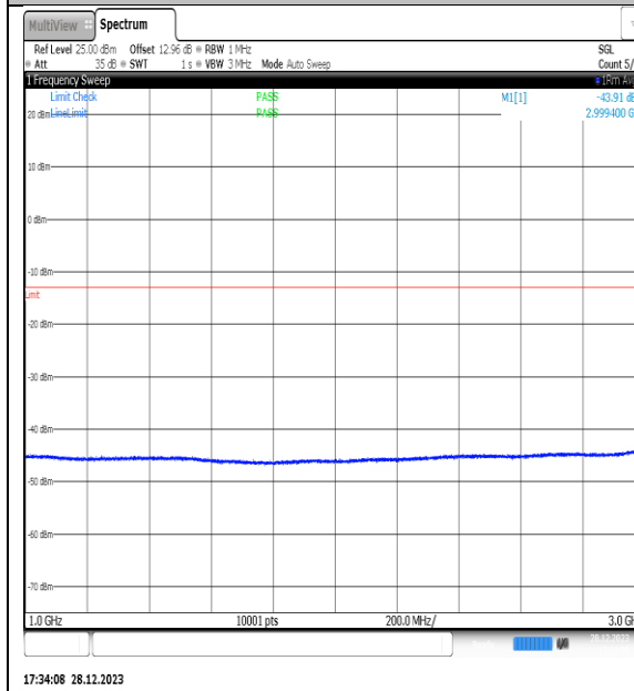
NTNV_N77-3450- 3550_PC2_30_70_M_TID4_NS_01_1000_3000_# 1
