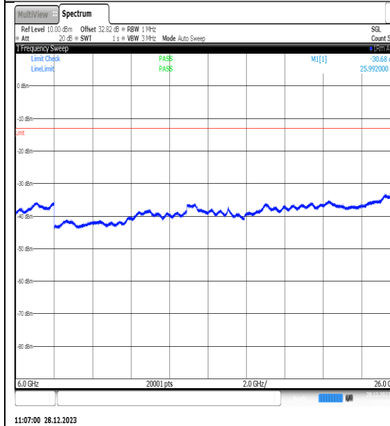
NTN_V_N77-3450- 3550_PC2_30_60_M_TID7_NS_01_6000_26000_# #1
