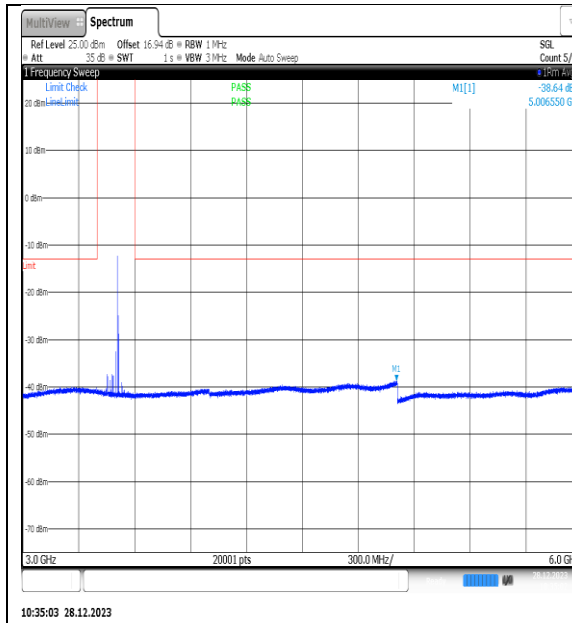
NTNV_N77-3450- 3550_PC2_30_60_L_TID15_NS_01_3000_6000_#1
