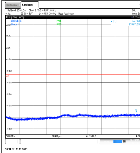
NTNV_N77-3450- 3550_PC2_30_60_L_TID15_NS_01_30_1000_#1
