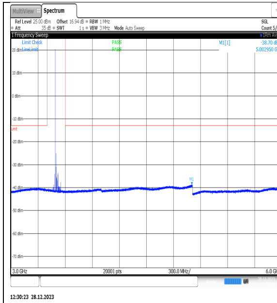
NTNV_N77-3450- 3550_PC2_30_60_H_TID5_NS_01_3000_6000_# 1
