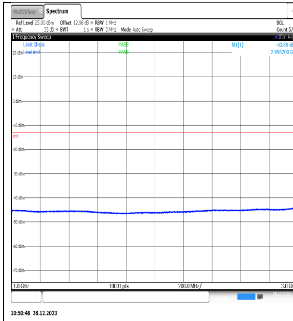
NTN_V_N77-3450- 3550_PC2_30_60_M_TID3_NS_01_1000_3000_# 1
