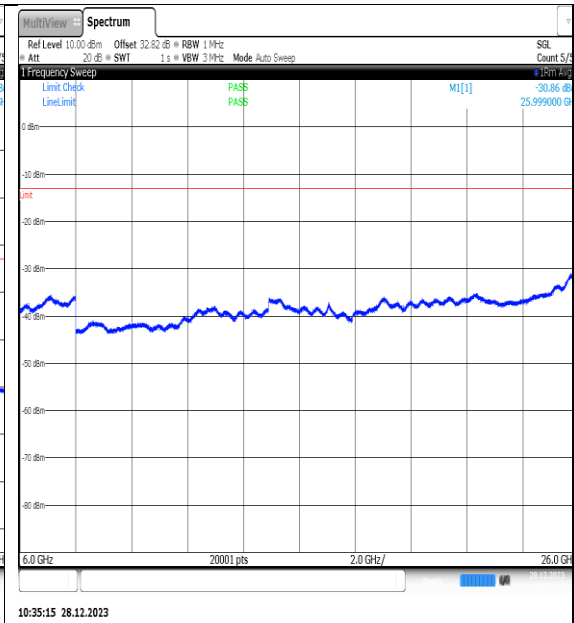
NTNV_N77-3450- 3550_PC2_30_60_L_TID15_NS_01_6000_26000_#1
