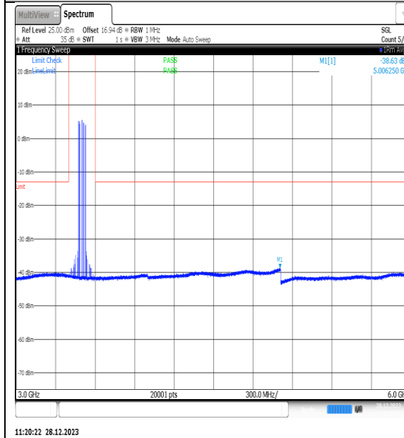
NTVN_N77-3450- 3550_PC2_30_60_M_TID10_NS_01_3000_6000_#1
