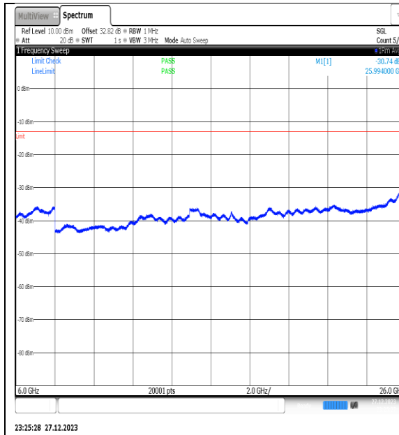
NTNV_N77-3450- 3550_PC2_30_60_L_TID5_NS_01_6000_26000_ #1
