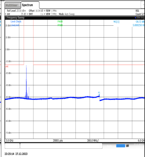
NTNV_N77-3450- 3550_PC2_30_60_L_TID5_NS_01_3000_6000_# 1
