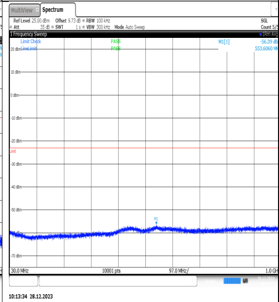
NTNV_N77-3450- 3550_PC2_30_60_L_TID10_NS_01_30_1000_#1
