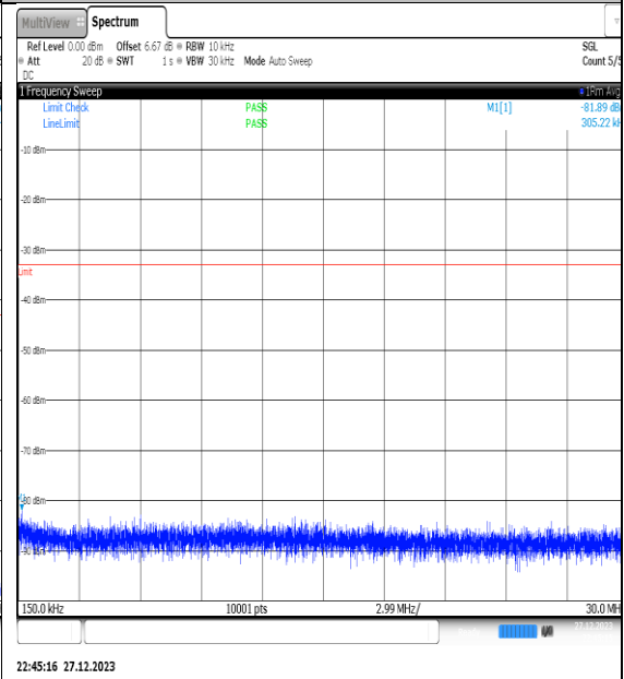
NTNV_N77-3450- 3550_PC2_30_60_L_TID2_NS_01_0.15_30_#1
