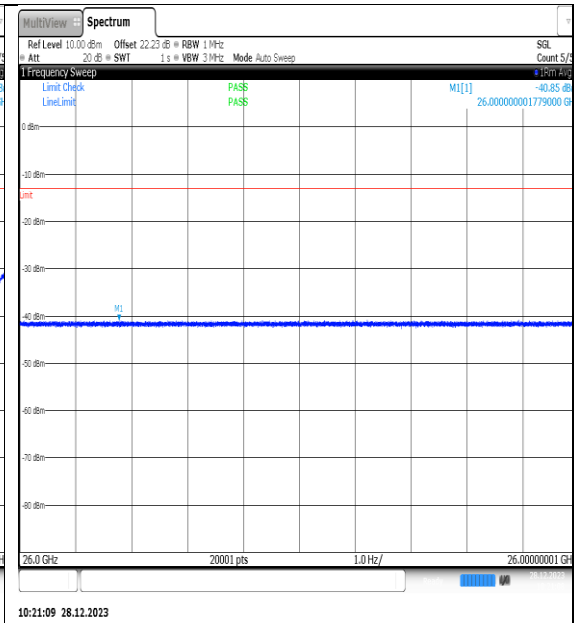
NTNV_N77-3450- 3550_PC2_30_60_L_TID12_NS_01_26000_4000 0_#1
