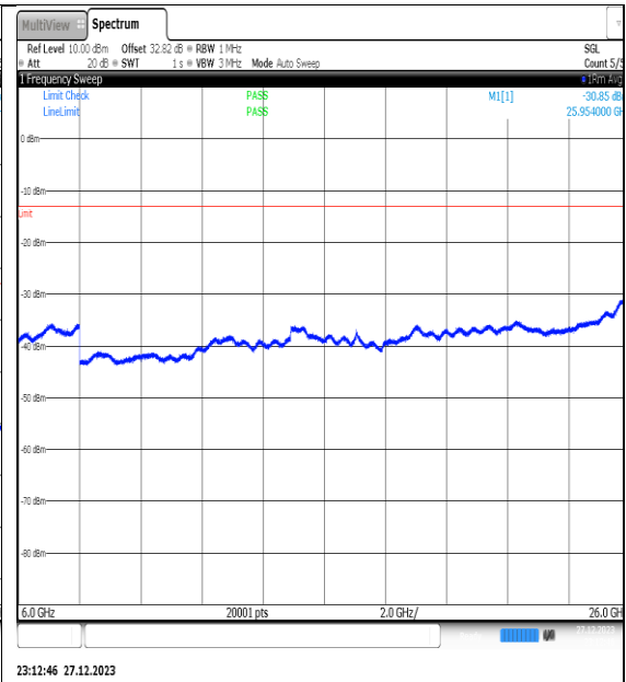
NTNV_N77-3450- 3550_PC2_30_60_L_TID4_NS_01_6000_26000_# 1
