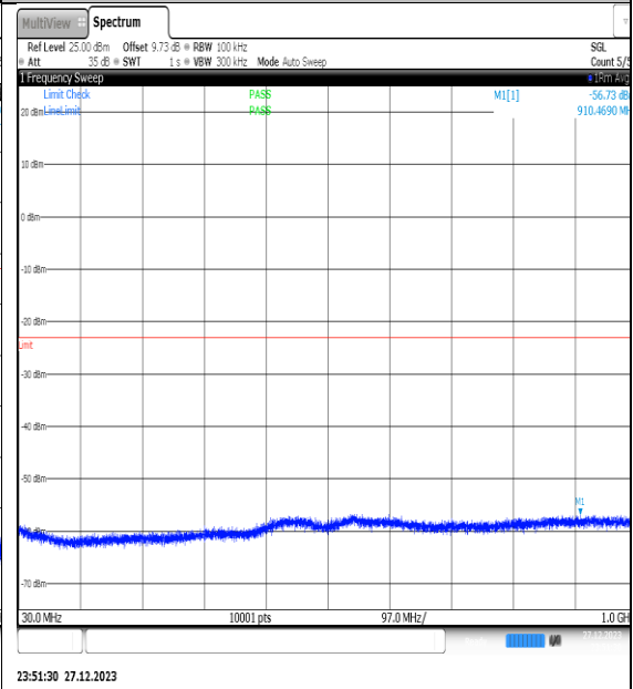
NTNV_N77-3450- 3550_PC2_30_60_L_TID7_NS_01_30_1000_#1
