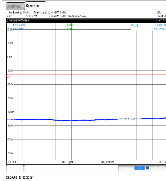
NTNV_N77-3450- 3550_PC2_30_60_L_TID5_NS_01_1000_3000_# 1
