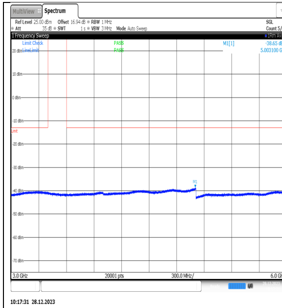
NTNV_N77-3450- 3550_PC2_30_60_L_TID11_NS_01_3000_6000_#1
