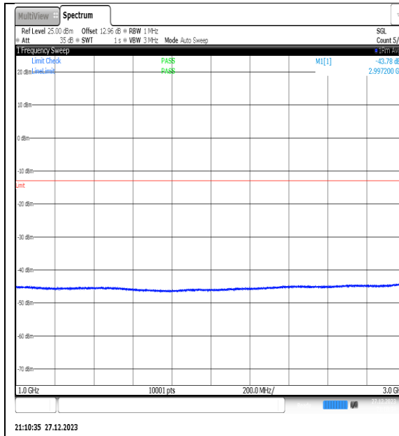
NTNV_N77-3450- 3550_PC2_30_50_H_TID9_NS_01_1000_3000_# 1
