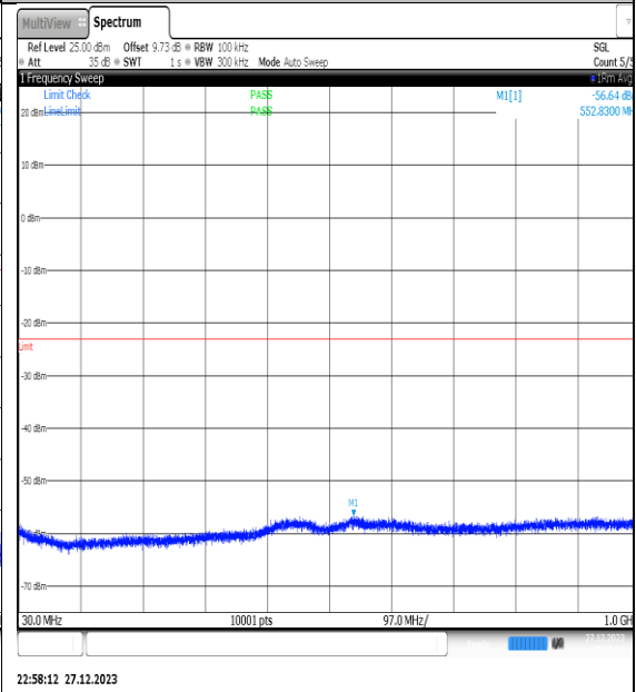
NTNV_N77-3450- 3550_PC2_30_60_L_TID3_NS_01_30_1000_#1
