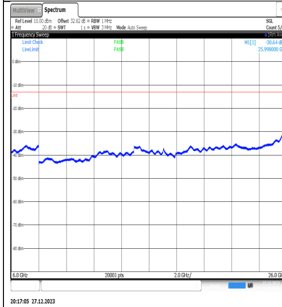
NTNV_N77-3450- 3550_PC2_30_50_H_TID5_NS_01_6000_26000_# 1
