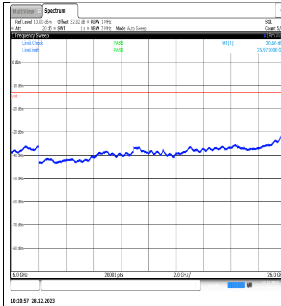
NTNV_N77-3450- 3550_PC2_30_60_L_TID12_NS_01_6000_26000 #1
