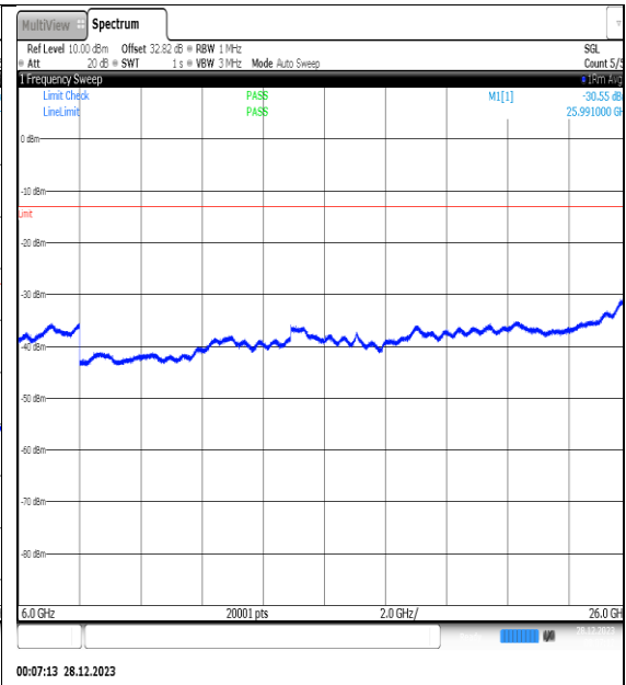
NTNV_N77-3450- 3550_PC2_30_60_L_TID8_NS_01_6000_26000_# 1
