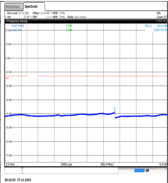
NTNV_N77-3450- 3550_PC2_30_50_H_TID5_NS_01_3000_6000_# 1
