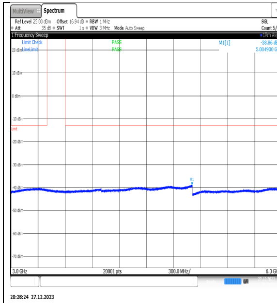
NTNV_N77-3450- 3550_PC2_30_50_H_TID6_NS_01_3000_6000_# 1
