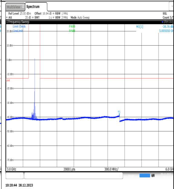
NTNV_N77-3450- 3550_PC2_30_60_L_TID12_NS_01_3000_6000_#1
