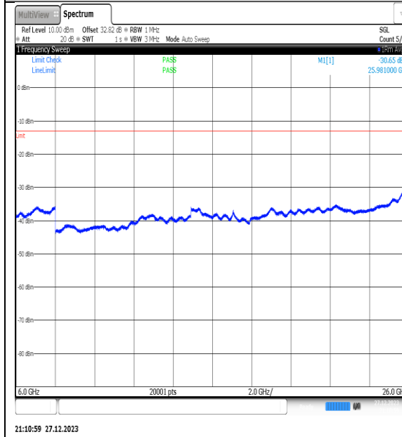
NTNV_N77-3450- 3550_PC2_30_50_H_TID9_NS_01_6000_26000_# #1
