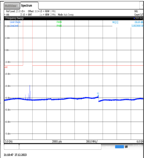
NTNV_N77-3450- 3550_PC2_30_50_H_TID9_NS_01_3000_6000_# 1
