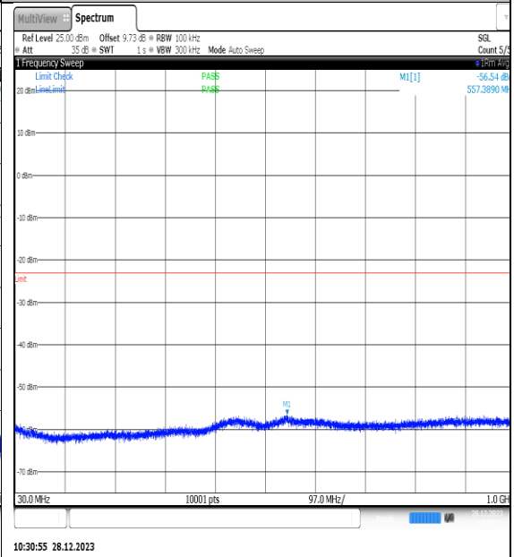
NTNV_N77-3450- 3550_PC2_30_60_L_TID14_NS_01_30_1000_#1
