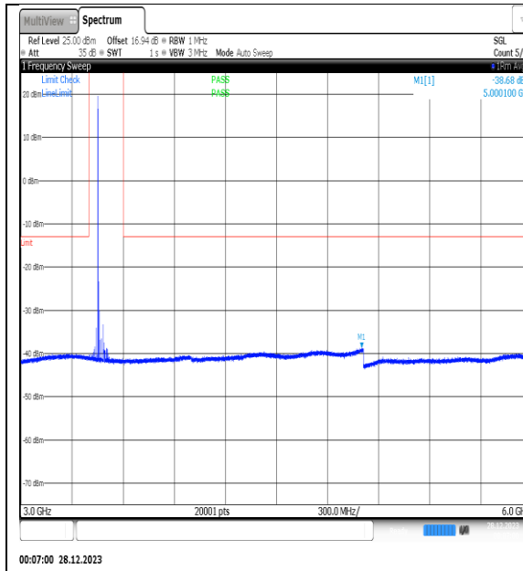
NTNV_N77-3450- 3550_PC2_30_60_L_TID8_NS_01_3000_6000_# 1
