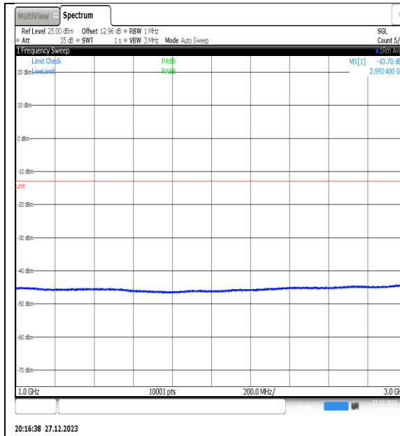
NTNV_N77-3450- 3550_PC2_30_50_H_TID5_NS_01_1000_3000_# 1
