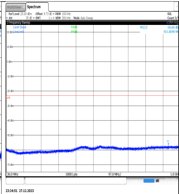
NTNV_N77-3450- 3550_PC2_30_60_L_TID5_NS_01_30_1000_#1
