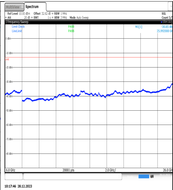
NTNV_N77-3450- 3550_PC2_30_60_L_TID11_NS_01_6000_26000_#1
