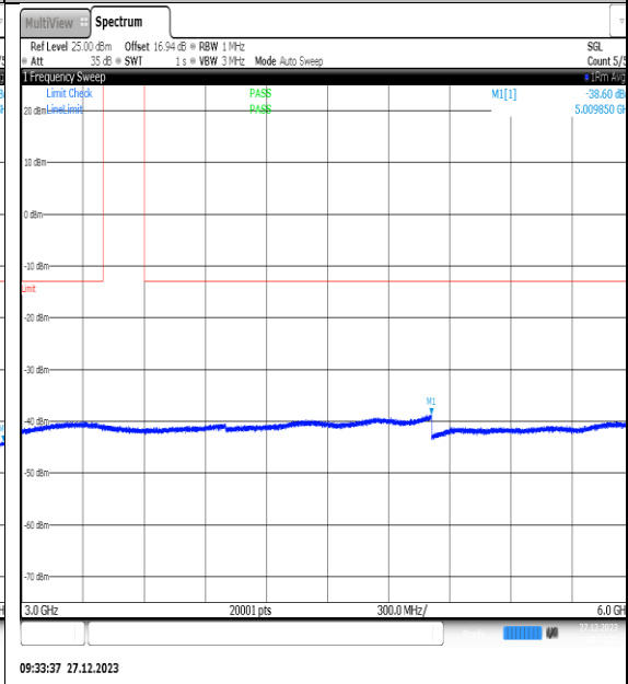
NTNV_N77-3450-3550_PC2_30_50_L_TID7_NS_01_3000_6000_#1
