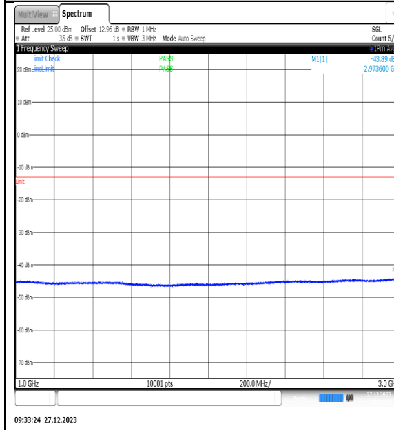
NTNV_N77-3450-3550_PC2_30_50_L_TID7_NS_01_1000_3000_#1
