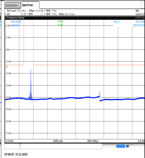
NTNV_N77-3450- 3550_PC2_30_40_H_TID6_NS_01_3000_6000_# 1
