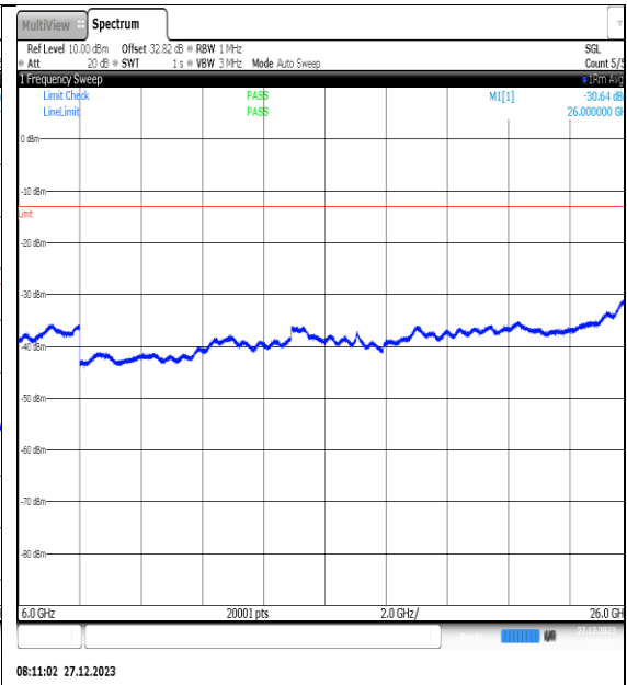
NTNV_N77-3450- 3550_PC2_30_40_H_TID9_NS_01_6000_26000_# 1
