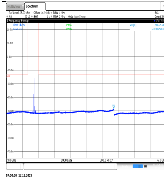
NTNV_N77-3450- 3550_PC2_30_40_H_TID5_NS_01_3000_6000_# 1
