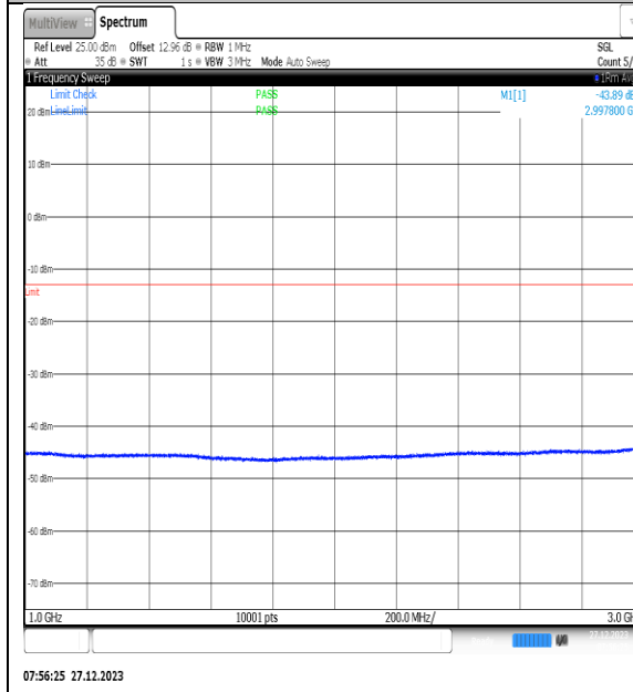
NTNV_N77-3450- 3550_PC2_30_40_H_TID6_NS_01_1000_3000_# 1
