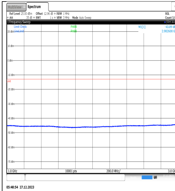
NTNV_N77-3450- 3550_PC2_30_40_L_TID10_NS_01_1000_3000_ #1
