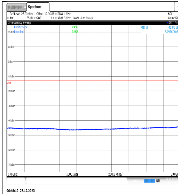
NTN_V_N77-3450- 3550_PC2_30_40_M_TID7_NS_01_1000_3000_# 1
