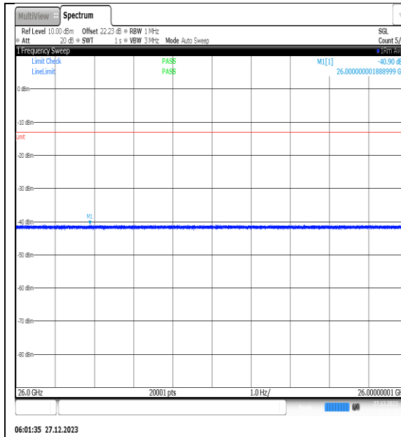
NTNV_N77-3450- 3550_PC2_30_40_L_TID13_NS_01_26000_4000 0_#1
