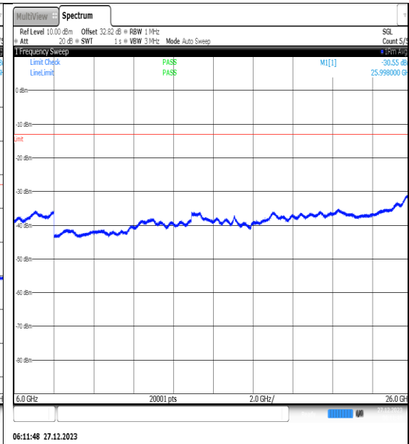
NTNV_N77-3450- 3550_PC2_30_40_L_TID15_NS_01_6000_26000 _#1
