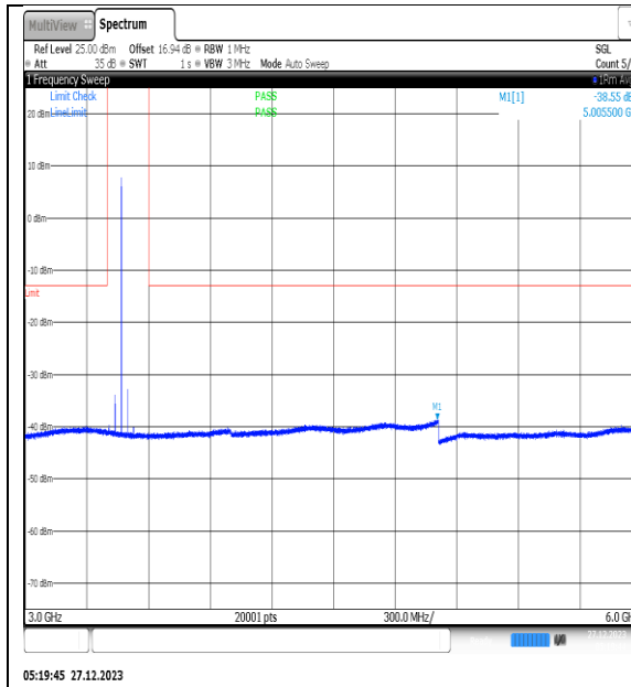
NTNV_N77-3450- 3550_PC2_30_40_L_TID7_NS_01_3000_6000_# 1
