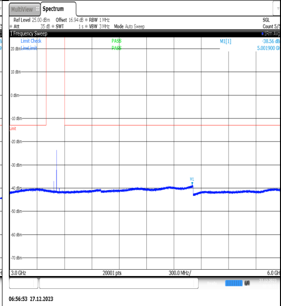
NTNV_N77-3450- 3550_PC2_30_40_M_TID9_NS_01_3000_6000_# 1
