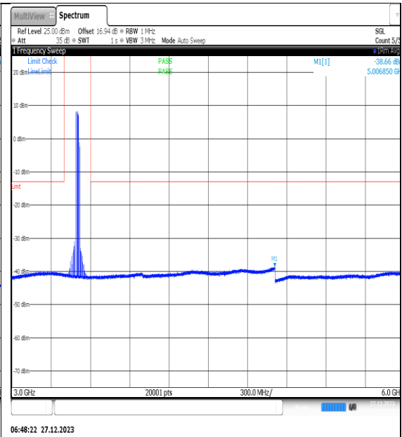
NTN_V_N77-3450- 3550_PC2_30_40_M_TID7_NS_01_3000_6000_# 1
