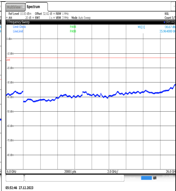
NTNV_N77-3450- 3550_PC2_30_40_L_TID11_NS_01_6000_26000 _#1
