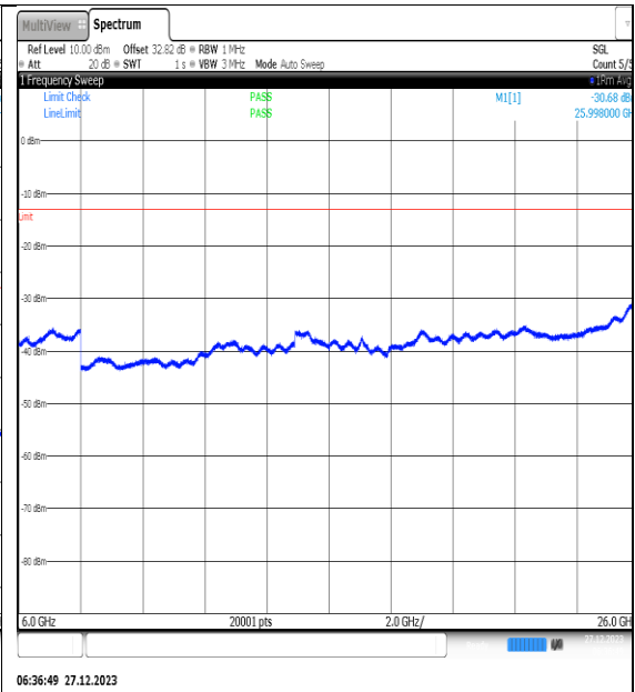
NTNV_N77-3450- 3550_PC2_30_40_M_TID4_NS_01_6000_26000_# 1
