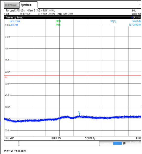
NTNV_N77-3450- 3550_PC2_30_40_L_TID6_NS_01_30_1000_#1
