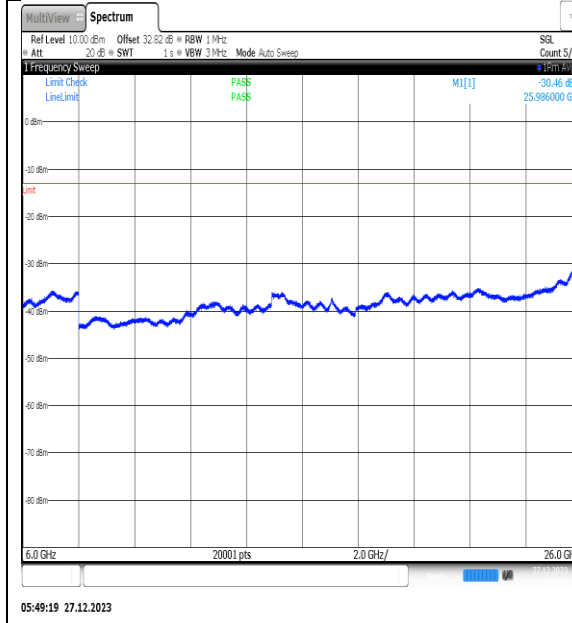
NTNV_N77-3450- 3550_PC2_30_40_L_TID10_NS_01_6000_26000_ #1
