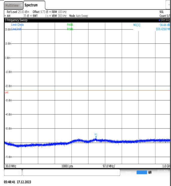
NTNV_N77-3450- 3550_PC2_30_40_L_TID10_NS_01_30_1000_#1
