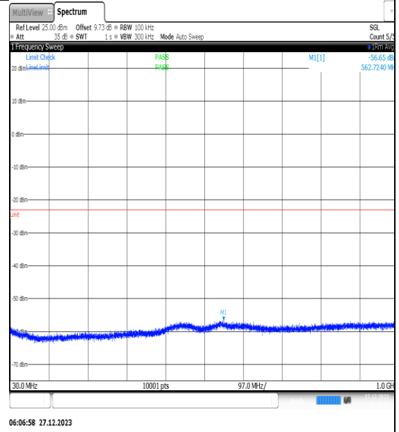
NTNV_N77-3450- 3550_PC2_30_40_L_TID14_NS_01_30_1000_#1
