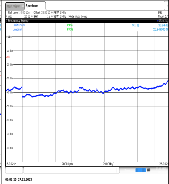
NTNV_N77-3450- 3550_PC2_30_40_L_TID13_NS_01_6000_26000_#1
