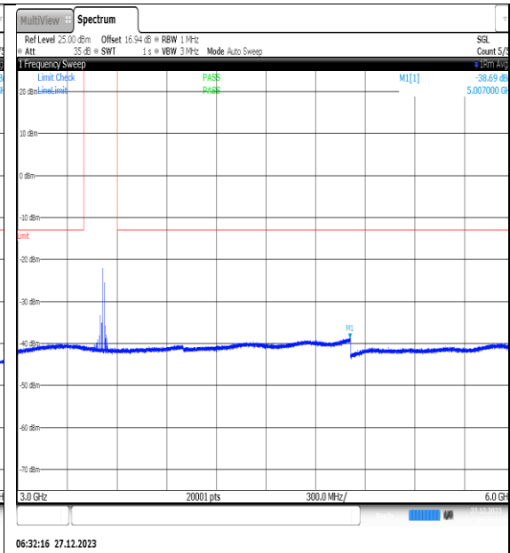
NTNV_N77-3450- 3550_PC2_30_40_M_TID3_NS_01_3000_6000_# 1
