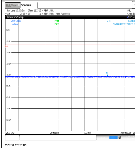
NTNV_N77-3450- 3550_PC2_30_40_L_TID11_NS_01_26000_4000 0_#1
