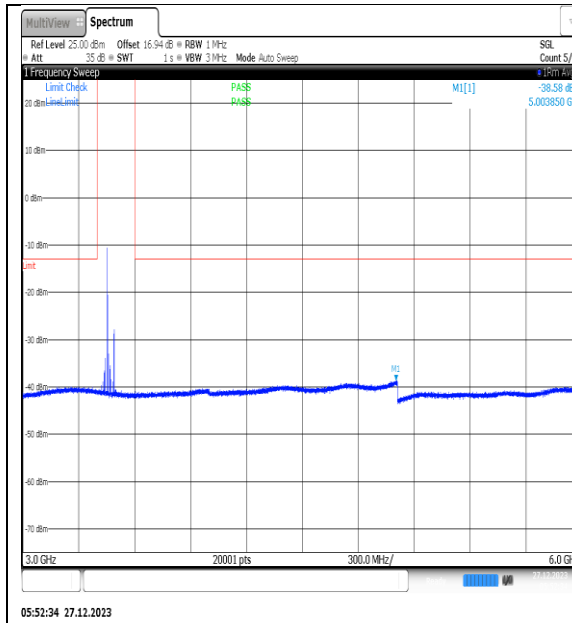
NTNV_N77-3450- 3550_PC2_30_40_L_TID11_NS_01_3000_6000_ #1
