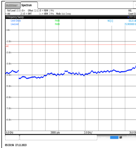
NTNV_N77-3450- 3550_PC2_30_40_L_TID8_NS_01_6000_26000_#1
