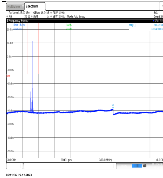
NTNV_N77-3450- 3550_PC2_30_40_L_TID15_NS_01_3000_6000_ #1
