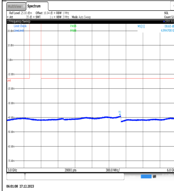
NTNV_N77-3450- 3550_PC2_30_40_L_TID13_NS_01_3000_6000_#1
