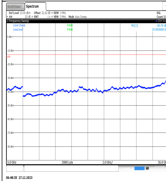
NTN_V_N77-3450- 3550_PC2_30_40_M_TID7_NS_01_6000_26000_# #1
