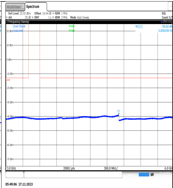
NTNV_N77-3450- 3550_PC2_30_40_L_TID10_NS_01_3000_6000_ #1
