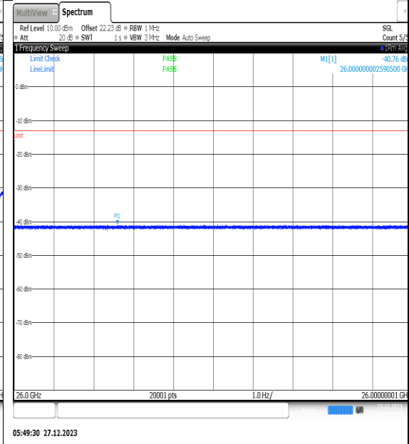
NTNV_N77-3450- 3550_PC2_30_40_L_TID10_NS_01_26000_4000_ 0_#1
