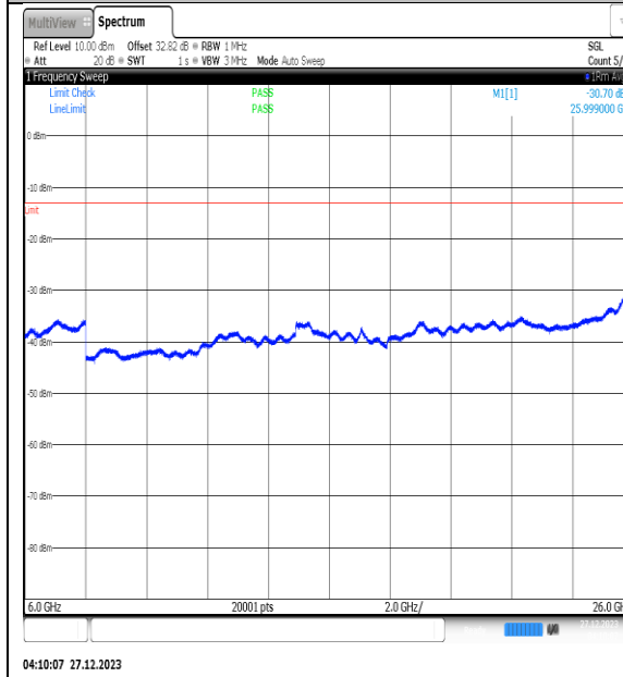
NTNV_N77-3450- 3550_PC2_30_30_H_TID9_NS_01_6000_26000_# #1
