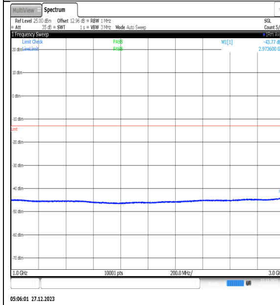
NTNV_N77-3450- 3550_PC2_30_40_L_TID4_NS_01_1000_3000_#
