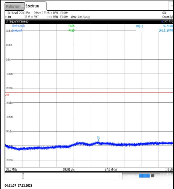
NTNV_N77-3450- 3550_PC2_30_40_L_TID2_NS_01_30_1000_#1
