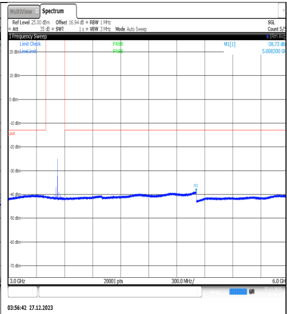
NTNV_N77-3450- 3550_PC2_30_30_H_TID5_NS_01_3000_6000_# 1
