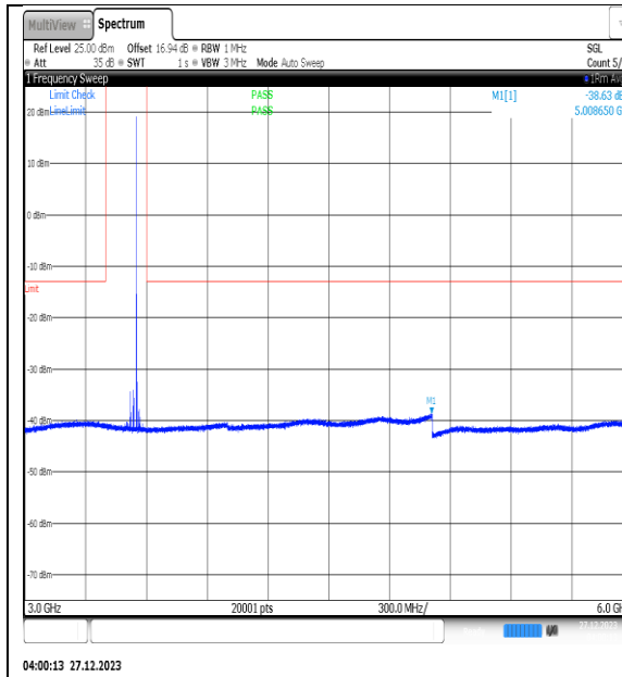
NTNV_N77-3450- 3550_PC2_30_30_H_TID6_NS_01_3000_6000_# 1
