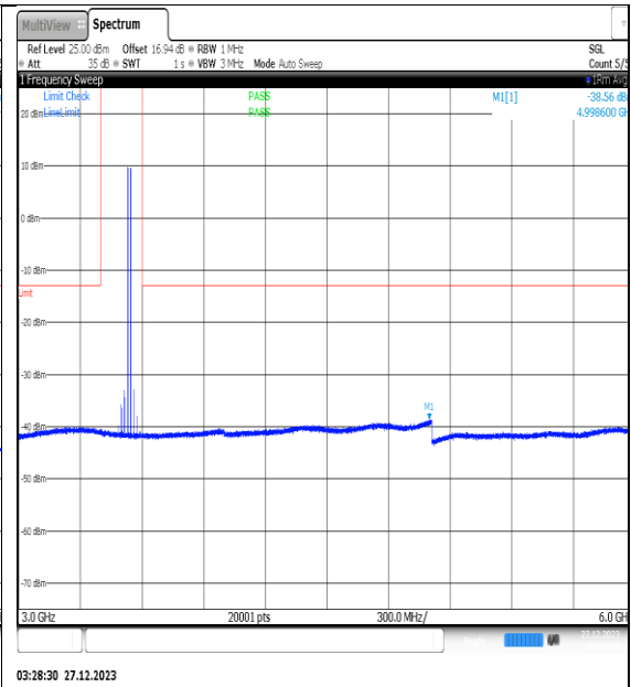
NTNV_N77-3450- 3550_PC2_30_30_H_TID1_NS_01_3000_6000_# 1
