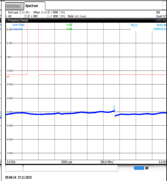
NTNV_N77-3450- 3550_PC2_30_40_L_TID4_NS_01_3000_6000_#
