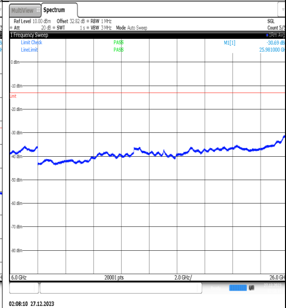
NTNV_N77-3450- 3550_PC2_30_30_L_TID14_NS_01_6000_26000_#1
