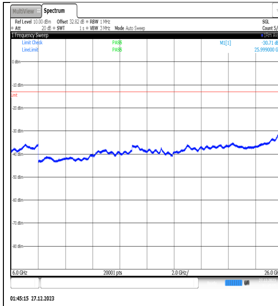
NTNV_N77-3450- 3550_PC2_30_30_L_TID9_NS_01_6000_26000_ #1
