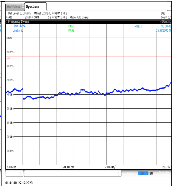
NTNV_N77-3450- 3550_PC2_30_30_L_TID8_NS_01_6000_26000_# 1
