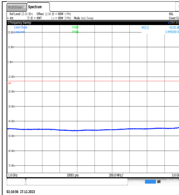
NTNV_N77-3450- 3550_PC2_30_30_L_TID15_NS_01_1000_3000_ #1
