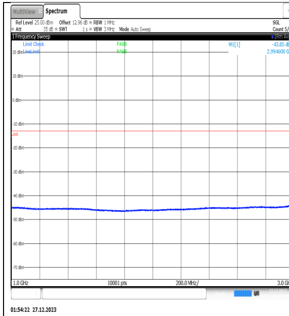
NTNV_N77-3450- 3550_PC2_30_30_L_TID11_NS_01_1000_3000_ #1
