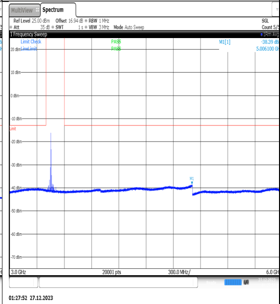
NTNV_N77-3450- 3550_PC2_30_30_L_TID5_NS_01_3000_6000_#1
