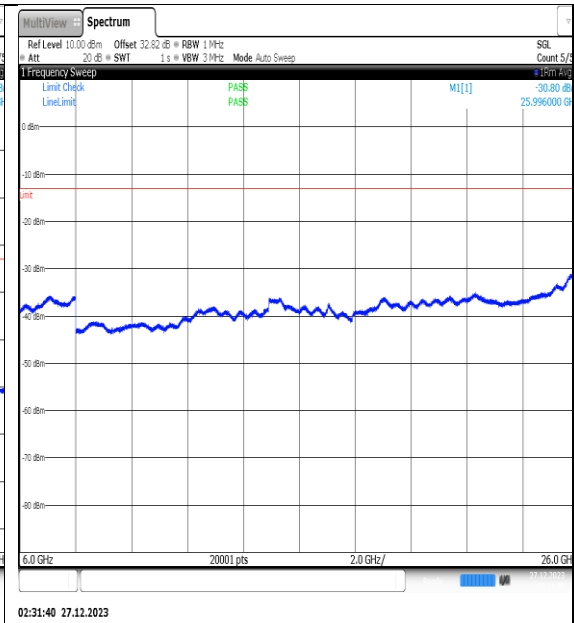
NTNV_N77-3450- 3550_PC2_30_30_M_TID5_NS_01_6000_26000_# 1
