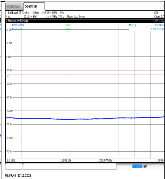
NTNV_N77-3450- 3550_PC2_30_30_L_TID14_NS_01_1000_3000_#1
