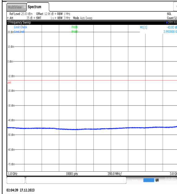
NTNV_N77-3450-3550_PC2_30_30_L_TID13_NS_01_1000_3000_#1
