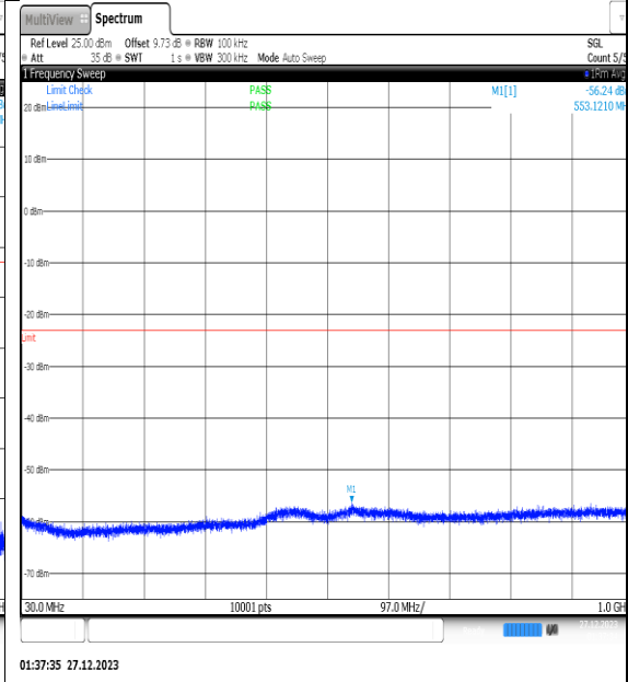
NTNV_N77-3450- 3550_PC2_30_30_L_TID7_NS_01_30_1000_#1
