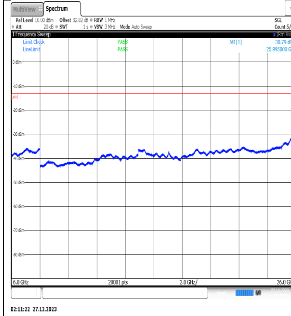
NTNV_N77-3450- 3550_PC2_30_30_L_TID15_NS_01_6000_26000 _#1
