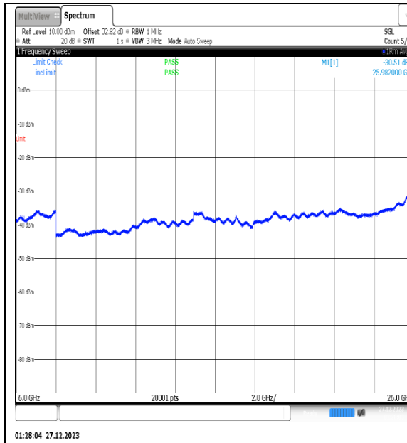
NTNV_N77-3450- 3550_PC2_30_30_L_TID5_NS_01_6000_26000_ #1
