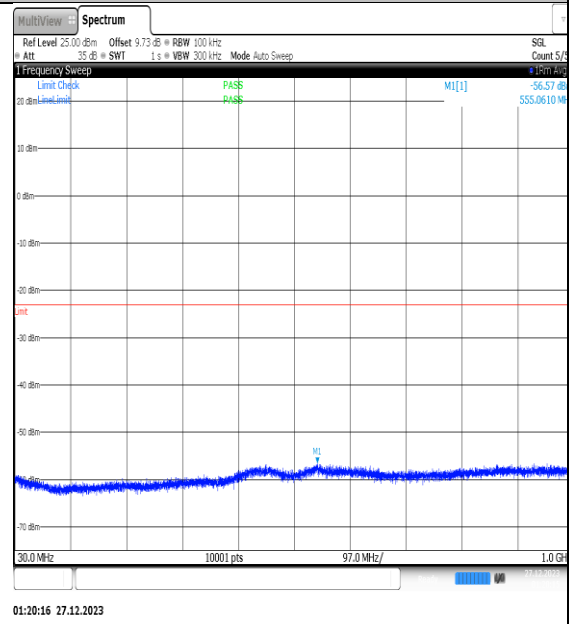
NTNV_N77-3450- 3550_PC2_30_30_L_TID3_NS_01_30_1000_#1
