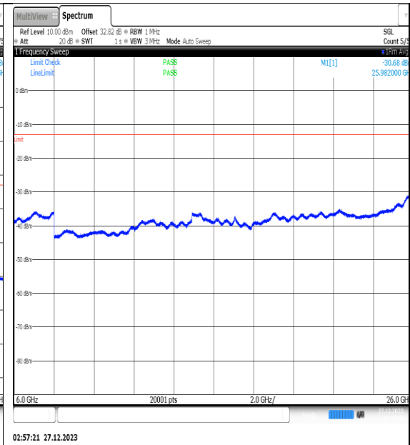
NTNV_N77-3450- 3550_PC2_30_30_M_TID9_NS_01_6000_26000_# 1
