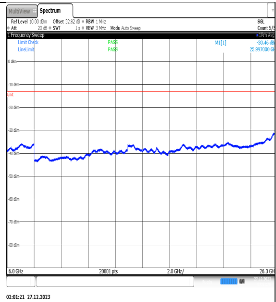
NTNV_N77-3450- 3550_PC2_30_30_L_TID12_NS_01_6000_26000 _#1
