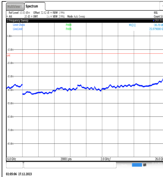
NTNV_N77-3450- 3550_PC2_30_30_L_TID13_NS_01_6000_26000 _#1
