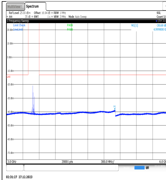
NTNV_N77-3450- 3550_PC2_30_30_M_TID5_NS_01_3000_6000_# 1
