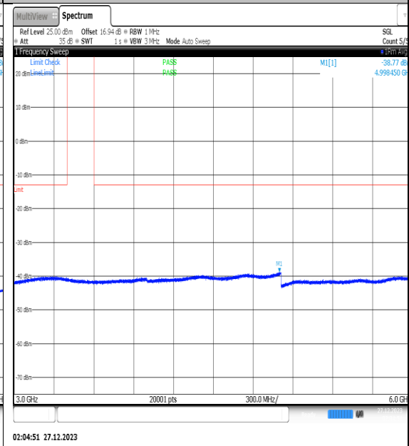
NTNV_N77-3450-3550_PC2_30_30_L_TID13_NS_01_3000_6000_#1
