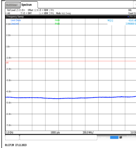
NTNV_N77-3450- 3550_PC2_30_30_L_TID5_NS_01_1000_3000_#1
