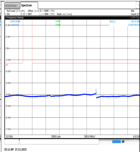
NTNV_N77-3450- 3550_PC2_30_30_L_TID15_NS_01_3000_6000_ #1
