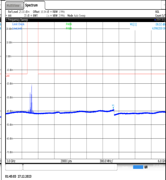
NTNV_N77-3450- 3550_PC2_30_30_L_TID9_NS_01_3000_6000_#
