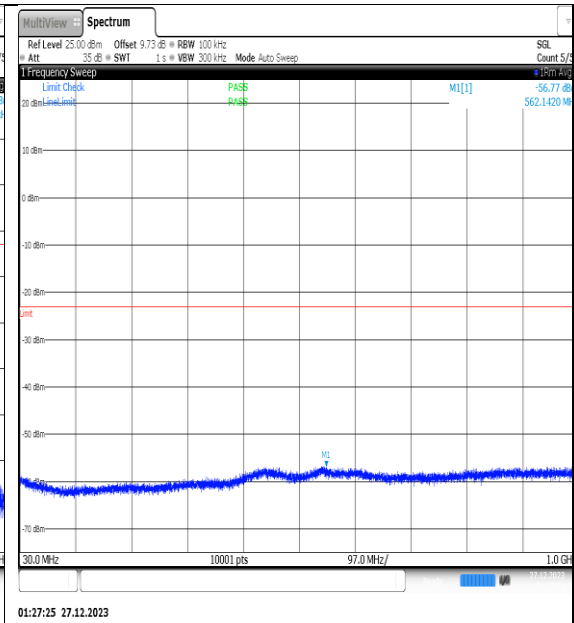
NTNV_N77-3450- 3550_PC2_30_30_L_TID5_NS_01_30_1000_#1
