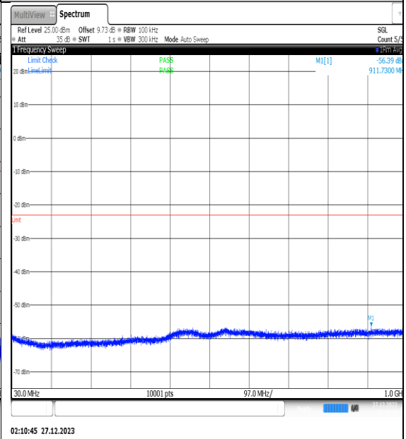
NTNV_N77-3450- 3550_PC2_30_30_L_TID15_NS_01_30_1000_#1
