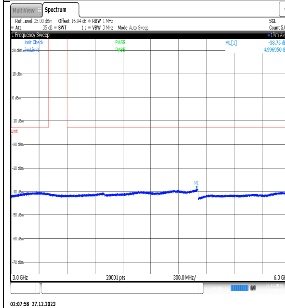
NTNV_N77-3450- 3550_PC2_30_30_L_TID14_NS_01_3000_6000_#1
