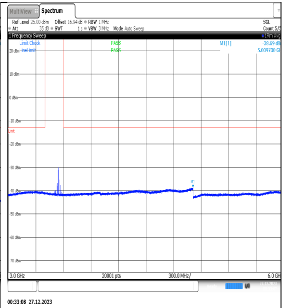
NTNV_N77-3450- 3550_PC2_30_25_H_TID6_NS_01_3000_6000_# 1
