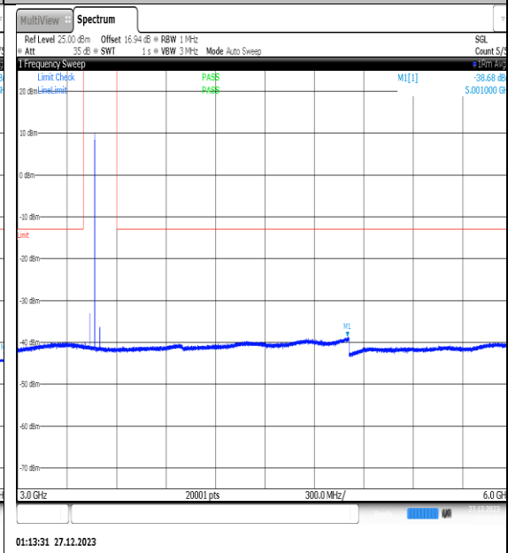
NTNV_N77-3450- 3550_PC2_30_30_L_TID1_NS_01_3000_6000_# 1
