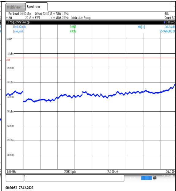
NTN_V_N77-3450- 3550_PC2_30_25_H_TID7_NS_01_6000_26000_# #1
