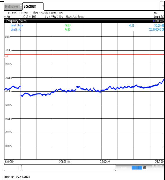
NTNV_N77-3450- 3550_PC2_30_25_H_TID3_NS_01_6000_26000_# 1
