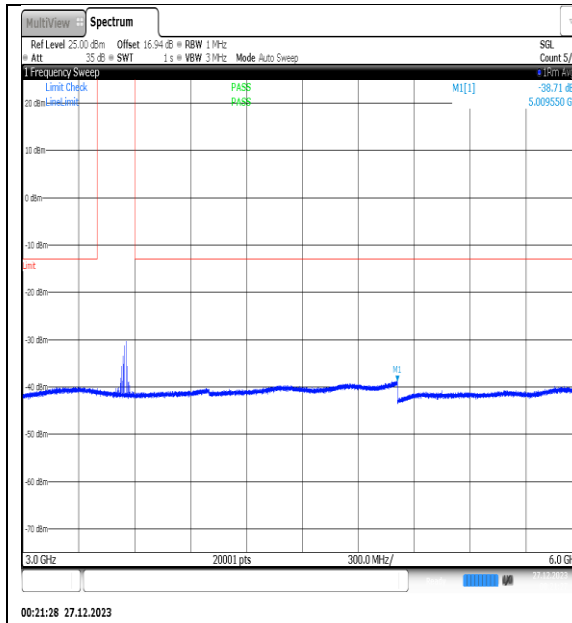
NTNV_N77-3450- 3550_PC2_30_25_H_TID3_NS_01_3000_6000_# 1
