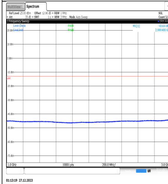
NTNV_N77-3450- 3550_PC2_30_30_L_TID1_NS_01_1000_3000_# 1
