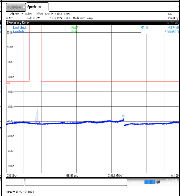
NTNV_N77-3450- 3550_PC2_30_25_H_TID8_NS_01_3000_6000_#
