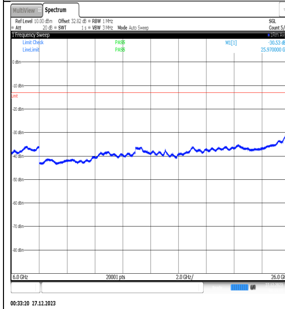
NTNV_N77-3450- 3550_PC2_30_25_H_TID6_NS_01_6000_26000_# 1
