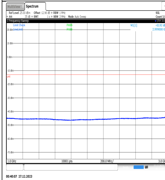
NTNV_N77-3450- 3550_PC2_30_25_H_TID8_NS_01_1000_3000_#
