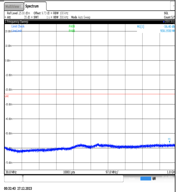
NTNV_N77-3450- 3550_PC2_30_25_H_TID6_NS_01_30_1000_#1
