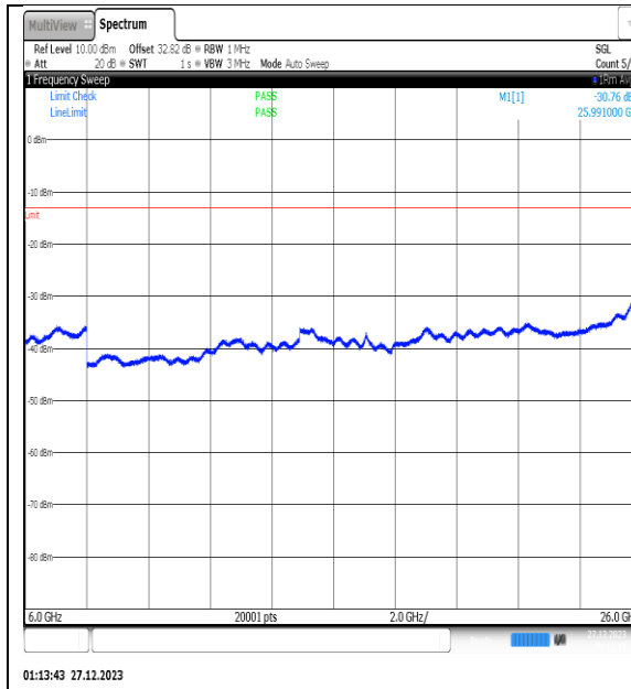
NTNV_N77-3450- 3550_PC2_30_30_L_TID1_NS_01_6000_26000_ #1
