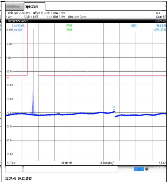
NTNV_N77-3450- 3550_PC2_30_25_M_TID9_NS_01_3000_6000_# 1
