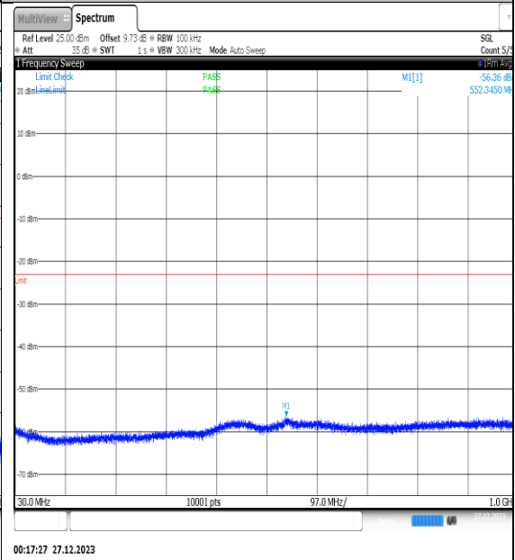
NTNV_N77-3450- 3550_PC2_30_25_H_TID2_NS_01_30_1000_#1
