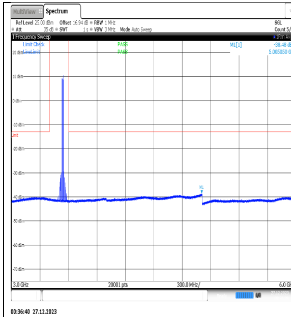
NTN_V_N77-3450- 3550_PC2_30_25_H_TID7_NS_01_3000_6000_# 1
