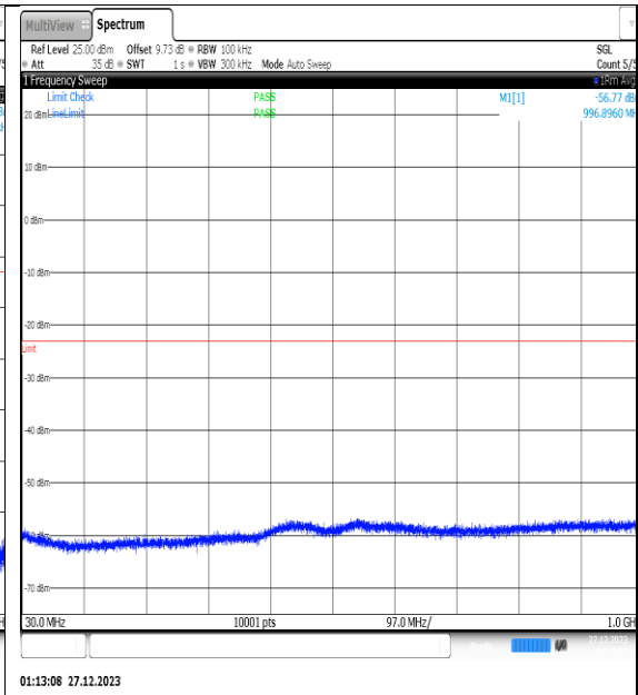
NTNV_N77-3450- 3550_PC2_30_30_L_TID1_NS_01_30_1000_#1
