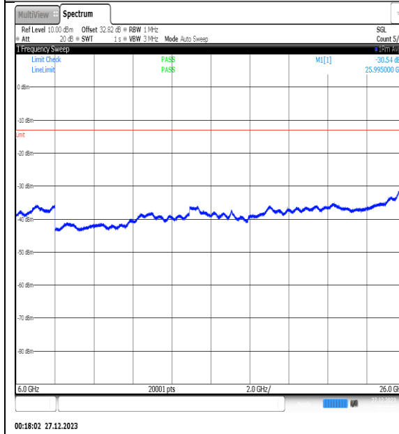
NTNV_N77-3450- 3550_PC2_30_25_H_TID2_NS_01_6000_26000_# 1
