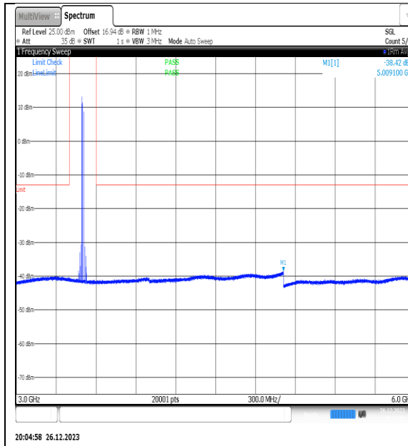
NTN_V_N77-3450- 3550_PC2_30_20_M_TID7_NS_01_3000_6000_# 1
