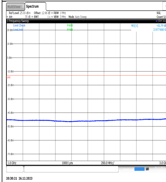
NTNV_N77-3450-3550_PC2_30_20_M_TID12_NS_01_1000_3000_#1
