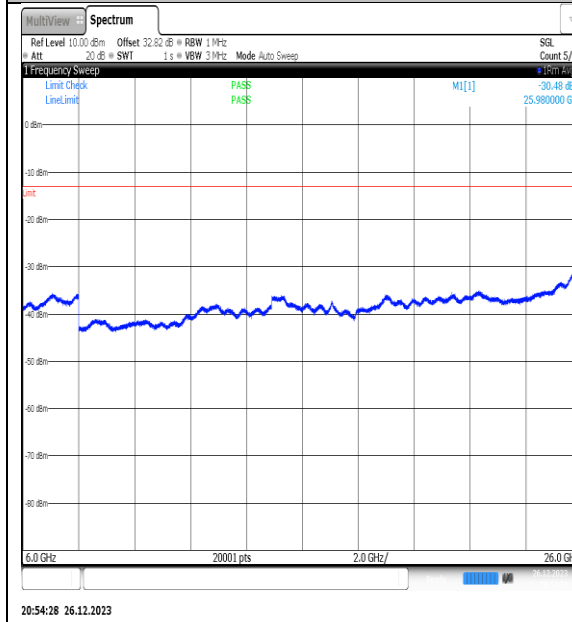
NTNV_N77-3450- 3550_PC2_30_20_H_TID3_NS_01_6000_26000_# 1
