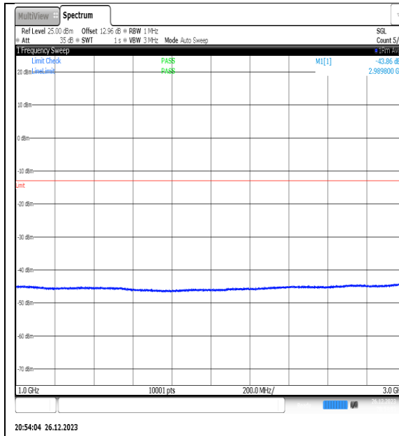
NTNV_N77-3450- 3550_PC2_30_20_H_TID3_NS_01_1000_3000_# 1
