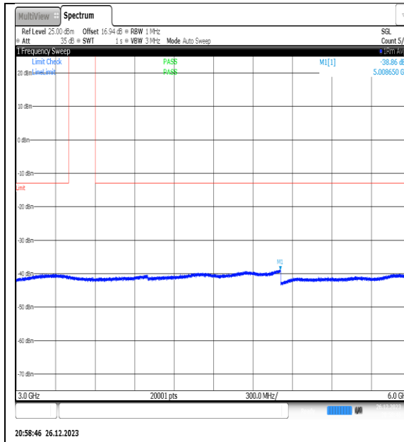
NTNV_N77-3450- 3550_PC2_30_20_H_TID4_NS_01_3000_6000_# 1
