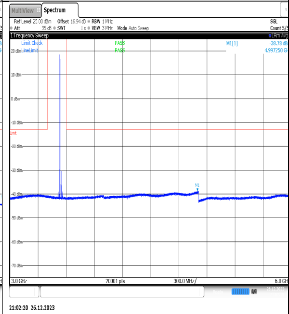
NTNV_N77-3450- 3550_PC2_30_20_H_TID5_NS_01_3000_6000_#
