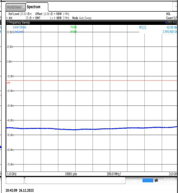
NTN V _N77-3450- 3550_PC2_30_20_M_TID15_NS_01_1000_3000_ #1
