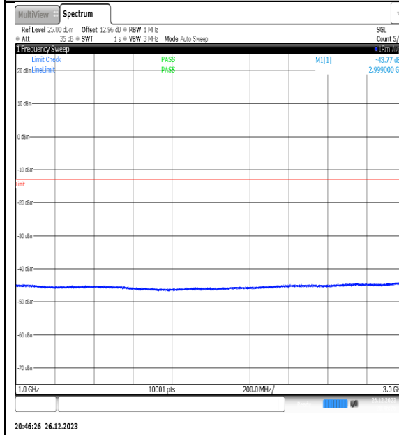
NTNV_N77-3450- 3550_PC2_30_20_H_TID1_NS_01_1000_3000_#
