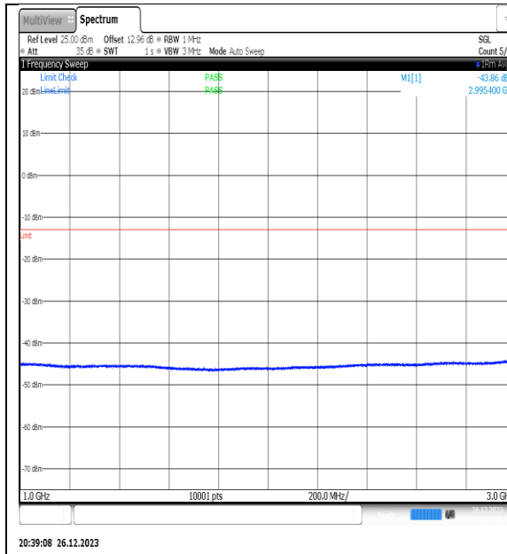
NTN_V_N77-3450- 3550_PC2_30_20_M_TID14_NS_01_1000_3000_ #1
