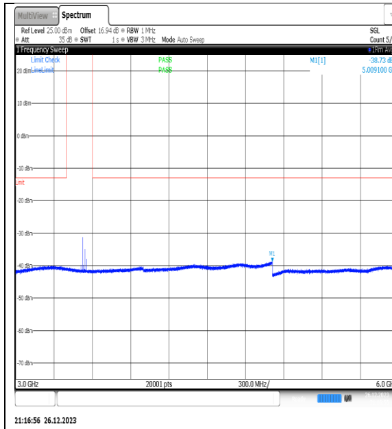
NTNV_N77-3450- 3550_PC2_30_20_H_TID8_NS_01_3000_6000_# 1
