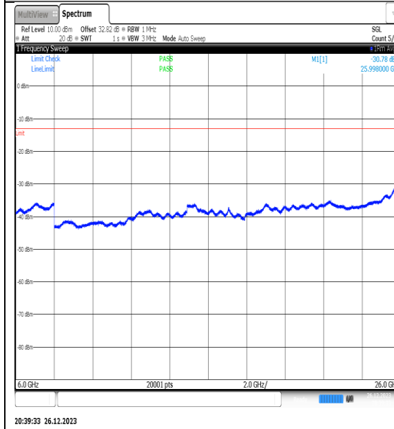
NTN_V_N77-3450- 3550_PC2_30_20_M_TID14_NS_01_6000_26000_ #1
