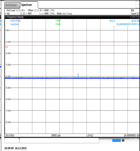
NTN_V_N77-3450- 3550_PC2_30_20_M_TID14_NS_01_26000_4000 0_#1
