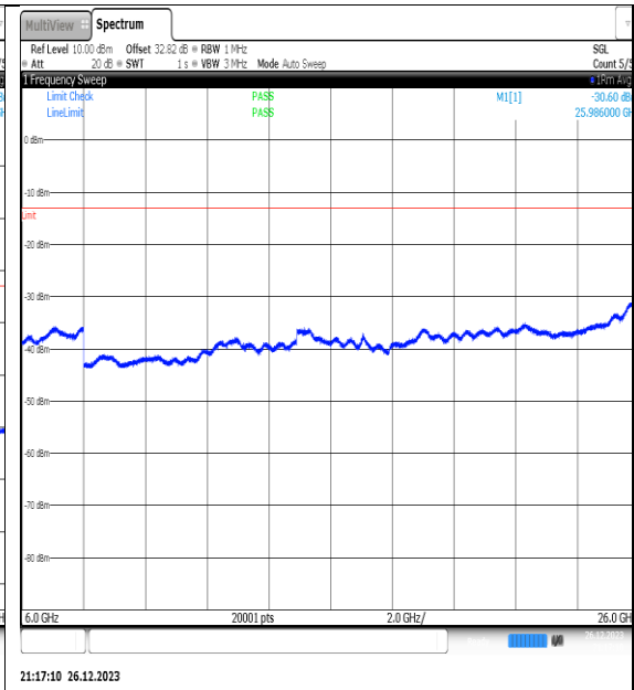
NTNV_N77-3450- 3550_PC2_30_20_H_TID8_NS_01_6000_26000_# #1
