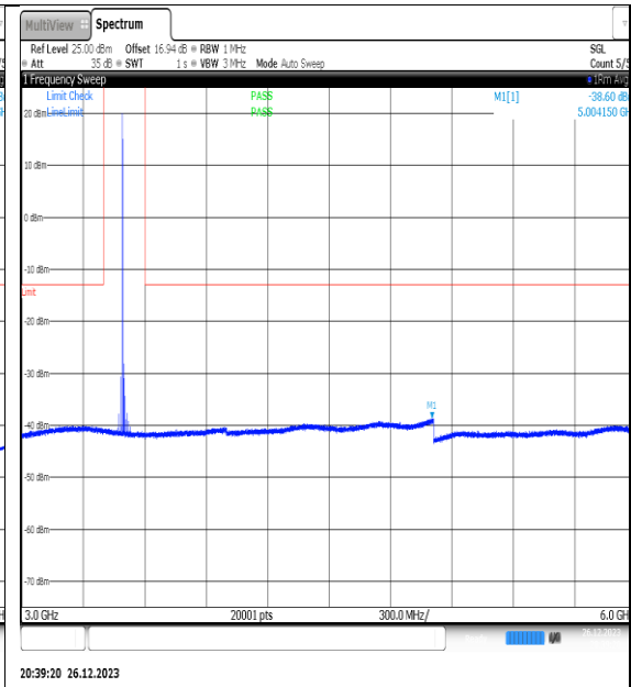
NTN_V_N77-3450- 3550_PC2_30_20_M_TID14_NS_01_3000_6000_ #1
