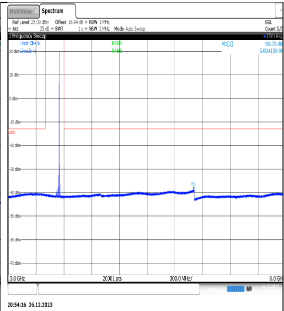
NTNV_N77-3450- 3550_PC2_30_20_H_TID3_NS_01_3000_6000_# 1
