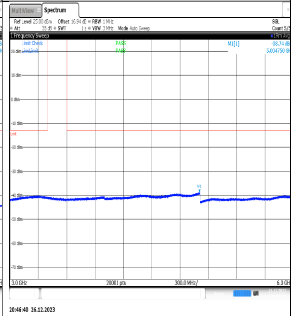
NTNV_N77-3450- 3550_PC2_30_20_H_TID1_NS_01_3000_6000_#
