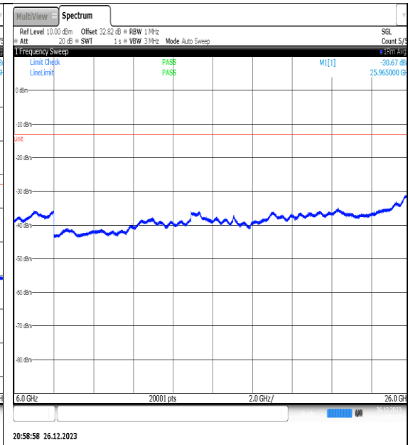
NTNV_N77-3450- 3550_PC2_30_20_H_TID4_NS_01_6000_26000_# #1
