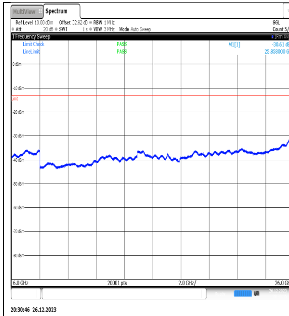
NTNV_N77-3450- 3550_PC2_30_20_M_TID12_NS_01_6000_26000 _#1
