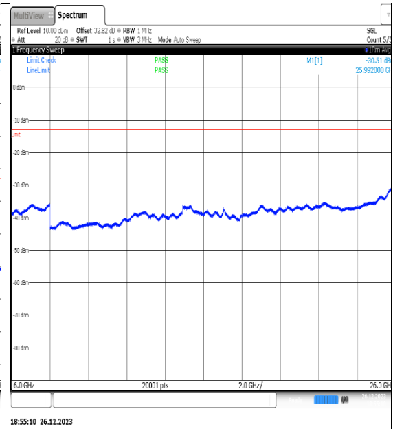
NTNV_N77-3450- 3550_PC2_30_20_L_TID6_NS_01_6000_26000_#1
