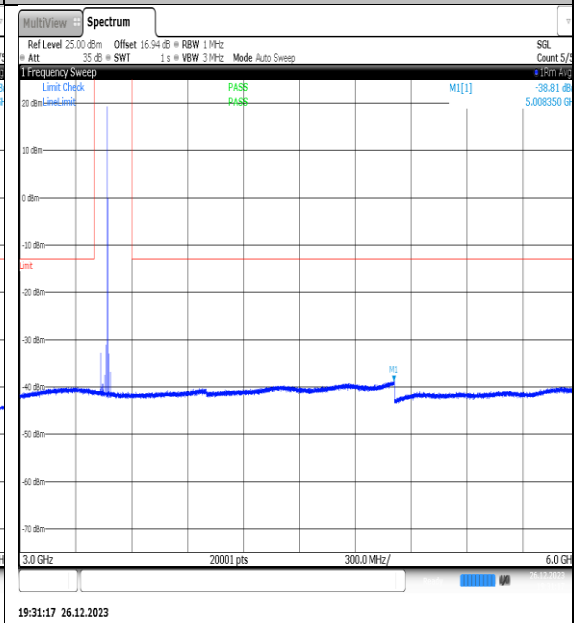
NTNV_N77-3450-3550_PC2_30_20_L_TID15_NS_01_3000_6000_#1
