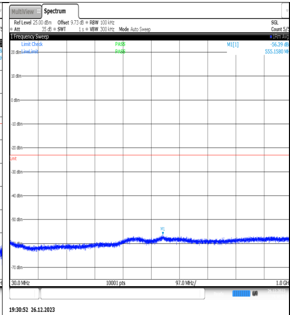
NTNV_N77-3450-3550_PC2_30_20_L_TID15_NS_01_30_1000_#1
