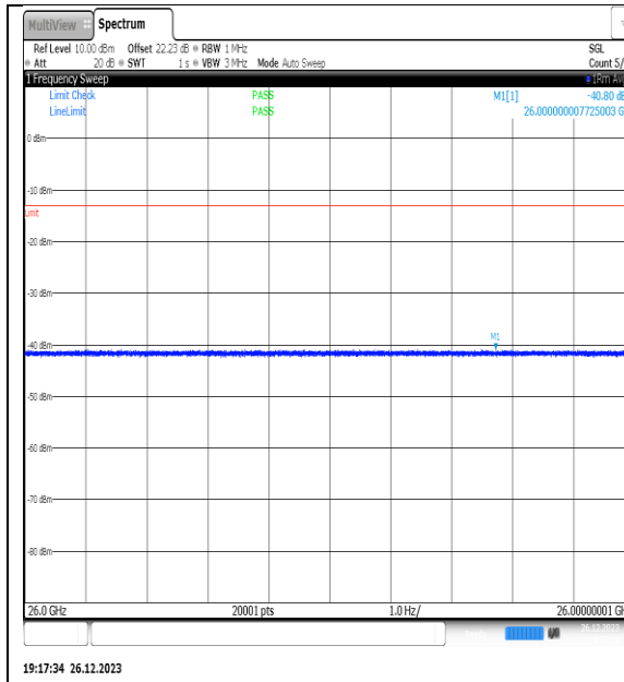
NTNV_N77-3450- 3550_PC2_30_20_L_TID12_NS_01_26000_4000 0_#1
