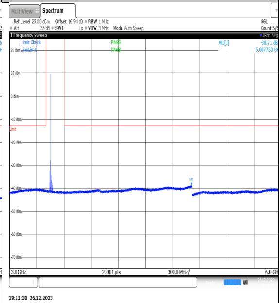
NTNV_N77-3450- 3550_PC2_30_20_L_TID11_NS_01_3000_6000_#1
