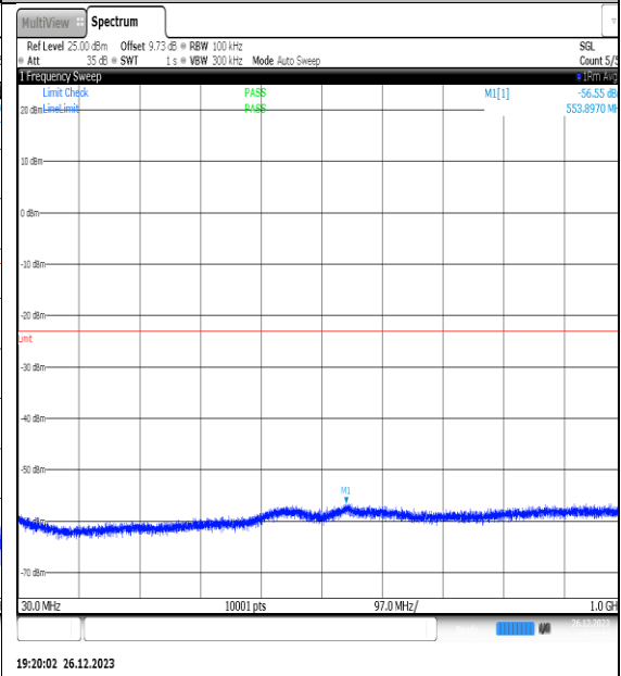
NTNV_N77-3450- 3550_PC2_30_20_L_TID13_NS_01_30_1000_#1
