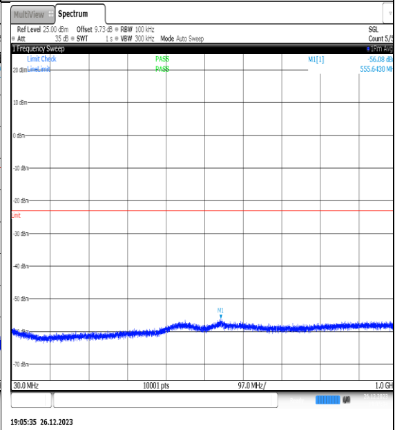
NTNV_N77-3450- 3550_PC2_30_20_L_TID9_NS_01_30_1000_#1
