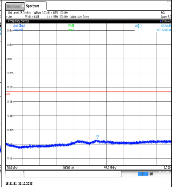
NTNV_N77-3450- 3550_PC2_30_20_L_TID5_NS_01_30_1000_#1
