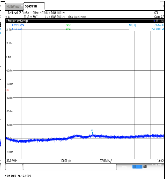
NTNV_N77-3450- 3550_PC2_30_20_L_TID11_NS_01_30_1000_#1
