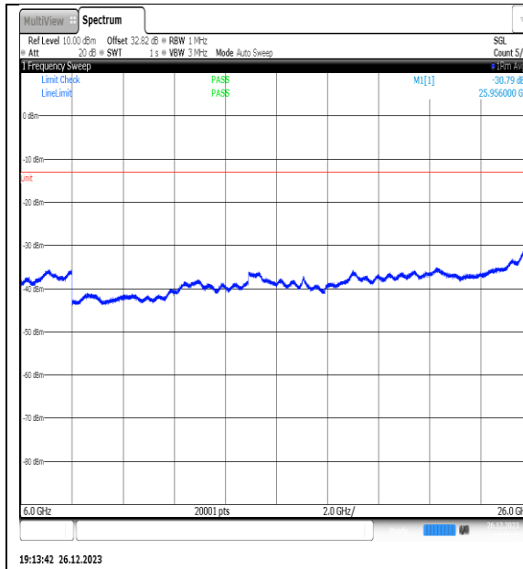
NTNV_N77-3450- 3550_PC2_30_20_L_TID11_NS_01_6000_26000 #1
