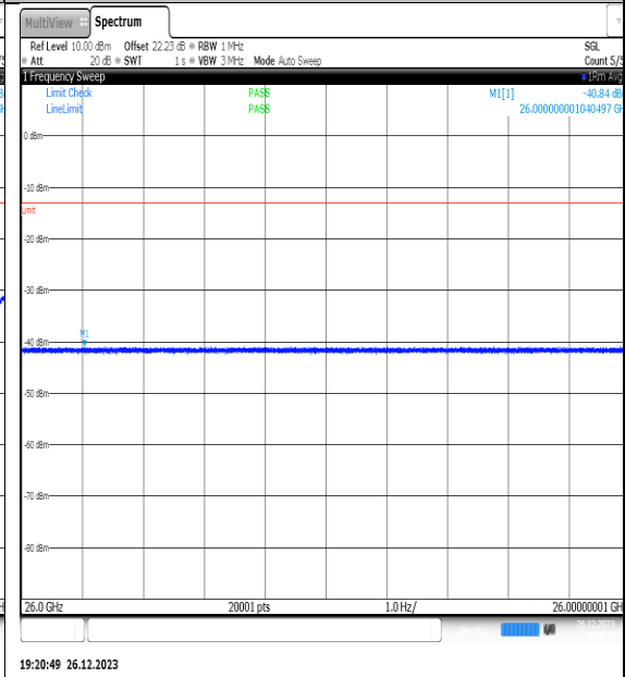
NTNV_N77-3450- 3550_PC2_30_20_L_TID13_NS_01_26000_4000_0_ #1
