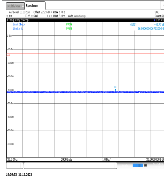
NTNV_N77-3450- 3550_PC2_30_20_L_TID10_NS_01_26000_4000_ 0_#1
