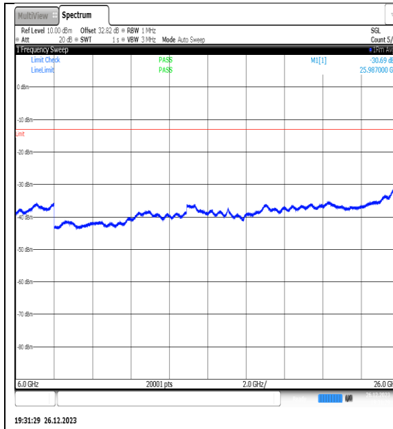
NTNV_N77-3450- 3550_PC2_30_20_L_TID15_NS_01_6000_26000 _#1
