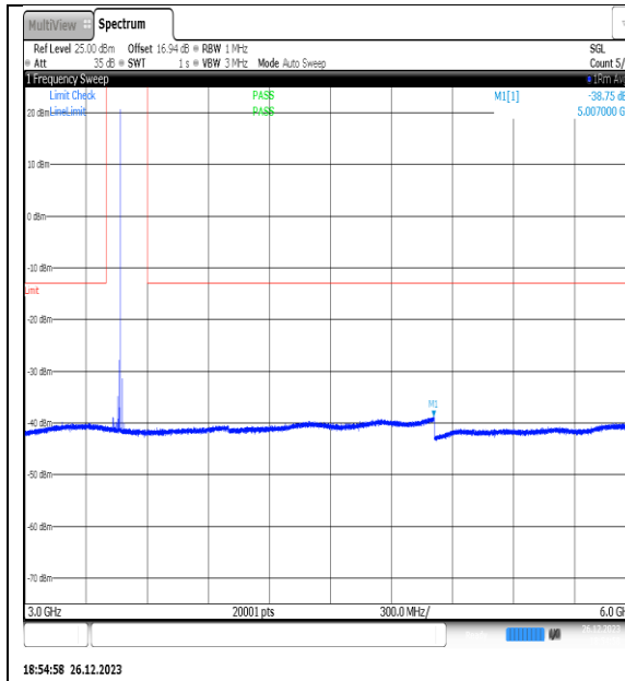
NTNV_N77-3450- 3550_PC2_30_20_L_TID6_NS_01_3000_6000_# 1
