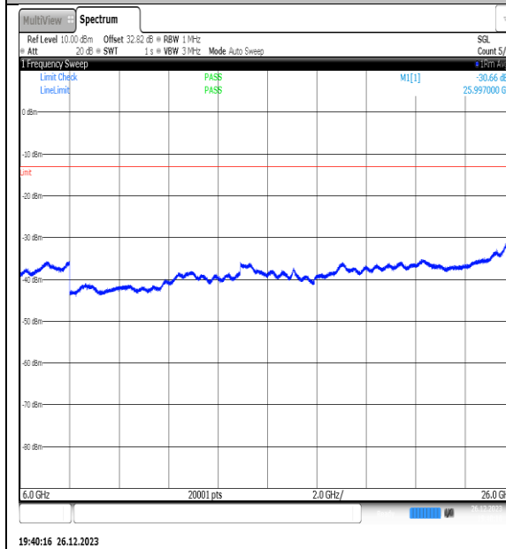
NTNV_N77-3450- 3550_PC2_30_20_M_TID2_NS_01_6000_26000_# 1
