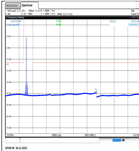
NTNV_N77-3450- 3550_PC2_30_20_L_TID10_NS_01_3000_6000_ #1
