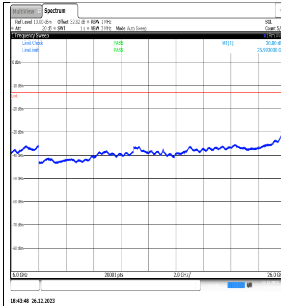
NTNV_N77-3450- 3550_PC2_30_20_L_TID3_NS_01_6000_26000_ #1
