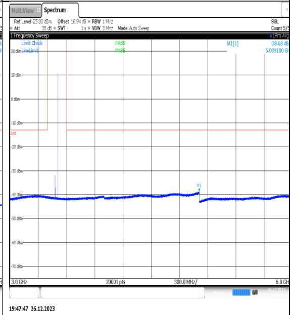
NTNV_N77-3450- 3550_PC2_30_20_M_TID4_NS_01_3000_6000_# 1
