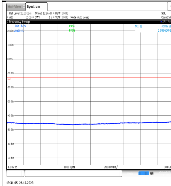
NTNV_N77-3450-3550_PC2_30_20_L_TID15_NS_01_1000_3000_#1
