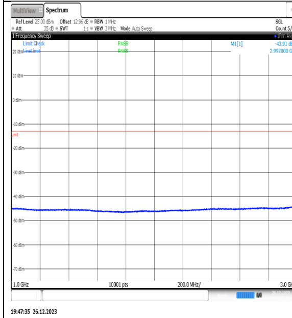
NTNV_N77-3450- 3550_PC2_30_20_M_TID4_NS_01_1000_3000_# 1
