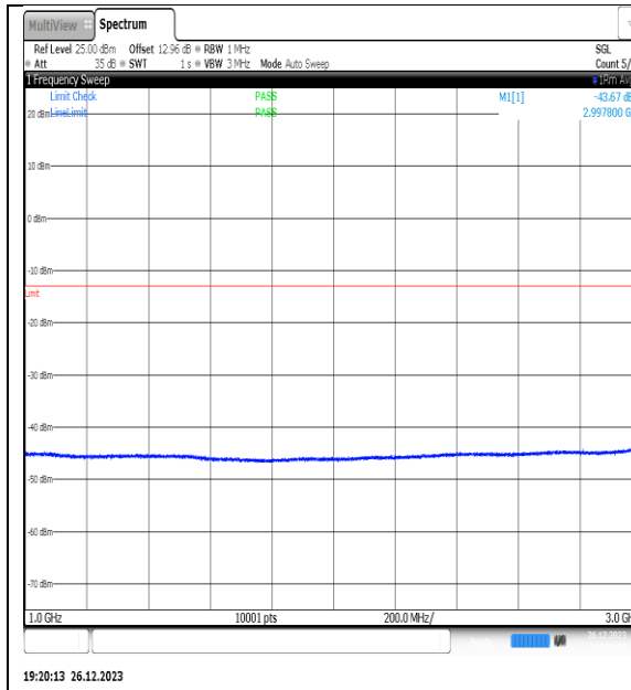
NTNV_N77-3450- 3550_PC2_30_20_L_TID13_NS_01_1000_3000_ #1
