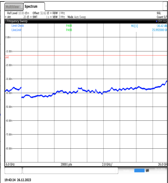
NTNV_N77-3450- 3550_PC2_30_20_M_TID3_NS_01_6000_26000_# 1
