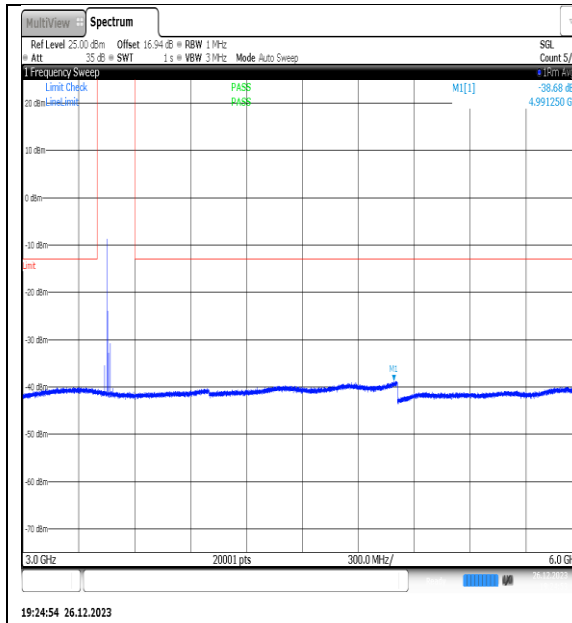
NTNV_N77-3450- 3550_PC2_30_20_L_TID14_NS_01_3000_6000_ #1
