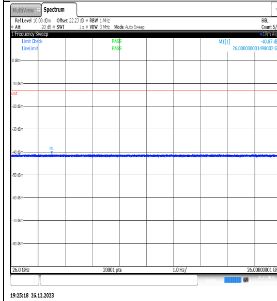
NTNV_N77-3450- 3550_PC2_30_20_L_TID14_NS_01_26000_4000_ 0_#1
