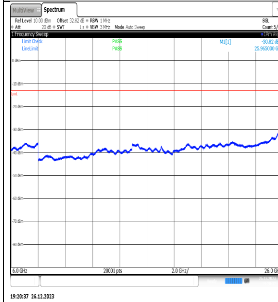
NTNV_N77-3450- 3550_PC2_30_20_L_TID13_NS_01_6000_26000_ #1
