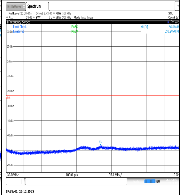
NTNV_N77-3450- 3550_PC2_30_20_M_TID2_NS_01_30_1000_#1
