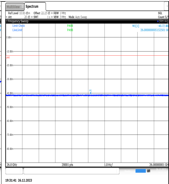
NTNV_N77-3450- 3550_PC2_30_20_L_TID15_NS_01_26000_4000 0_#1
