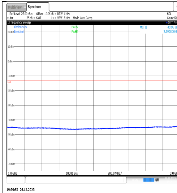
NTNV_N77-3450- 3550_PC2_30_20_M_TID2_NS_01_1000_3000_# 1
