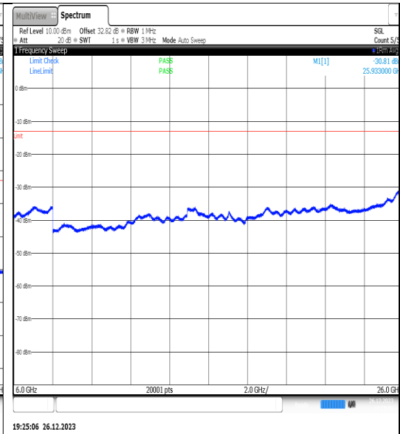
NTNV_N77-3450- 3550_PC2_30_20_L_TID14_NS_01_6000_26000_ #1
