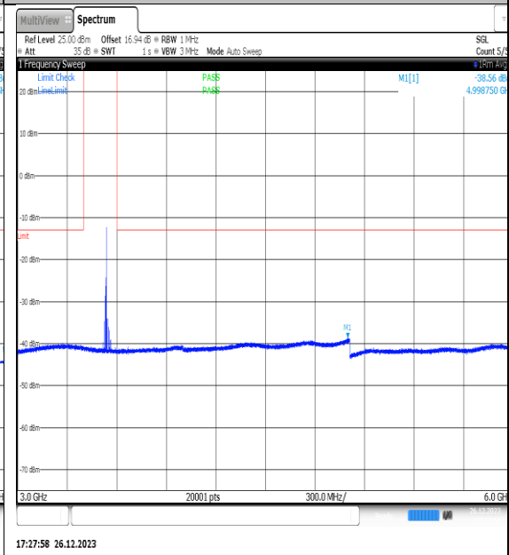
NTNV_N77-3450- 3550_PC2_30_15_H_TID2_NS_01_3000_6000_# 1
