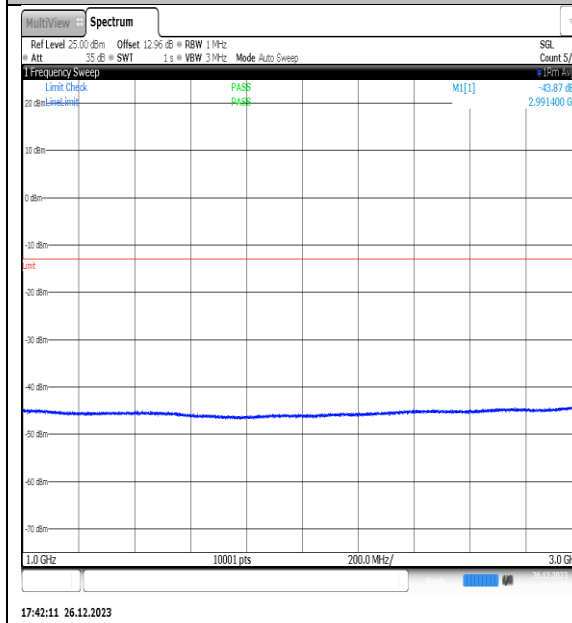
NTNV_N77-3450- 3550_PC2_30_15_H_TID6_NS_01_1000_3000_# 1
