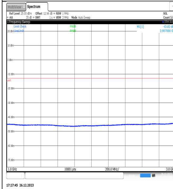
NTNV_N77-3450- 3550_PC2_30_15_H_TID2_NS_01_1000_3000_# 1
