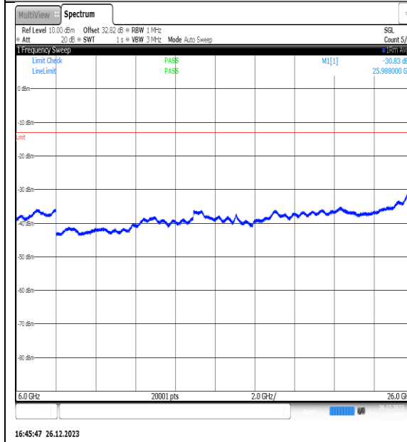
NTN_V_N77-3450- 3550_PC2_30_15_M_TID7_NS_01_6000_26000_# #1
