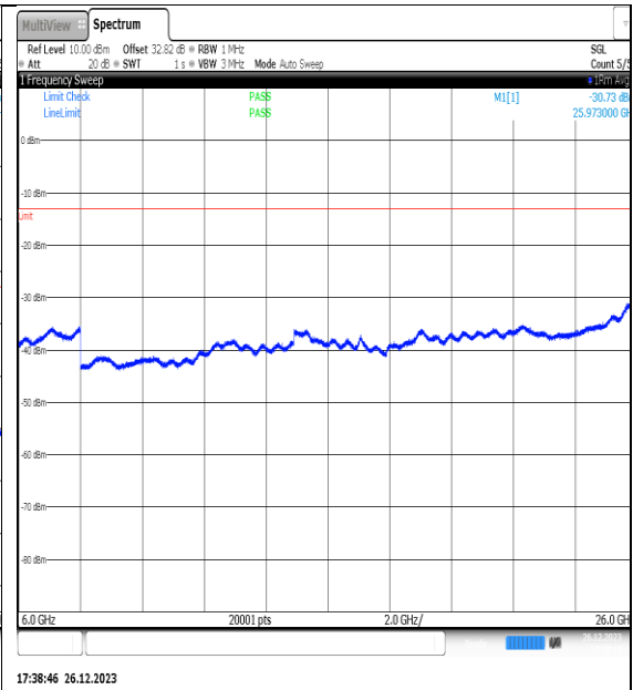
NTNV_N77-3450- 3550_PC2_30_15_H_TID5_NS_01_6000_26000_# 1
