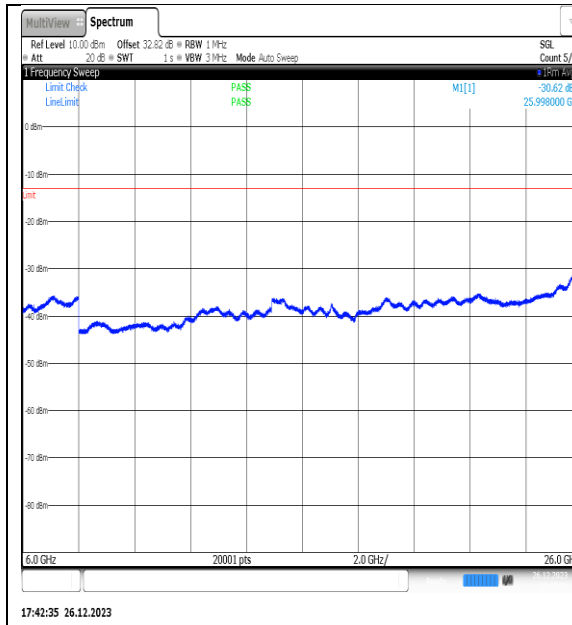
NTNV_N77-3450- 3550_PC2_30_15_H_TID6_NS_01_6000_26000_#1
