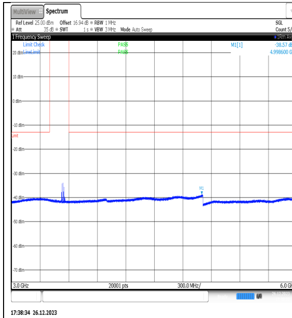
NTNV_N77-3450- 3550_PC2_30_15_H_TID5_NS_01_3000_6000_# 1
