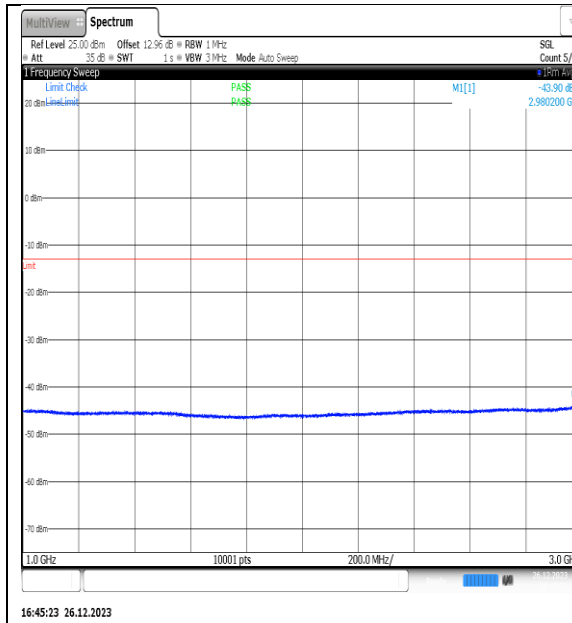
NTN_V_N77-3450- 3550_PC2_30_15_M_TID7_NS_01_1000_3000_# 1
