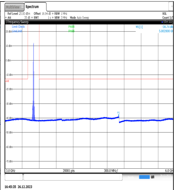
NTN_V_N77-3450- 3550_PC2_30_15_M_TID7_NS_01_3000_6000_# 1
