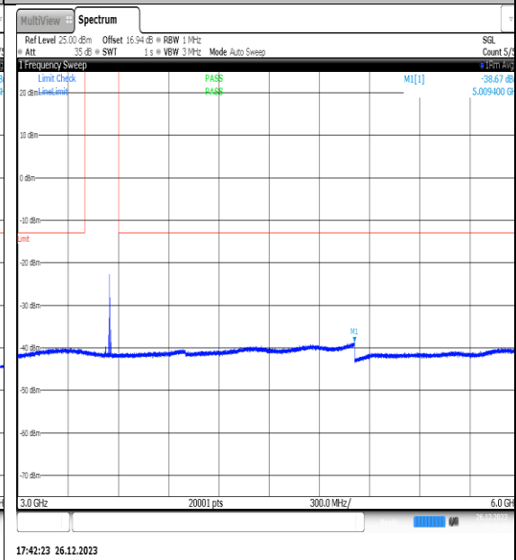
NTNV_N77-3450- 3550_PC2_30_15_H_TID6_NS_01_3000_6000_# 1
